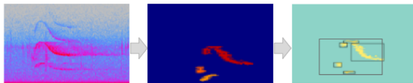
FIG. 3.8 – Principales étapes de l'extraction des événements acoustiques : Binarisation et détection des composants connectés. Le spectrogramme montre des fréquences de 0 à 6,5 kHz pendant 2,5 sec.
