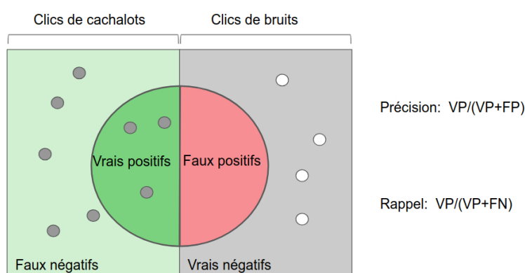
FIG. 5.10 – Résumé des notions de précision et de rappel dans le cadre d'une détection de clics de Cachalots. Les transitoires détectés par notre modèle sont à l'intérieur du cercle (vrais positifs + faux positifs).
