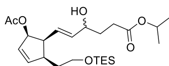
cis-167 : dr 1.7:1
