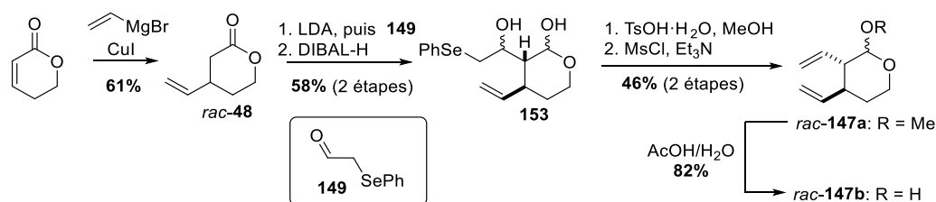
Schéma 7. Synthèse du lactol rac -147b par difonctionnalisation vicinale.
