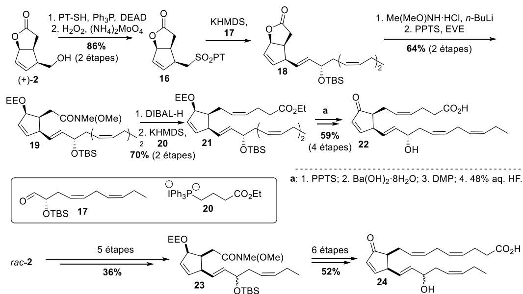
Schéma 3. L'approche de Zanoni/Porta et al. concernant les NeuroPs à base de cyclopenténone.
