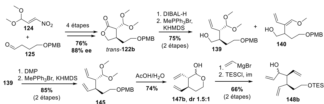
Schéma 6. Synthèse du précurseur 148b protégé orthogonalement à partir de la lactone trans - 122b .
