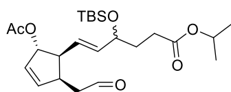
trans - 169 : dr 2.5:1
