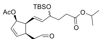
cis -169: dr 2.5:1
