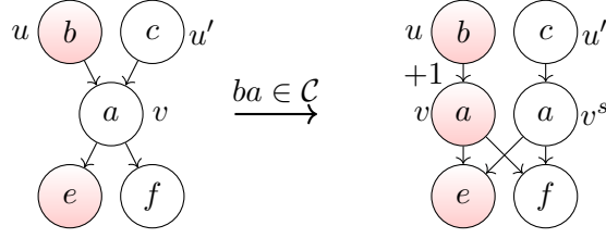
FIGURE 3.6 – Scission : en tant que prédécesseur du sommet étiqueté par b , v doit être activé, mais puisqu’il est aussi prédécesseur du sommet étiqueté par c , il ne doit pas l’être non plus. Un nouveau sommet v^s étiqueté par a est ainsi créé.
