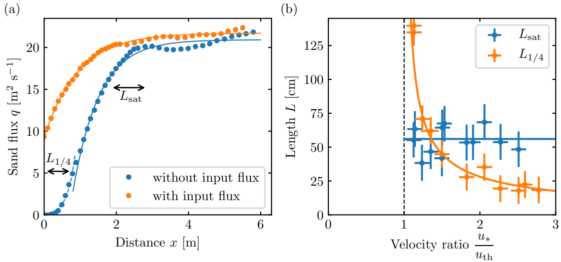
FIGURE 1.8 – (a) Flux le long d’un lit plat de sédiments avec (orange) et sans (bleu) flux en entrée, pour d = 120 \mu\text{m} et u_*/u_{th} \simeq 1.5 . Le lit commence en x = 0 , précédé d’une zone non-érodable. Courbes en traits pleins : relaxation exponentielle proche de l’état saturé. Courbe pointillée : croissance exponentielle initiale. (b) Variation des deux longueurs caractéristiques en fonction de la distance au seuil de transport. Données provenant de Andreotti et al. (2010). Figure adaptée de Durán et al. (2011)
