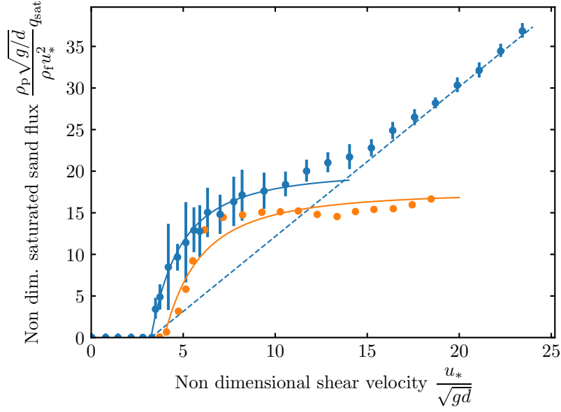
FIGURE 1.7 – Flux saturé en fonction de la vitesse de cisaillement provenant de mesures en soufflerie par Iversen & Rasmussen (1999) (orange) et de simulations numériques par Durán et al. (2011) (bleu). Le flux est normalisé par u_*^2 afin de montrer les comportements asymptotiques. Les courbes en traits pleins correspondent au comportement en u_*^2 - u_{\text{th}}^2 , et celle en pointillés à celui en u_* u_*^2 - u_{\text{th}}^2 . Figure adaptée de Durán et al. (2011)
