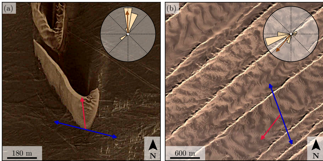
FIGURE 1.22 – (a) Barkhane asymétrique au sud de la Skeleton Coast, Namibie ( 20^{\circ}21''\text{S} , 13^{\circ}19''\text{E} ). (b) Dunes râtaux au nord du désert du Kumtagh, Chine ( 40^{\circ}10''\text{N} , 92^{\circ}11''\text{E} ). Les distributions angulaires des flux de sable sont calculées à partir des données de vents à 10 m du modèle de réanalyse climatique Era5 (Hersbach et al. 2020), en supposant une taille de grain de 180\ \mu\text{m} et une rugosité aérodynamique de 1 mm. Les orientations prédites par l'équation (1.46) pour le mécanisme d'élongation (rouge) et par l'équation (1.45) pour l'instabilité de lit (bleu) en utilisant ces distributions correspondent aux crêtes visibles sur l'image satellite (images satellites : Google TM , CNES/Airbus, TerraMetrics, Maxar Technologies).
