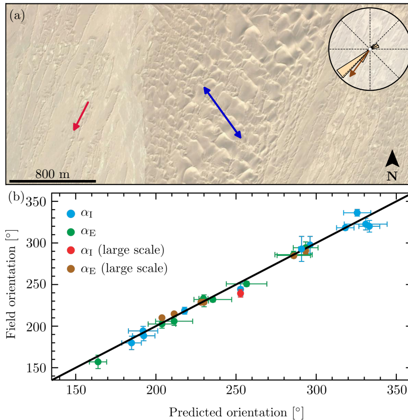
FIGURE 1.21 – (a) Coexistence de deux orientations distinctes dans le désert du Taklamacan en Chine ( 38.3^\circ\text{N} , 86.7^\circ\text{E} ). Les orientations prédites par l'équation (1.46) pour le mécanisme d'élongation (rouge) et par l'équation (1.45) pour l'instabilité de lit (bleu) correspondent aux crêtes visibles sur l'image satellite (image satellite : Google TM , Maxar technologies). En haut à droite, la distribution angulaire des flux de sable sur lit plat est calculée à partir des données de vents à 10 m du modèle de réanalyse climatique Era5 (Hersbach et al. 2020), en supposant une taille de grain de 180\ \mu\text{m} et une rugosité aérodynamique de 1 mm. La flèche marron donne la direction du flux résultant correspondant. (b) Comparaison des orientations prédites par le modèle de Courrech du Pont et al. (2014) avec des mesures effectuées sur des images satellites de 11 régions dans les déserts du Sahara, Rub'Al Khali, Taklamacan et Mu Us. Les orientations sont mesurées dans le sens trigonométrique par rapport à l'est, à petite ( \sim 30\ \text{m} ) et grande ( \sim 1\ \text{km} ) échelles. Figure adaptée de Courrech du Pont et al. (2014).
