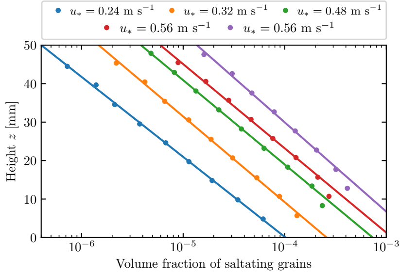
FIGURE 1.6 – Mesure en soufflerie de profils verticaux de fraction volumique de grains en saltation, pour différentes valeurs de vitesse de cisaillement (Creysse et al. 2009).
