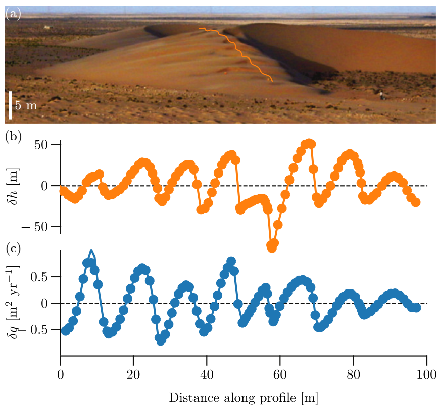
FIGURE 1.9 – (a) Oscillation de sable sur la crête d'une dune. La ligne orange correspond au profil des mesures de topographie (b) et de flux (c). La modulation du flux \delta q est calculée via le taux d'érosion en utilisant la conservation de la masse. Figure modifiée de Elbelrhiti et al. (2005).
