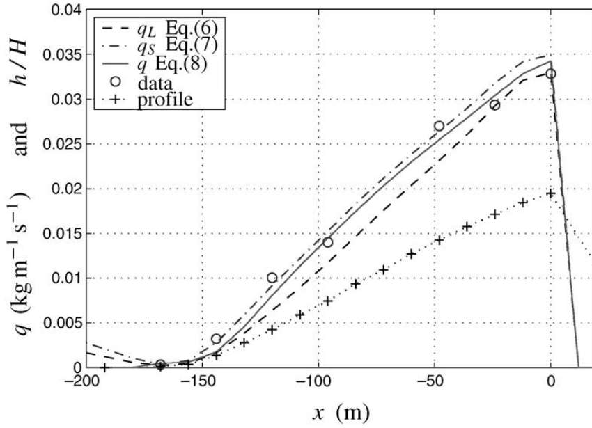
FIGURE 1.16 – Flux le long de la section centrale d’une barkhane. Les prédictions théoriques sont faites à partir de mesures de vitesse du vent en utilisant les formules de flux saturé de Lettau & Lettau (1978) ( q_L ) et Sørensen (1991) ( q_S ). La ligne pleine q prend en compte la relaxation spatiale du flux, avec la longueur de saturation. Figure provenant de Sauermann et al. (2003).
