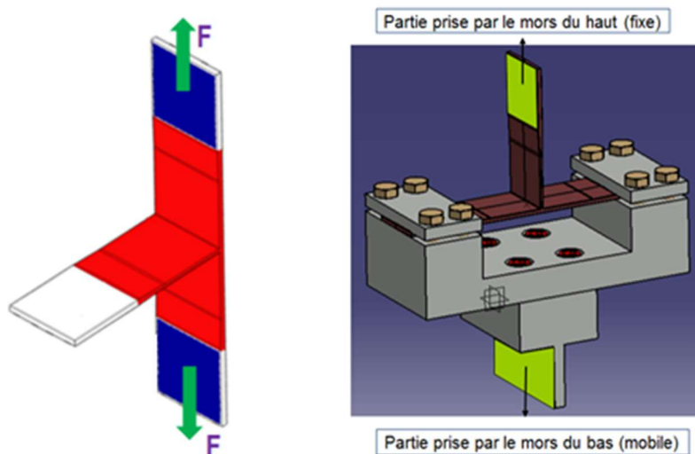
Figure 1-18 : Schématisation des conditions appliquées en traction (à gauche) et en flexion (à droite) aux éprouvettes T-Bone pour une étude de la réponse en fatigue multiaxiale d'un PA66GF50 [Serr15]
