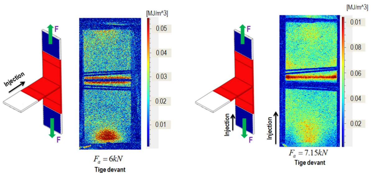
Figure 1-25 : Lieu de rupture en fonction du point d'injection sur des éprouvettes T-Bone en PA66GF50 soumises à un chargement de fatigue en traction ( R=0 et f=1Hz ) à T23RH50 [Serr15]
