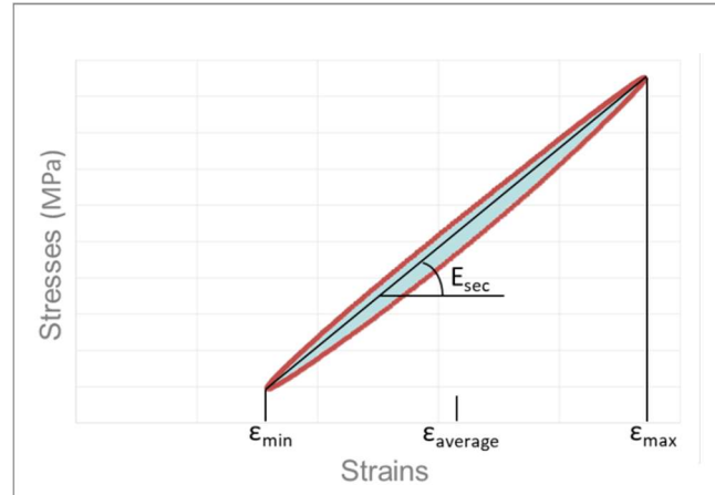
Figure 3-6 : Représentation des critères de comparaison
