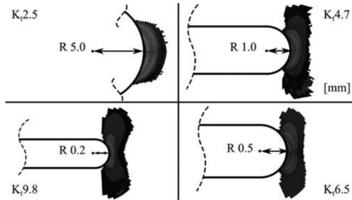
Figure 1-47 : Evolution de la taille et de la forme du volume d'intérêt autour d'un trou de différentes tailles [Scha15]
