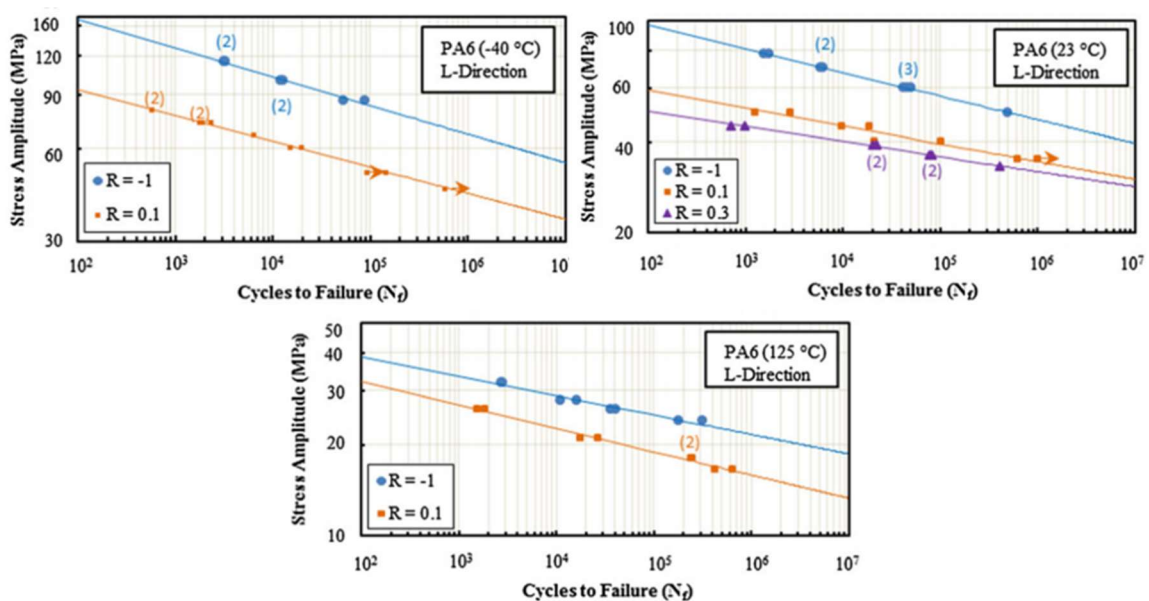
Figure 1-20 : Courbes de Wöhler (amplitude de contrainte en fonction de la durée de vie) pour un chargement uniaxial de traction dans la direction des fibres à différentes températures et différents rapports de charge sur du PA6GF35 DAM [Mort16]
