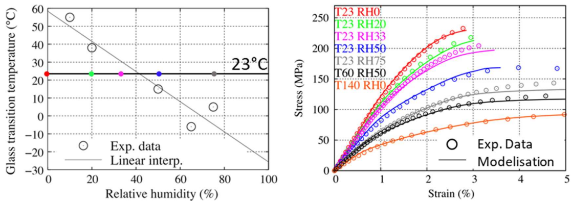
Figure 1-15 : Validation du modèle proposé par Launay sur des essais de traction monotone d'un PA66GF35 pour différents conditionnements [Laun13a]. Les différents conditionnements sont situés par rapport à leur transition vitreuse estimée sur la figure de gauche.
