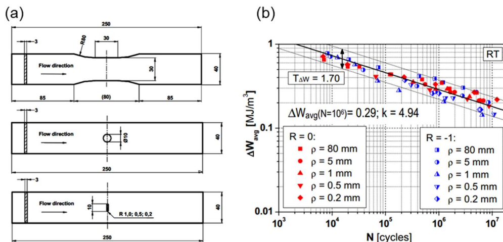
Figure 1-45 : (a) Eprouvettes présentant trous de différents diamètres \rho ; (b) Comparaison des résultats en fatigue pour des éprouvettes de PA66GF35 percées par des trous de différents diamètres \rho et soumises à un chargement uniaxial pour deux rapports de charge différents à l'ambiante [Demo07]
