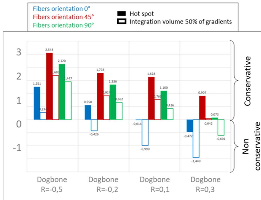
Figure 4-20 : Ecart (en décades) entre durées de vie expérimentales et durées de vie prédites avec le volume d'intégration ou avec la méthode « point chaud » pour les éprouvettes Dogbone. Les frontières du volume d'intégration sont fixées à 50% du gradient maximal de FIP. Les écarts mentionnés sont moyennés sur tous les niveaux de chargement de la courbe S-N correspondant au couple (R, orientation) considéré
