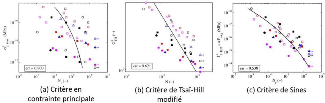
Figure 1-31 : Comparaison des résultats avec un critère (a) en contrainte principale, (b) de Tsai-Hill modifié et (c) de Sines pour différents chargements sur du PA66GF35 à T23RH50 [Laun13c]. La base de données expérimentale est issue des travaux de Klimkeit ([Klim11a]) pour un PA66GF35 à T23RH50. Les FIP en entrée des trois critères sont calculés à partir du tenseur des contraintes macroscopique calculé sur le 20 ème cycle simulé. Seul un volume représentatif de la partie utile est simulé.
