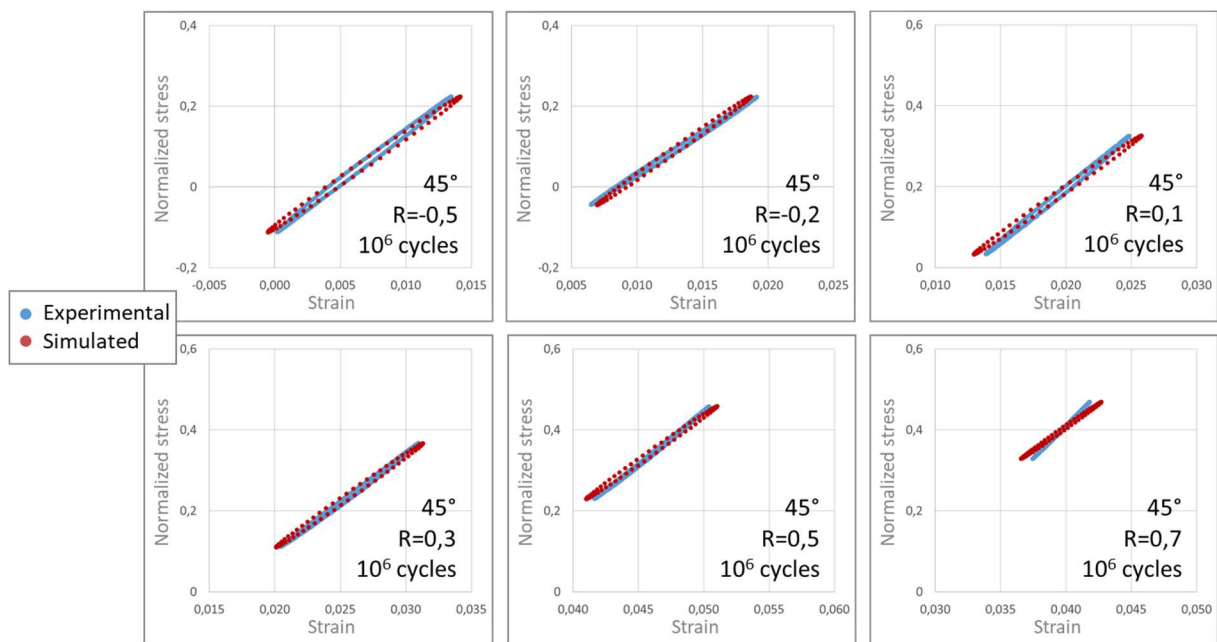
Figure A-7 : Boucles d'hystérèse calculées et expérimentales dans la direction de sollicitation pour des essais uniaxiaux menés sur éprouvettes Dogbone à 45° pour une durée de vie d'environ 10^6 cycles et pour différents rapports de charge
