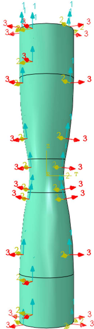
Figure B-2 : Représentation du repère matériau dans Abaqus sur toute la géométrie des éprouvettes tubulaires
