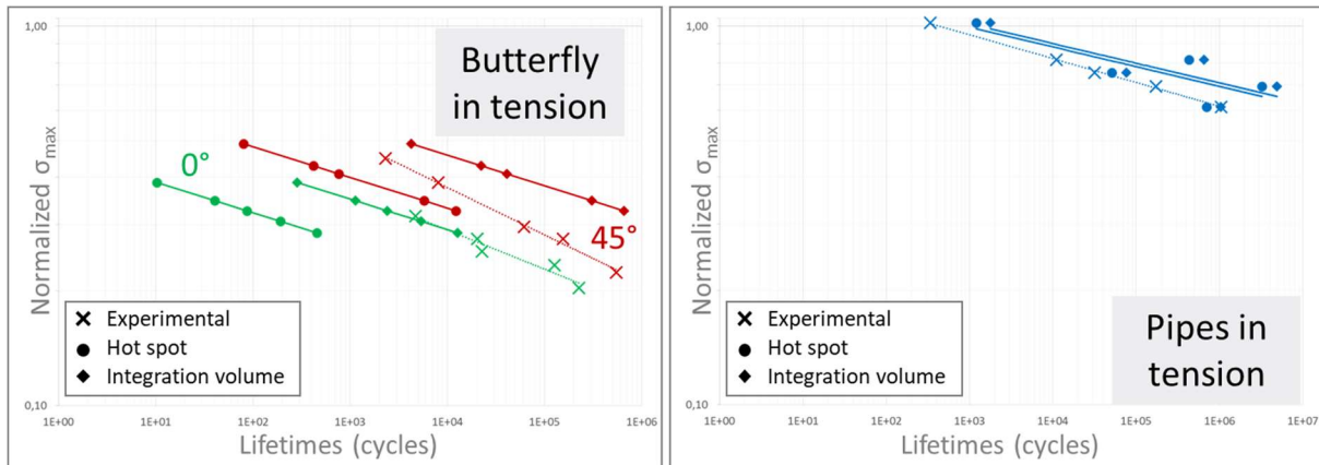
Figure 4-24 : Comparaison entre les courbes de Wöhler calculées avec le volume d'intégration ou avec la méthode « point chaud » et les courbes expérimentales pour les éprouvettes papillon à 0°, 45° et pour les éprouvettes tubulaires. Traction à R=0 . Les frontières du volume d'intégration sont fixées à 50% du gradient maximal de FIP.
