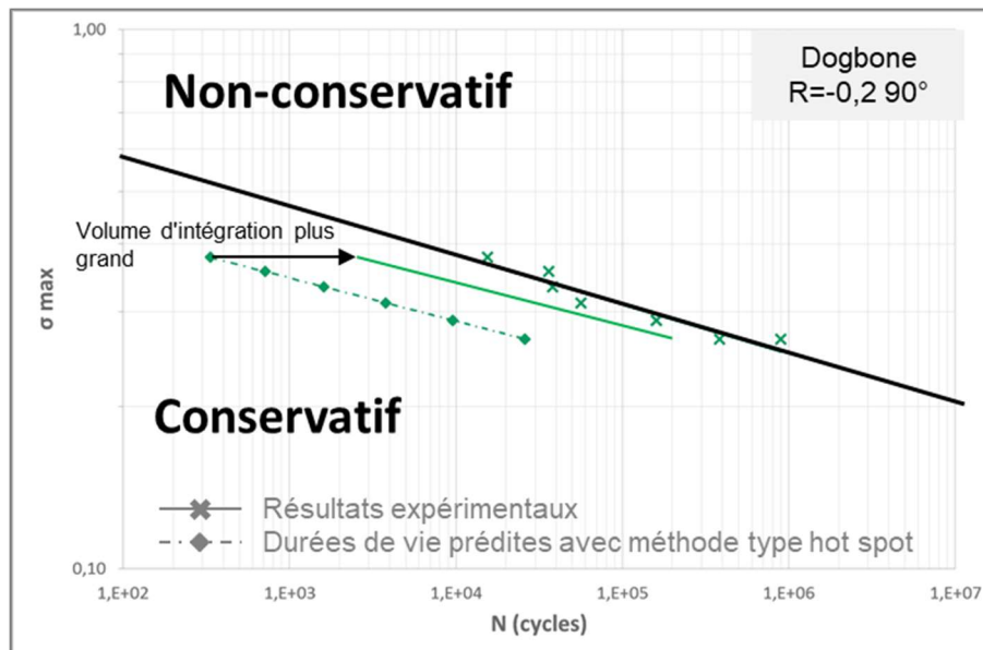
Figure 3-20 : Représentation du déplacement de la courbe S-N vers la droite lorsque la taille du volume d'intégration augmente
