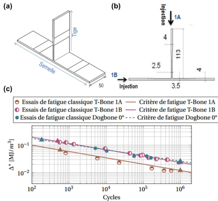
Figure 1-24 : (a) Géométrie des éprouvettes structurales T-Bone ; (b) Plan en coupe d'une T-Bone avec indication des deux seuils d'injection correspondant aux deux types d'éprouvettes envisagés ; (c) Courbes représentant l'énergie dissipée mesurée par thermographie infrarouge à l'avant de la semelle (côté tige) pour les deux types d'éprouvettes injectées en PA66GF50 à T23RH50 pour les essais de traction présentés figure 1-18 [Serr15]
