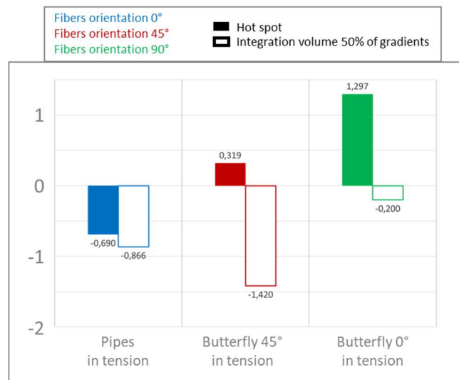
Figure 4-25 : Écarts (en décades) entre durées de vie expérimentales et durées de vie prédites avec le volume d'intégration ou avec la méthode « point chaud » pour les éprouvettes papillon à 0°, 45° et les tubes. Traction à R=0 . Les frontières du volume d'intégration sont fixées à 50% du gradient maximal de FIP. Les écarts mentionnés sont moyennés sur tous les niveaux de chargement de la courbe S-N considérée.
