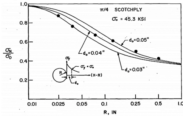
Figure 1-42 : Méthode "point stress criterion" : évolution du rapport entre contrainte à rupture en traction monotone des éprouvettes en composite laminées verre/époxy percées sur celle des éprouvettes lisses en fonction du rayon de perçage [Whit74]
