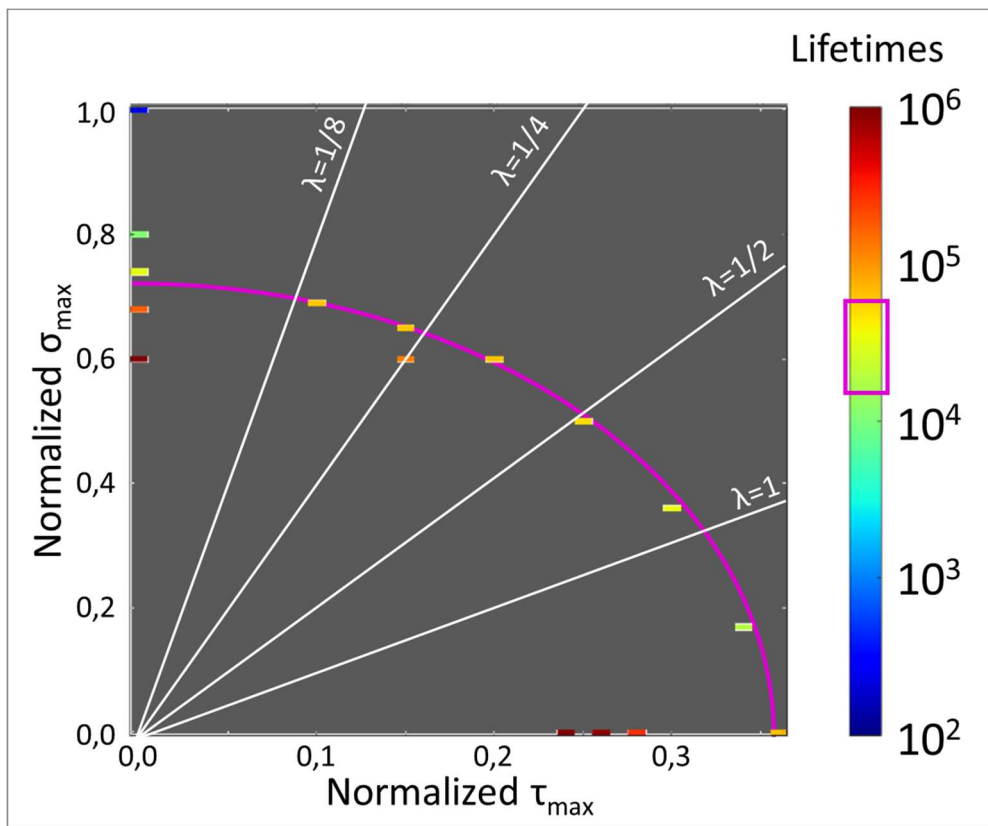
Figure 2-41 : Diagramme de durées de vie du PA66GF50 à T80RH50 pour les éprouvettes tubulaires en traction-torsion en phase à R=0
