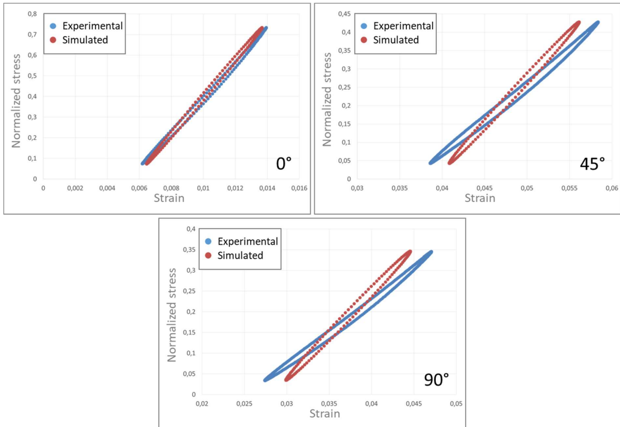
Figure 3-11 : Comparaison des boucles d'hystérèse macroscopiques expérimentale et numérique obtenue avec la loi viscoélastique identifiée pour la matrice en traction à R=0.1 pour des éprouvettes Dogbone orientées à (a) 0^\circ , (b) 45^\circ et (c) 90^\circ
