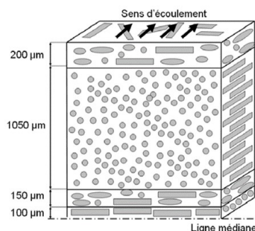
Figure 1-3 : Illustration de la microstructure cœur-peau dans la demi-épaisseur d'une plaque injectée [Klim11a]
