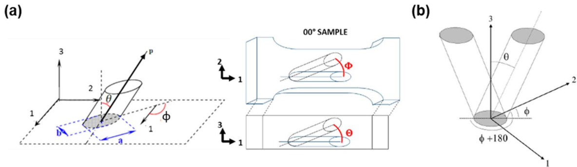
Figure 1-9 : (a) Représentation des angles \phi et \theta dans l'espace et vis-à-vis du plan de découpe [Sant18]; (b) Représentation de l'ambiguïté d'orientation [Eber01]
