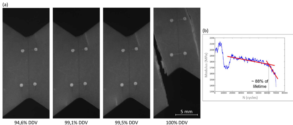
Figure 2-29 : (a) Photographies prises au cours de l'essai Iosipescu sur une éprouvette à 0^\circ et (b) évolution du module sécant de cette même éprouvette au cours de l'essai
