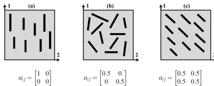
Figure 1-8 : Exemples de tenseurs d'orientation et schématisation de l'orientation des fibres associée pour des cas où (a) les fibres sont toutes orientées selon l'axe 1 ; (b) les fibres sont réparties de manière isotrope ; (c) les fibres sont alignées dans une direction à 45° de l'axe 1 ([Arif14b])
