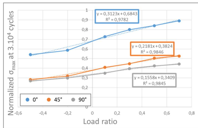
Figure 2-9 : Evolution de la contrainte maximale à 5.10^4 cycles en fonction du rapport de charge pour des essais de fatigue uniaxiaux sur éprouvettes Dogbone pour les orientations 0°, 45° et 90° à T80RH50
