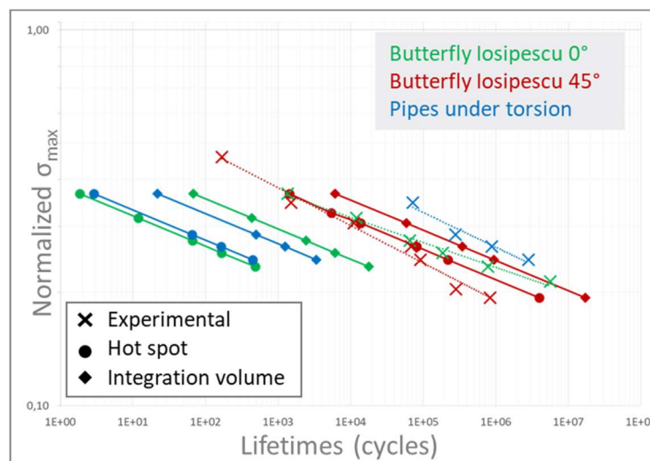
Figure 4-28 : Comparaison entre les courbes de Wöhler calculées avec le volume d'intégration ou avec la méthode « point chaud » et les courbes expérimentales pour les éprouvettes papillon à 0°, 45° sous essais Iosipescu et pour les éprouvettes tubulaires en torsion, R=0 . Les frontières du volume d'intégration sont fixées à 50% du gradient maximal de FIP.
