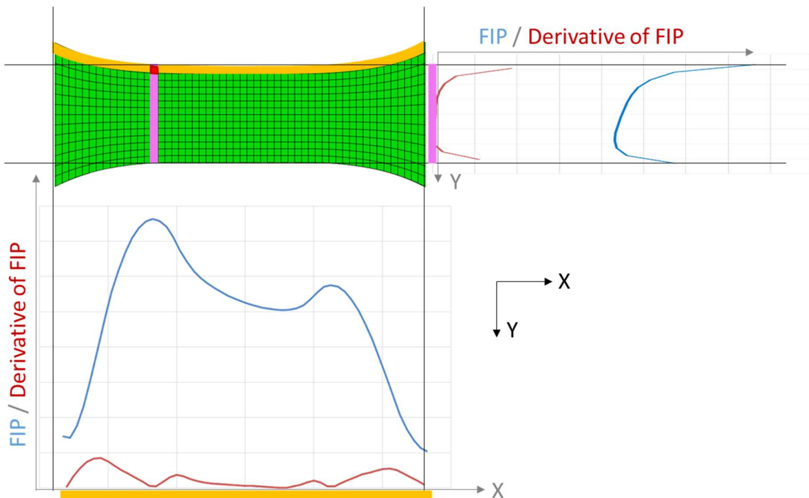
Figure 4-13 : Etape 3 de la définition du domaine d'intégration dans le plan : tracé de la dérivée spatiale du FIP moyen le long des chemins d'étude
