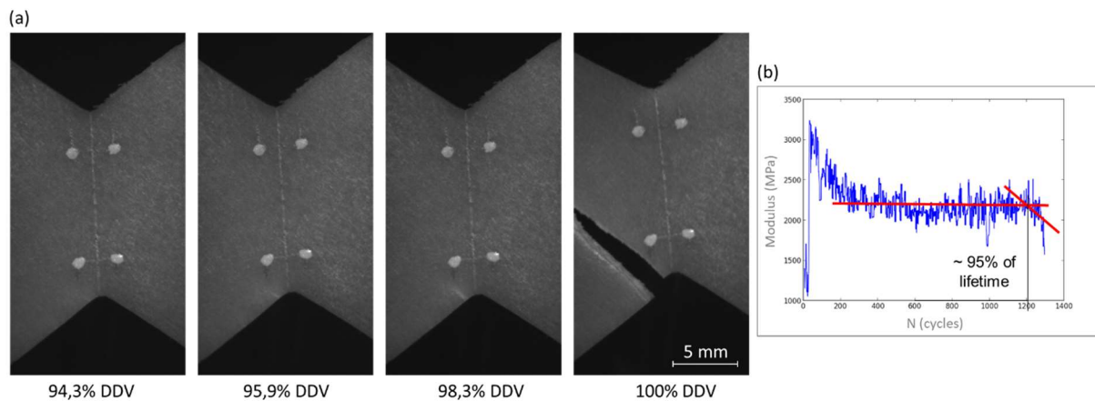
Figure 2-30 : (a) Photographies prises au cours de l'essai Iosipescu sur une éprouvette à 45^\circ et (b) évolution du module sécant de cette même éprouvette au cours de l'essai
