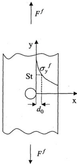
Figure 1-41 : Schéma de l'expérience et des axes [Zago01]
