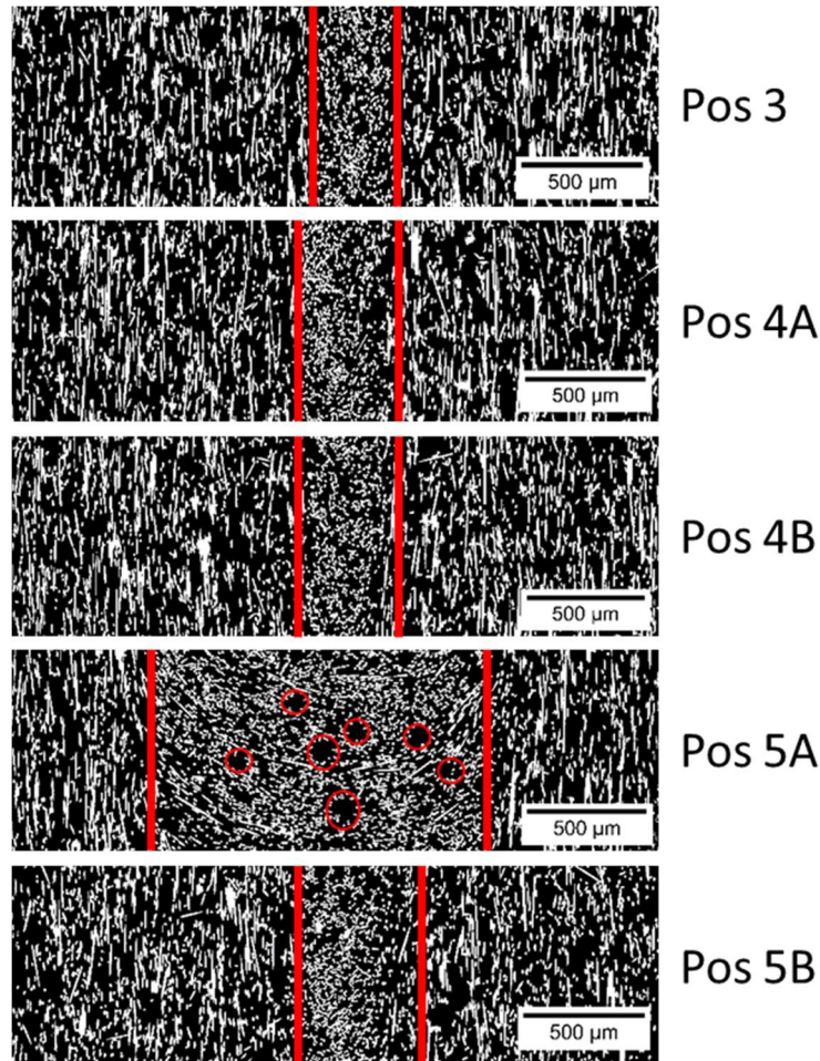
Figure 2-14 : Images en microscopie réalisées à l'ENSTA Bretagne sur des éprouvettes prélevées à différentes positions dans la plaque injectée. Les traits verticaux rouges représentent les frontières du cœur, les cercles rouges entourent des vides.
