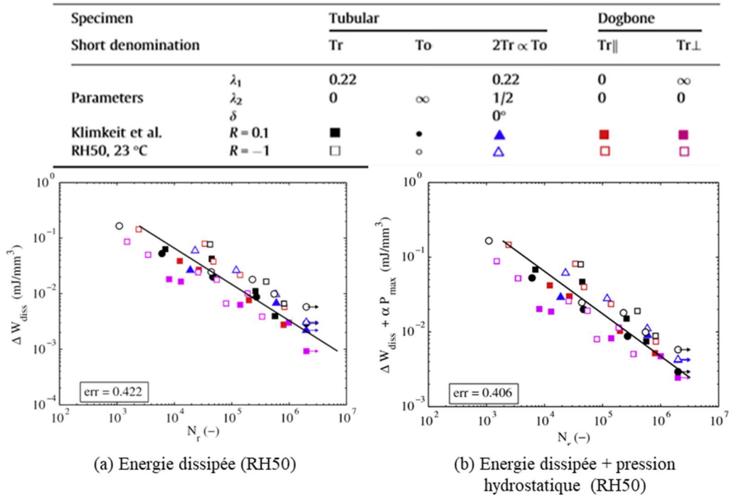
Figure 1-33 : Comparaison des résultats avec un critère en énergie dissipée et un critère en énergie dissipée combinée à la pression hydrostatique [Laun13c]. La base de données expérimentale est issue des travaux ([Klim11a]) pour un PA66GF35 à T23RH50. Les FIP en entrée des deux critères sont calculés à partir des tenseurs des contraintes et des déformations macroscopiques calculés sur le 20 ème cycle simulé. Seul un volume représentatif de la partie utile est simulé.
