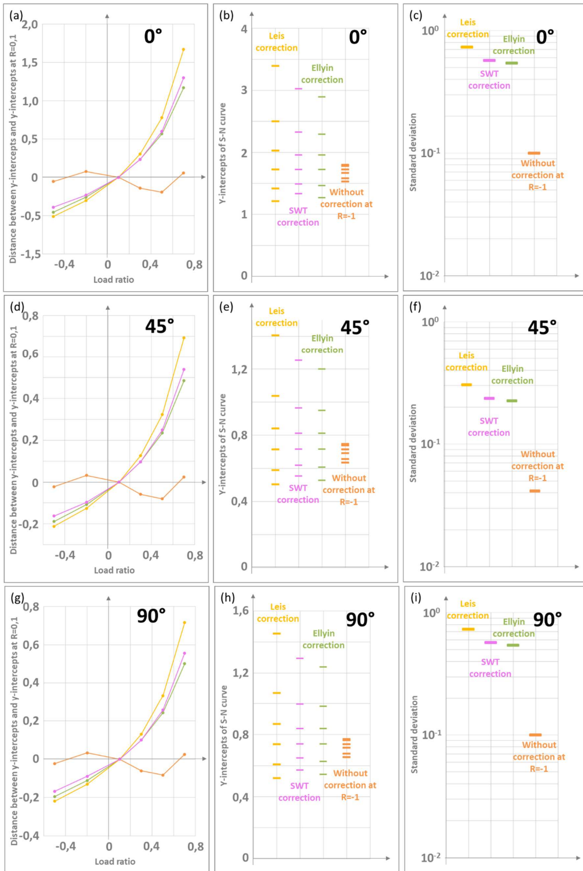
Figure 4-11 : (a, d, g) Ecart à l'ordonnée à l'origine de la courbe S-N brute à R=0,1 en fonction du rapport de charge pour les corrections de contrainte moyenne proposées dans la littérature, et pour chaque orientation; (b, e, h) Ordonnée à l'origine des courbes S-N normées pour les six rapports de charge, pour chacune des corrections et pour chaque orientation ; (c, f, i) Ecart-type des ordonnées à l'origine des courbes S-N sur l'ensemble des rapports de charge pour chacune des corrections et pour chaque orientation
