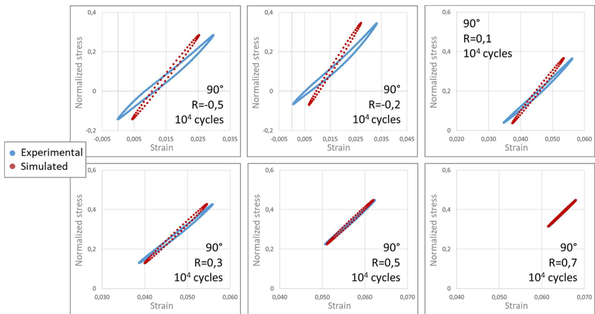
Figure A-3 : Boucles d'hystérèse calculées et expérimentales dans la direction de sollicitation pour des essais uniaxiaux menés sur éprouvettes Dogbone à 90° pour une durée de vie d'environ 10 4 cycles et pour différents rapports de charge
