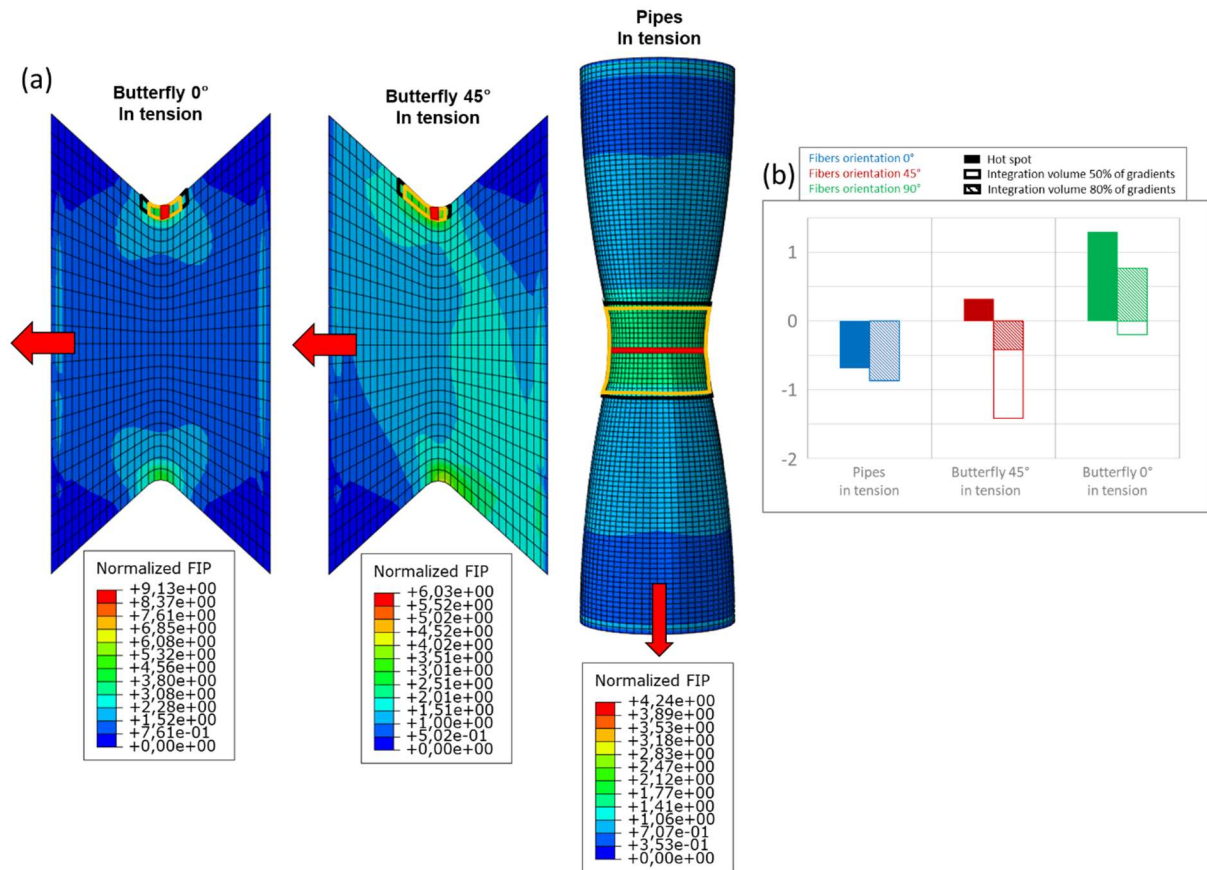
Figure 4-26 : (a) Représentation des volumes d'intégration pour un seuil fixé à 50% (Encadrés noirs) ou 80% (Encadrés jaunes) du gradient maximal de FIP et des points chauds (Rectangles rouges) sur la cartographie du FIP aux nœuds en surface des éprouvettes. Epreuves papillon à 0° et à 45° et tubes en traction à R=0. Les cartographies sont réalisées au niveau de charge le plus élevé des courbes S-N ; (b) Ecart (en décades) entre durées de vie expérimentales et durées de vie prédites avec le volume d'intégration ou avec la méthode « point chaud ». Le volume d'intégration employé prend en compte 50% ou 80% du gradient maximal de FIP. Les écarts mentionnés sont moyennés sur tous les niveaux de chargement de la courbe S-N considérée.
