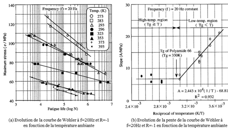
Figure 1-13 : Influence de la température de travail sur la courbe de Wöhler d'un PA6GF33 DAM pour des essais de traction-compression uniaxiale à R=-1 et f=20\text{Hz} [Hand99]
