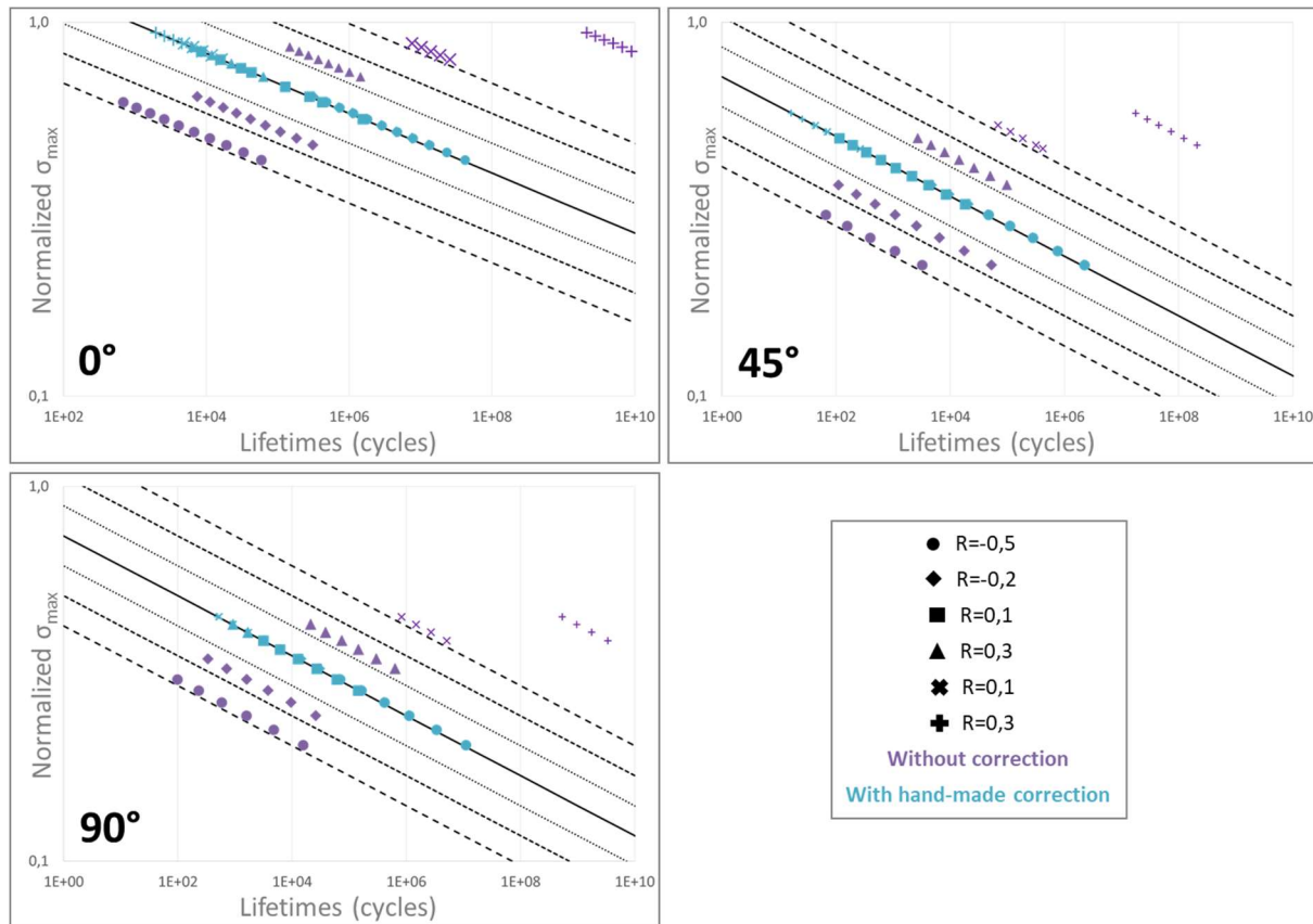
Figure 4-5 : Courbes de Wöhler simulées avec et sans correction de contrainte moyenne pour tous les rapports de charge de la base de données sur éprouvettes Dogbone.
