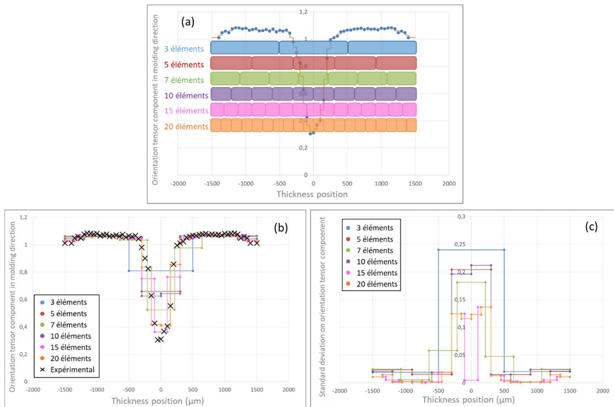
Figure 3-15 : (a) Représentation des discrétisations dans l'épaisseur superposées à la composante a_{11} du tenseur d'orientation dans le sens de la sollicitation pour une éprouvette à 0^\circ ; (b) Composante dans la direction d'injection du tenseur d'orientation dans un élément pour les discrétisations étudiées ; (c) Ecarts-types de l'orientation des fibres dans un élément pour les discrétisations étudiées
