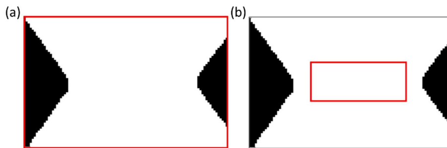
Figure 2-21 : Zone sur laquelle est moyennée la déformation lorsqu'elle l'est (a) dans la partie utile ; (b) dans la zone centrale
