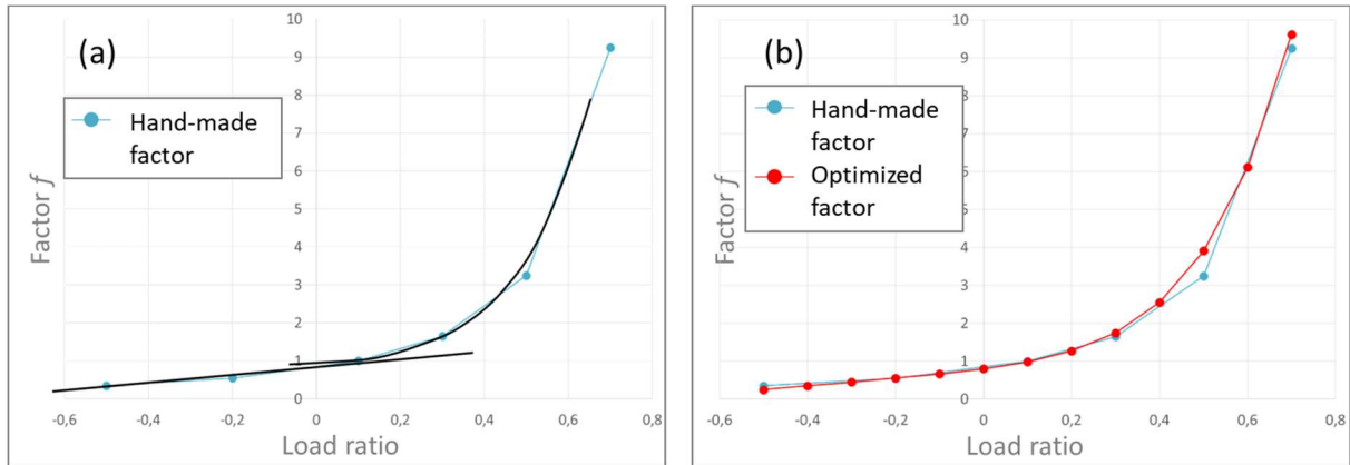
Figure 4-6 : (a) Evolution du facteur f évalué à la main et superposition d'une courbe puissance et d'une courbe linéaire pour différents domaines de rapports de charge ; (b) Evolution du facteur f évalué à la main et du facteur f donné par (4-2) dont les paramètres ont été optimisés pour correspondre au mieux au facteur évalué à la main
