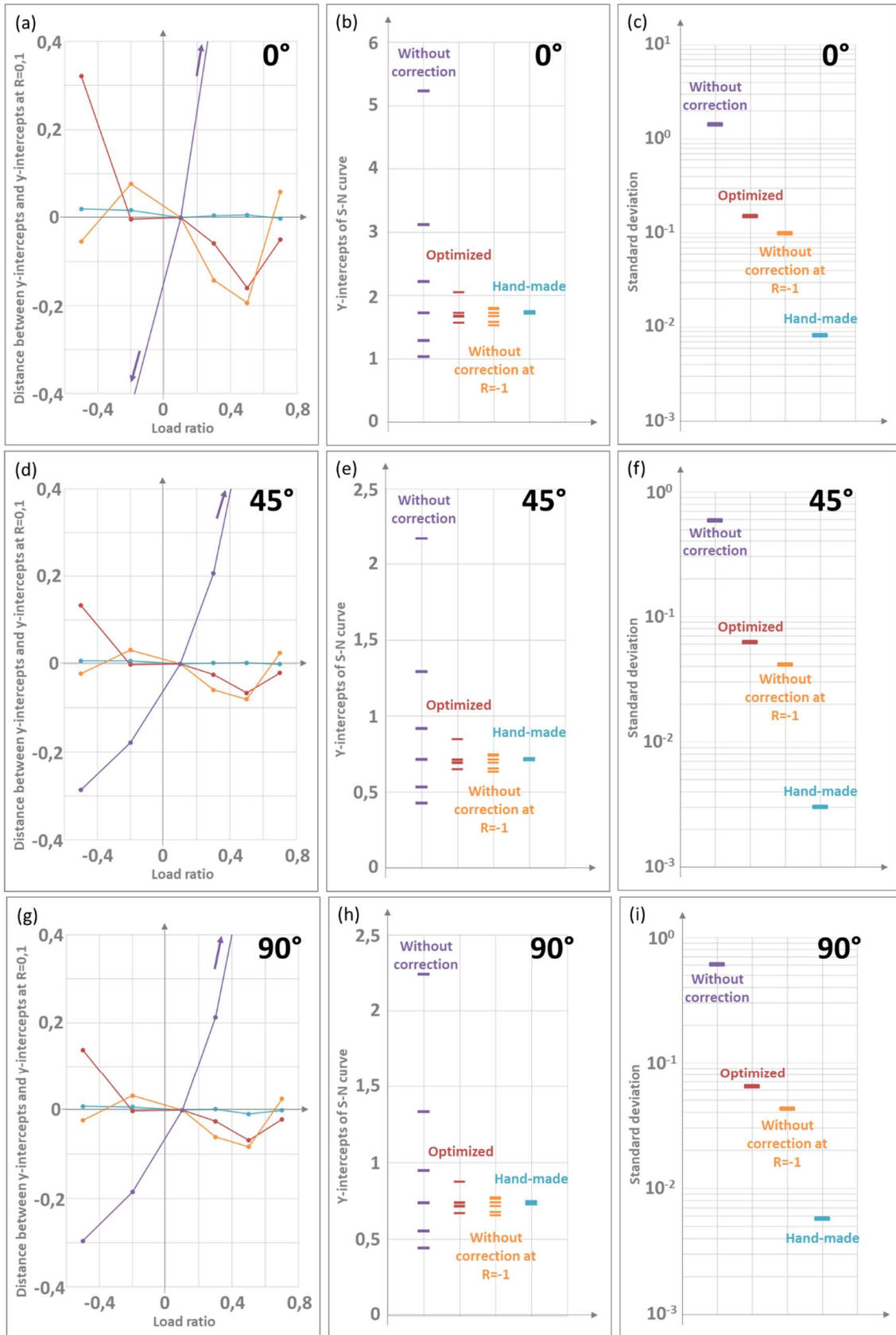
Figure 4-9 : (a, d, g) Ecart à l'ordonnée à l'origine de la courbe S-N brute à R=0,1 en fonction du rapport de charge pour chaque définition du facteur de correction de contrainte moyenne et pour chaque orientation ; (b, e, h) Ordonnées à l'origine des courbes S-N normées pour les six rapports de charge pour chaque définition du facteur de correction de contrainte moyenne et pour chaque orientation ; (c, f, i) Ecart-type des ordonnées à l'origine des courbes S-N sur l'ensemble des rapports de charge pour chaque définition du facteur de correction de contrainte moyenne et pour chaque orientation
