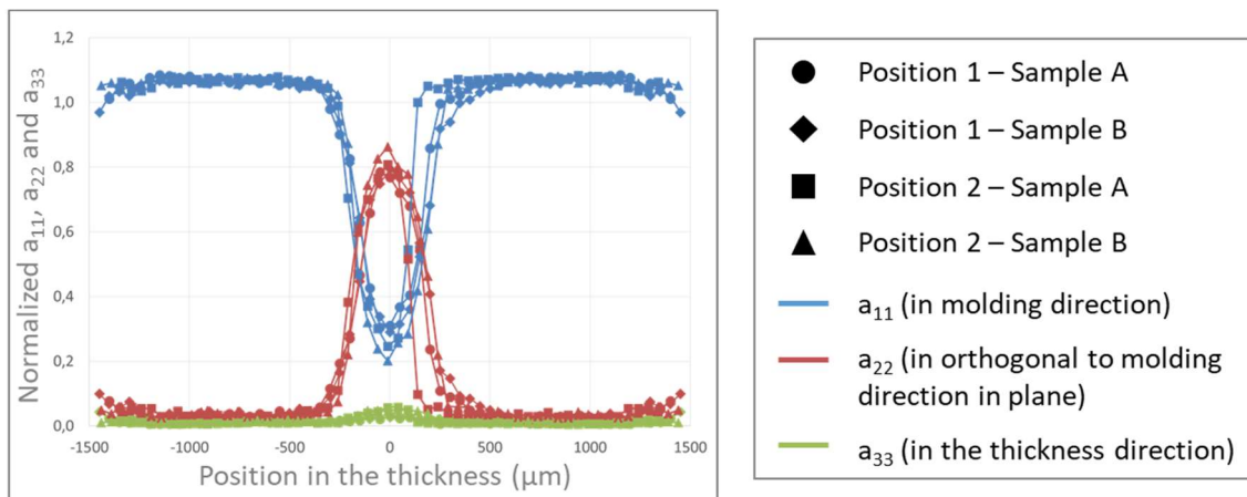
Figure 2-3 : Evolution des composantes diagonales du tenseur d'orientation dans l'épaisseur pour différents prélèvements aux deux positions de mesure évoquées à la figure 2-2
