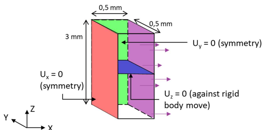
Figure 3-9 : Volume utilisé pour la procédure d'identification inverse, conditions aux limites et chargement appliqués
