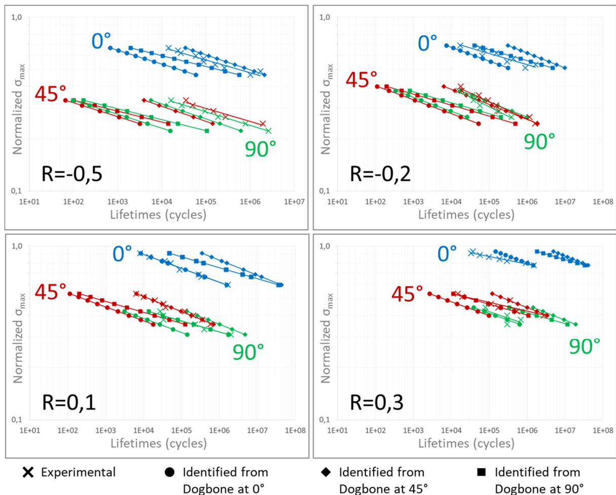
Figure 3-22: Résultats obtenus en traction à R=0.1 sur les Dogbone pour différents rapports de charge avec trois stratégies différentes d'identification du critère : identifications sur les éprouvettes à 0^\circ , 45^\circ et 90^\circ
