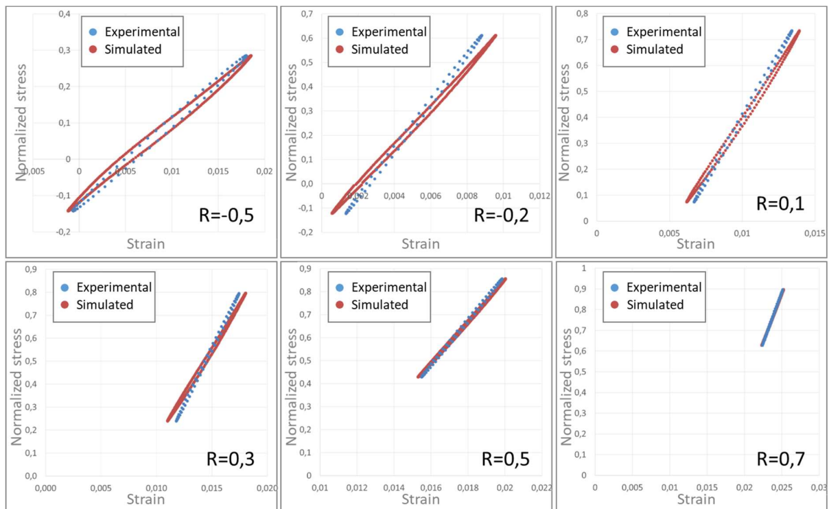
Figure 3-12 : Boucles d'hystérèse calculées et expérimentales dans la direction de sollicitation pour des essais uniaxiaux menés sur éprouvettes Dogbone à 0^\circ pour une durée de vie d'environ 3.10^4 cycles et pour différents rapports de charge
