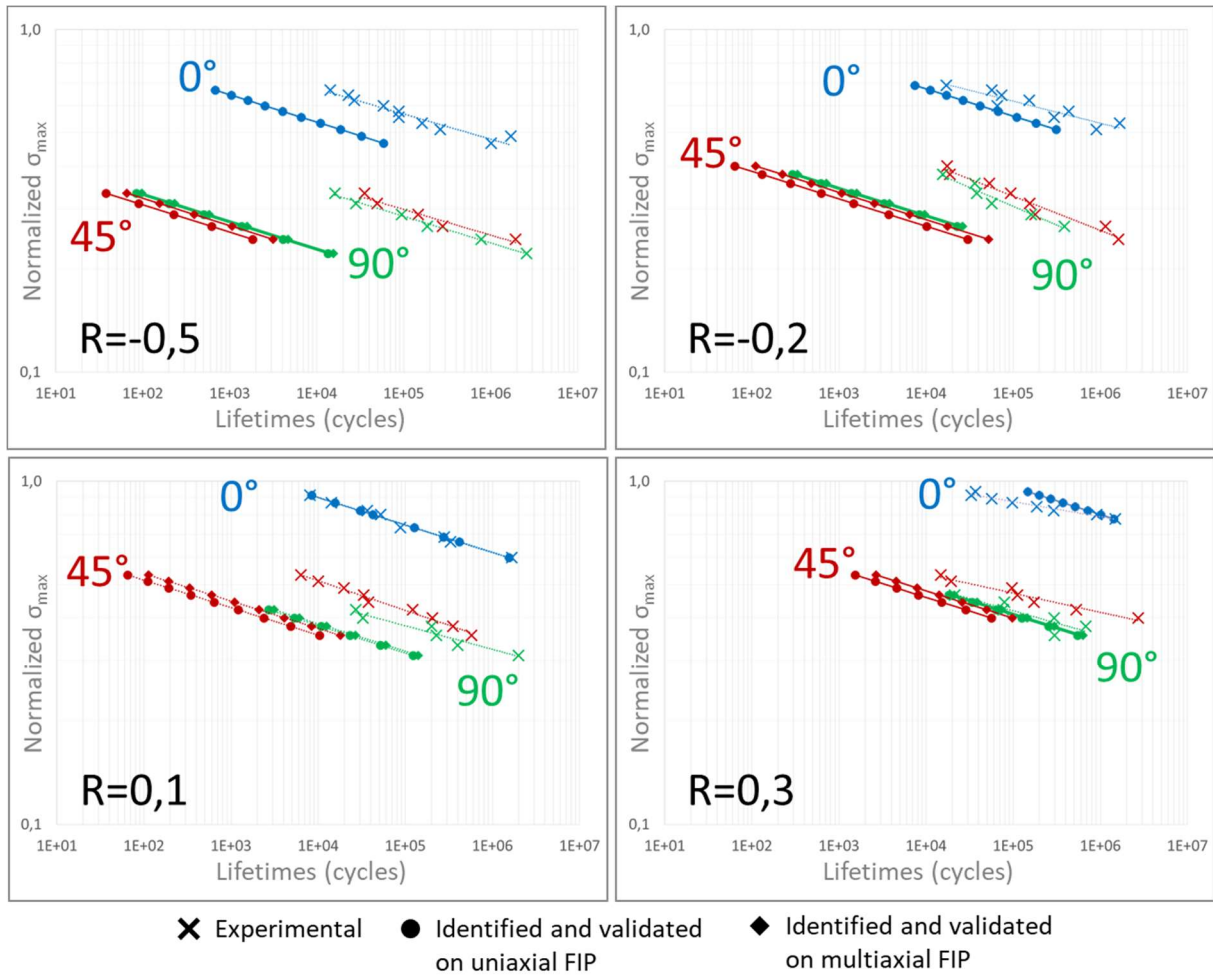
Figure 3-31 : Courbes S-N obtenues selon différentes stratégies de calcul du FIP pour l'identification et la validation du critère de fatigue pour les éprouvettes Dogbone en traction, les quatre rapports de charge et les trois orientations. Les courbes S-N expérimentales sont reportées pour comparaison
