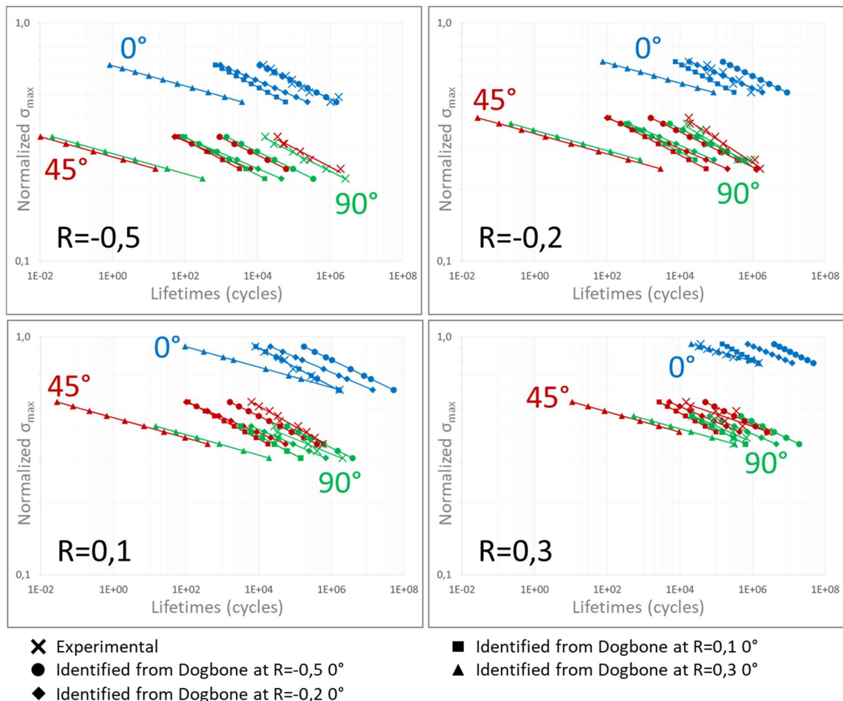
Figure 3-24 : Résultats obtenus en traction sur les Dogbone pour différents rapports de charge avec quatre stratégies différentes d'identification du critère : identifications sur les éprouvettes à R=-0.5, -.2, 0.1 et 0.3
