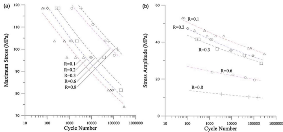
Figure 1-21 : Courbes de Wöhler en (a) amplitude de contrainte et (b) contrainte maximale obtenues en traction uniaxiale pour différents rapports de charge sur du PA66GF33 orienté à 0° à l'ambiante à f=1\text{Hz} [Mall04]
