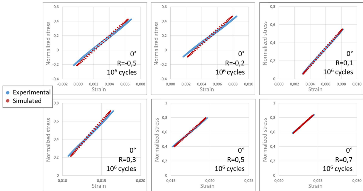
Figure A-6 : Boucles d'hystérèse calculées et expérimentales dans la direction de sollicitation pour des essais uniaxiaux menés sur éprouvettes Dogbone à 0° pour une durée de vie d'environ 10^6 cycles et pour différents rapports de charge
