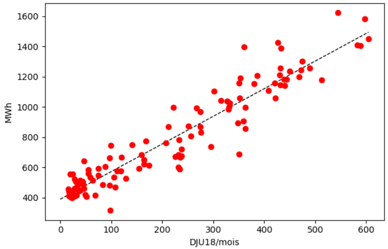
Figure 28 : Sensibilité climatique du centre administratif de l'Eurométropole de Strasbourg, pour chaque mois entre 2009 et 2017.
