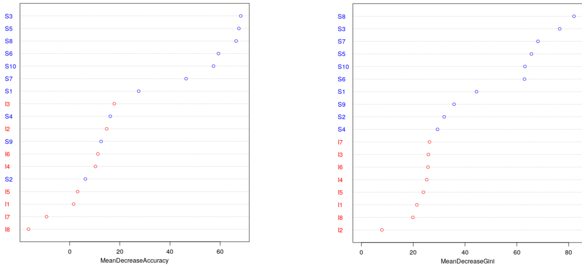
FIGURE 4.17 – Indice d'utilité des différentes caractéristiques (tri croissant)
