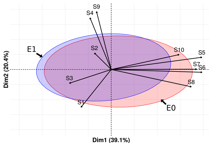
FIGURE 4.19 – ACP selon les deux premières composantes
