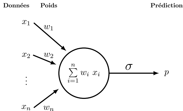
FIGURE 2.7 – Représentation d'un neurone seul
