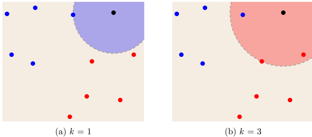
FIGURE 2.2 – Exemple de KNN
