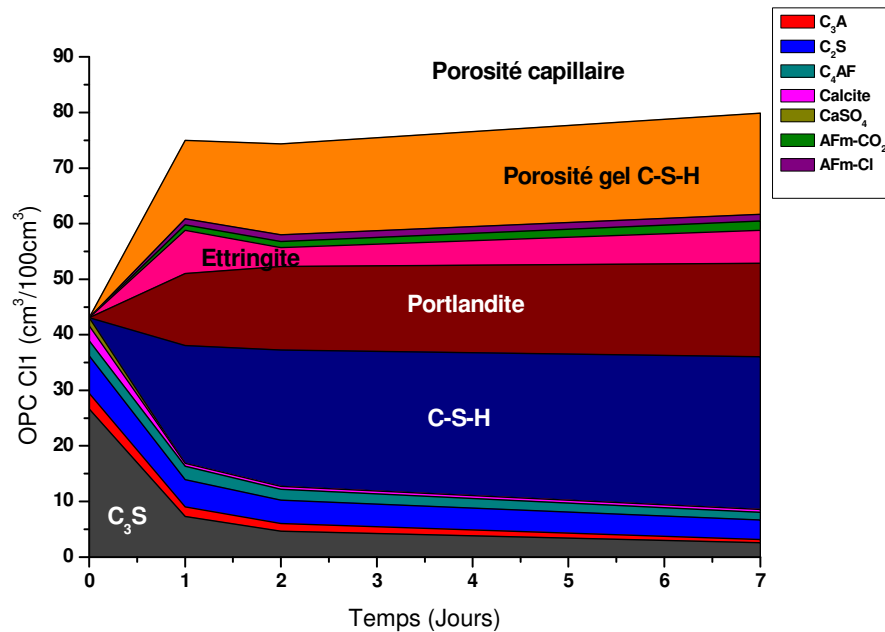
Figure IV-43 Assemblage de phases du système OPC CII
