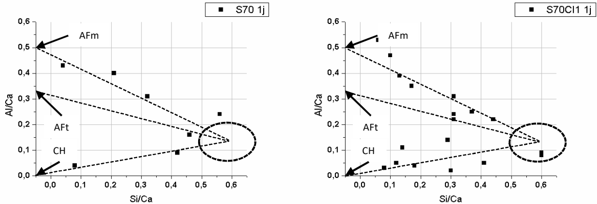
Figure IV-19 Ratios \text{Al}/\text{Ca} et \text{Si}/\text{Ca} des phases hydratées mesurées par EDS pour les échantillons S70 et S70Cl1 à 1j. La surface du cercle représente une composition moyenne de C-S-H purs
