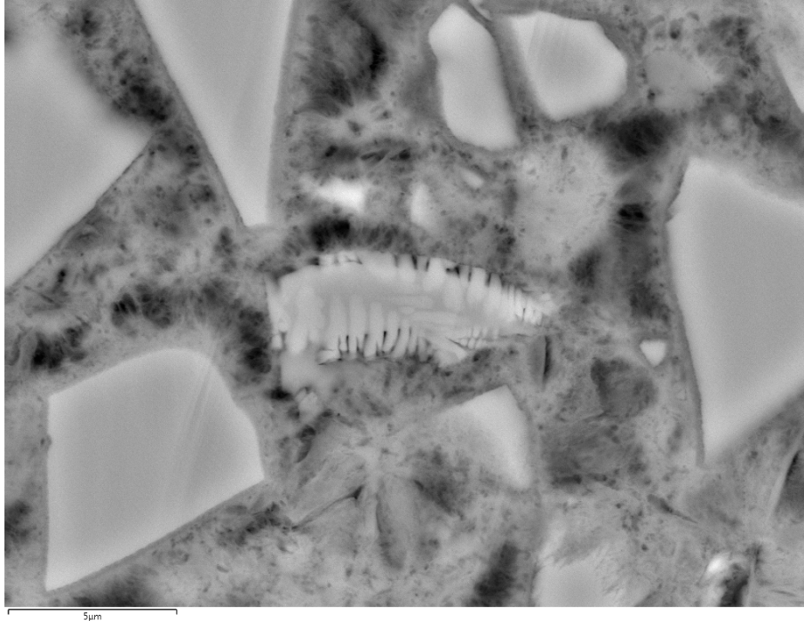
Figure II-1 Image MEB d'un échantillon S70C11 après 7 jours d'hydratation (x5000)
