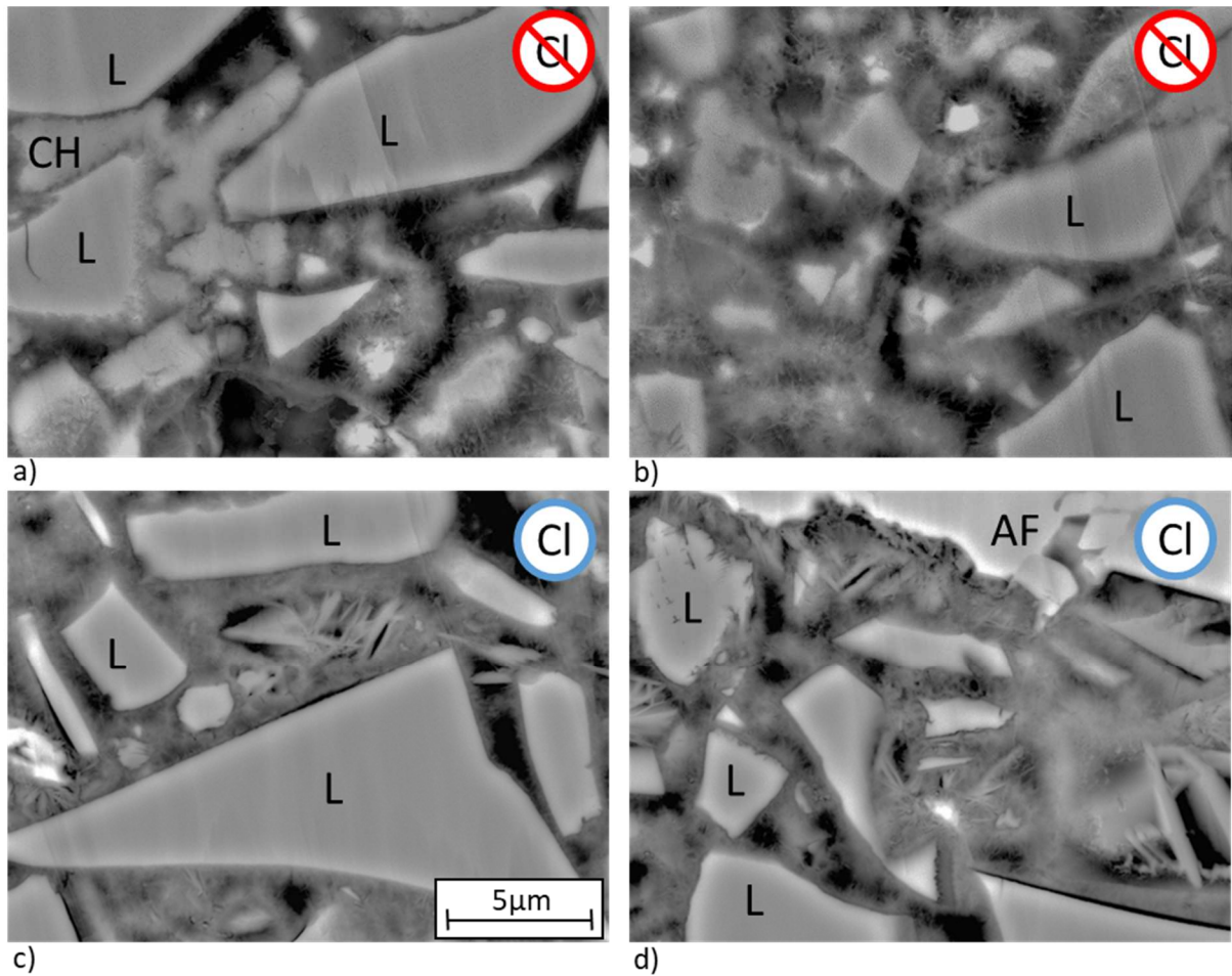
Figure IV-15 Images S70 (a et b) et S70Cl1 (c et d) à 48h de réaction
