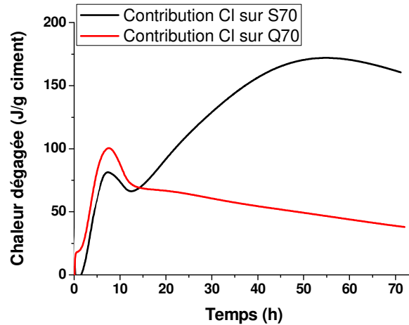
Figure III-13 Comparaison des contributions de l'ajout de \text{CaCl}_2 sur le dégagement de chaleur pour les mélanges S70 et Q70
