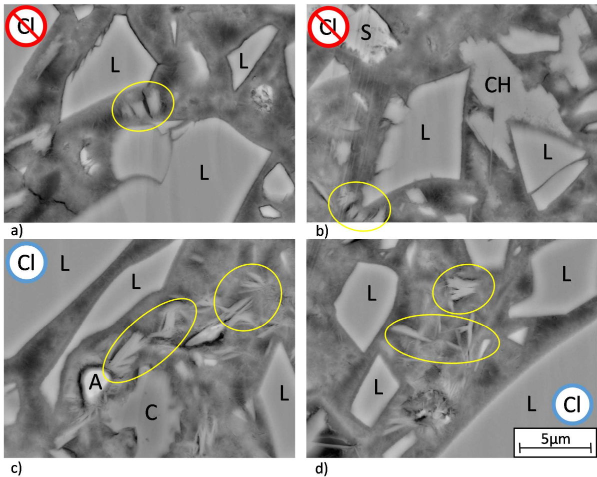
Figure IV-17 Images S70 (a et b) et S70Cl1 (c et d) à 7 jours de réaction. Les zones entourées en jaune montrent des AFm
