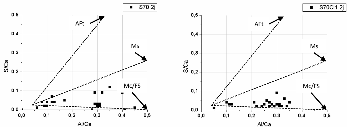
Figure IV-23 Ratios S/\text{Ca} et \text{Al}/\text{Ca} des phases hydratées mesurées par EDS pour les échantillons S70 et S70Cl1 à 2j. Les lignes se rejoignent sur une composition moyenne de C-S-H purs
