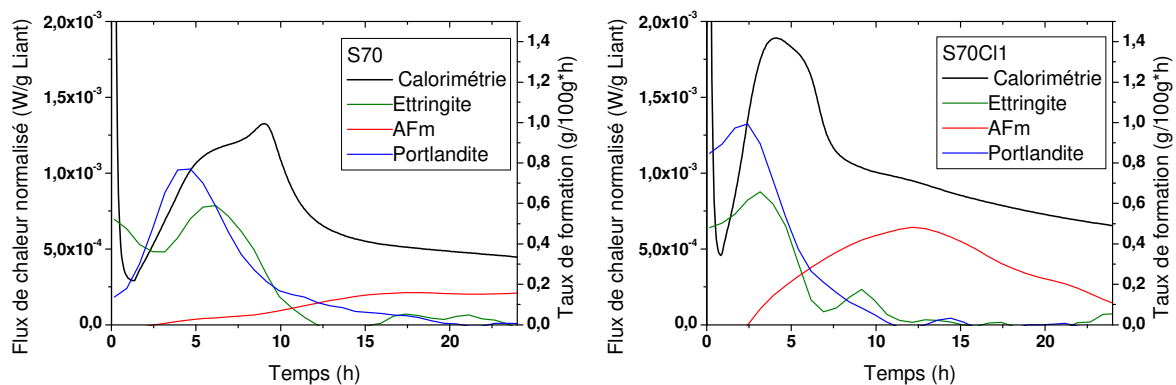
Figure V-16 Taux de formation des phases CH, AFt et AFm avec flux de chaleur correspondant pour les systèmes S70 (gauche) et S70C11 (droite)
