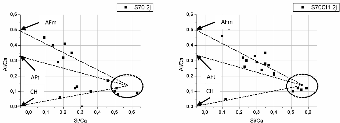
Figure IV-20 Ratios Al/Ca et Si/Ca des phases hydratées mesurées par EDS pour les échantillons S70 et S70Cl1 à 2j. La surface du cercle représente une composition moyenne de C-S-H purs
