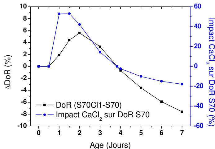
Figure IV-41 Ecarts de degré de réaction (DoR) entre le système S70 et S70Cl1 sur 7 jours de réactions (carrés noirs) avec écart relatif par rapport au DoR du système S70 (ronds bleus)
