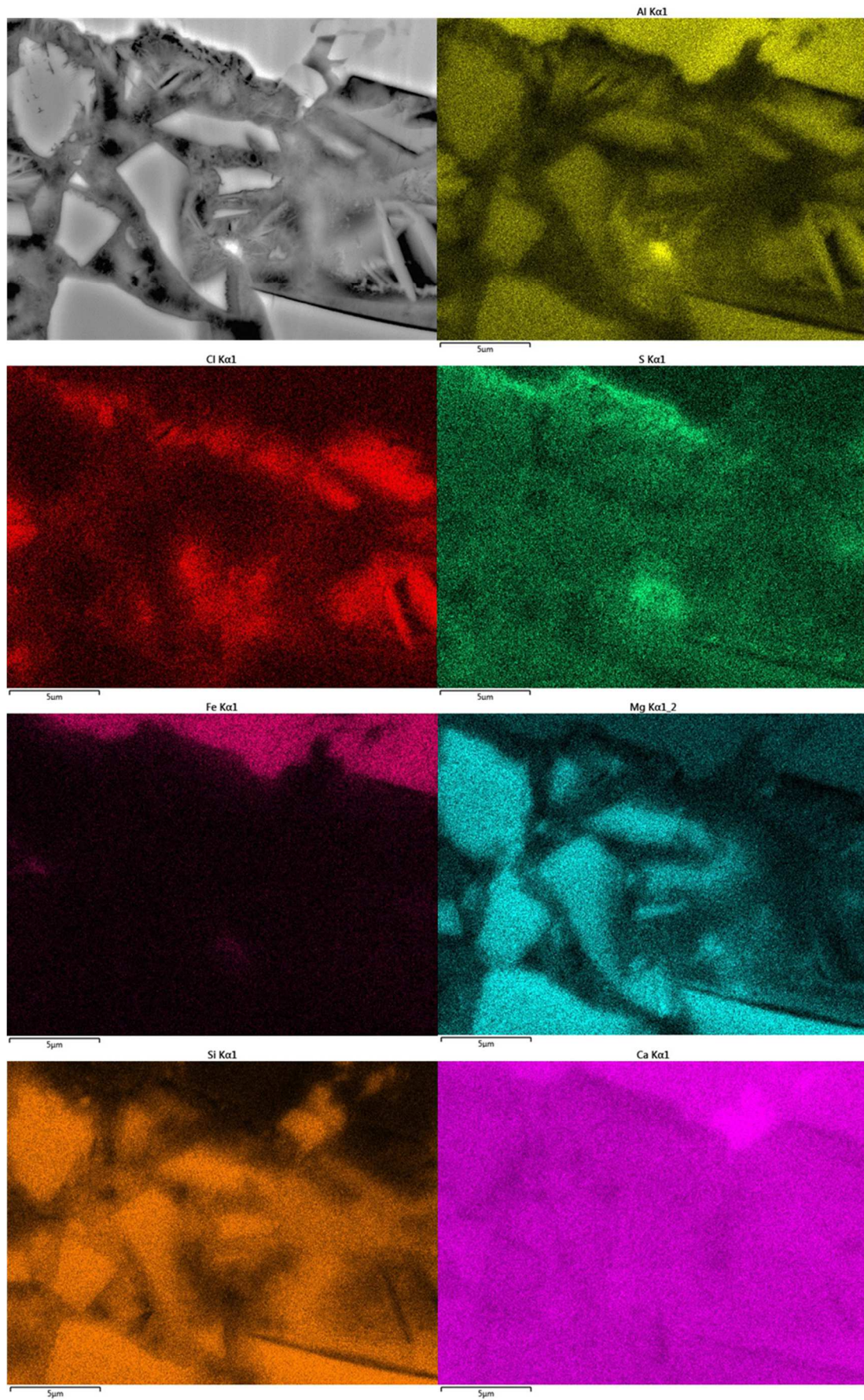
Figure IV-16 Image S70C11 à 48h de réaction avec cartographies EDS associées
