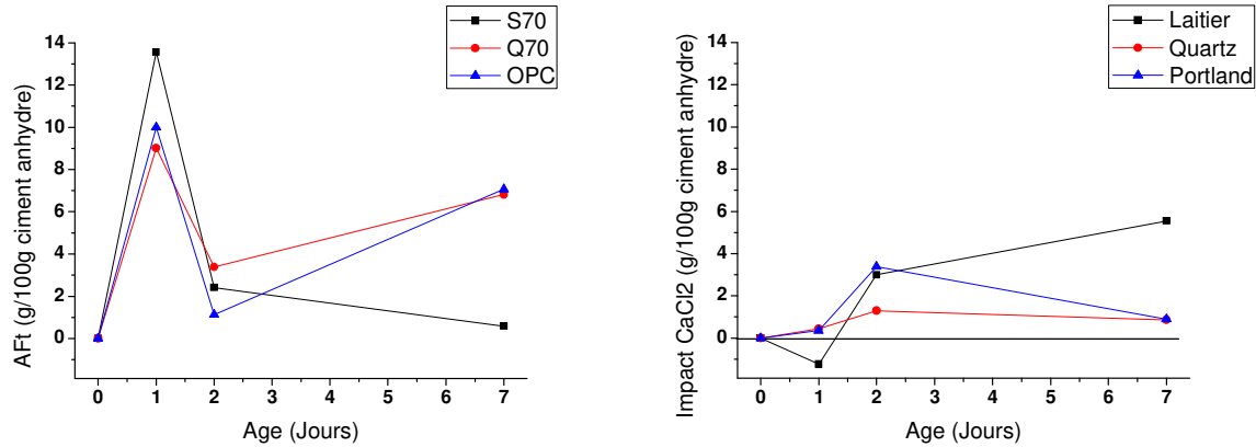
Figure IV-31 Formation d'ettringite normalisée sur la quantité de ciment (gauche) et impact du \text{CaCl}_2 (droite)
