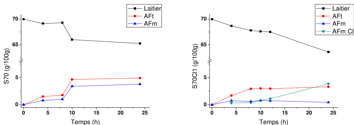
Figure V-29 Suivi quantitatif par RMN ^{27}\text{Al} des systèmes S70 et S70Cl1 pendant 24 heures.
