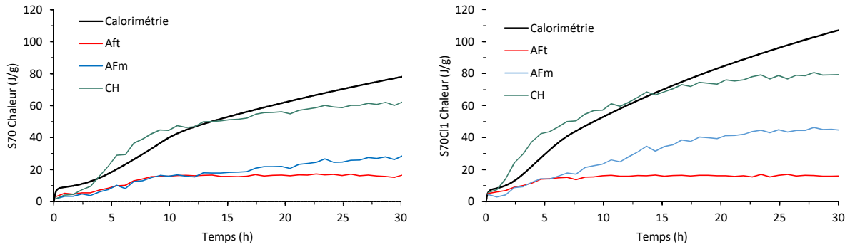
Figure V-18 Calcul alternatif pour les chaleurs dégagées dans les systèmes S70 et S70Cl1
