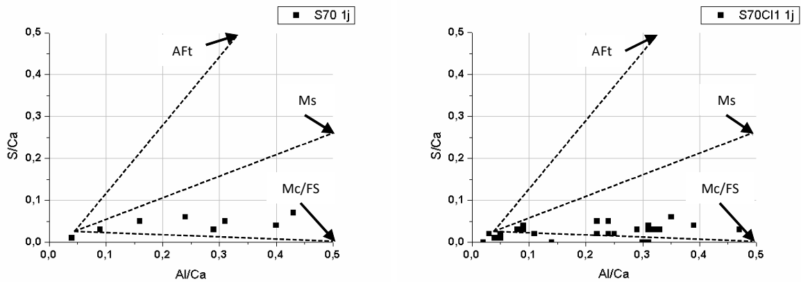
Figure IV-22 Ratios S/\text{Ca} et \text{Al}/\text{Ca} des phases hydratées mesurées par EDS pour les échantillons S70 et S70Cl1 à 1j. Les lignes se rejoignent sur une composition moyenne de C-S-H purs
