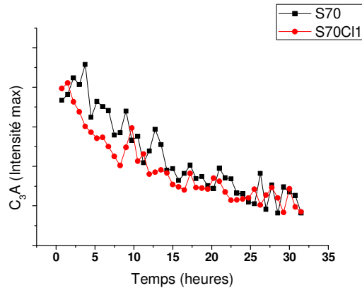
Figure V-8 Suivi de la consommation de \text{C}_3\text{A} par DRX in-situ dans les mélanges S70 et S70Cl1 (en intensité relative)
