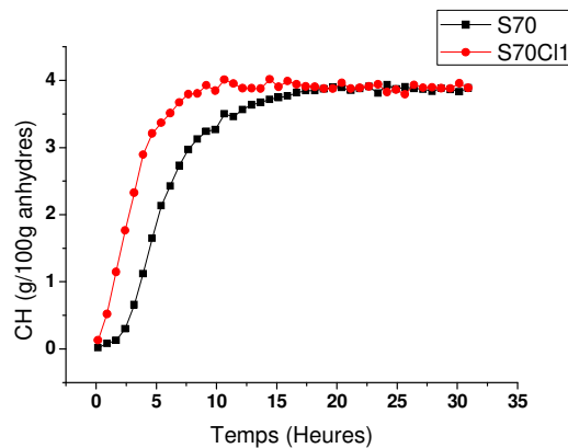
Figure V-2 Suivi de l'évolution de la formation de Portlandite par DRX in situ dans les systèmes S70 et S70C11
