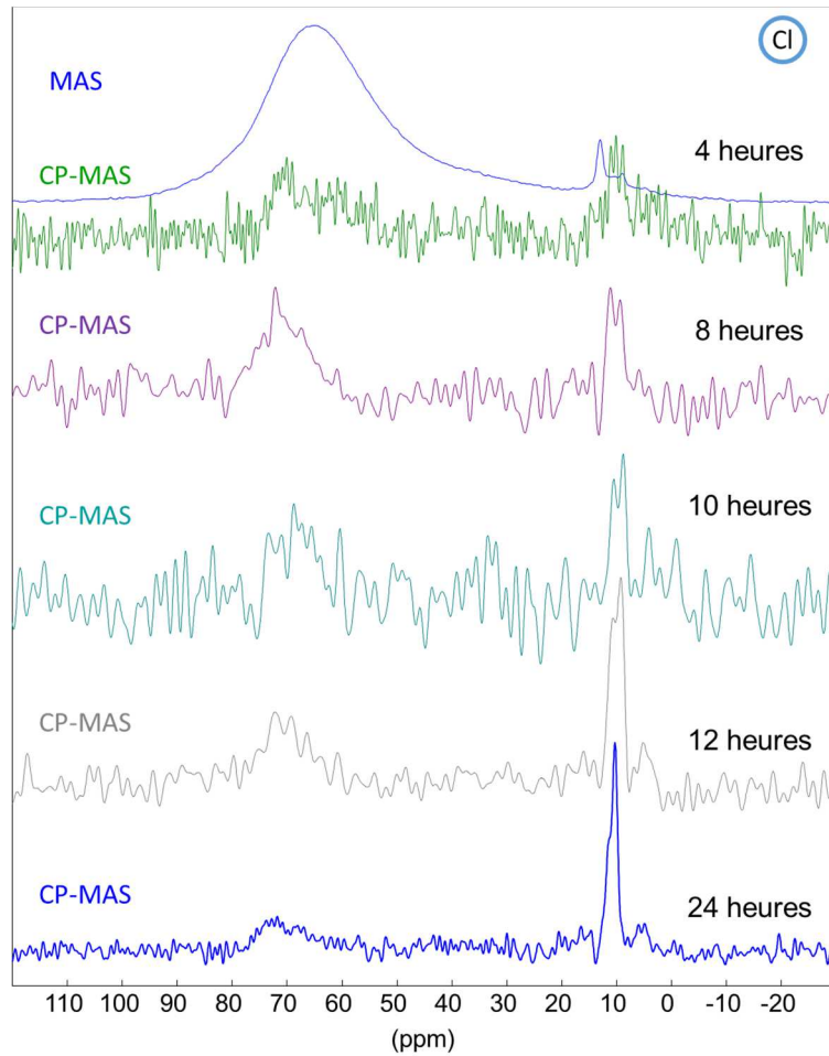
Figure V-31 Spectres ^1\text{H} - ^{27}\text{Al} (CP MAS) du système S70Cl1. Spectre ^{27}\text{Al} (MAS) à 4 heures en référence
