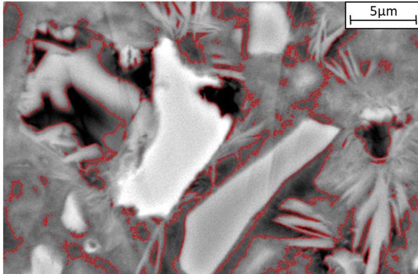
Figure IV-4 Résultat de la mesure de porosité par analyse d'image. Les zones encerclées représentent la porosité. Echantillon S70Cl1 après 7 jours
