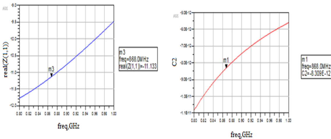
Figure 88 : L'impédance ( R=-11 \Omega en parallèle avec C= -8.2\text{pF} ) synthétisée à la sortie du circuit NIC proposé
