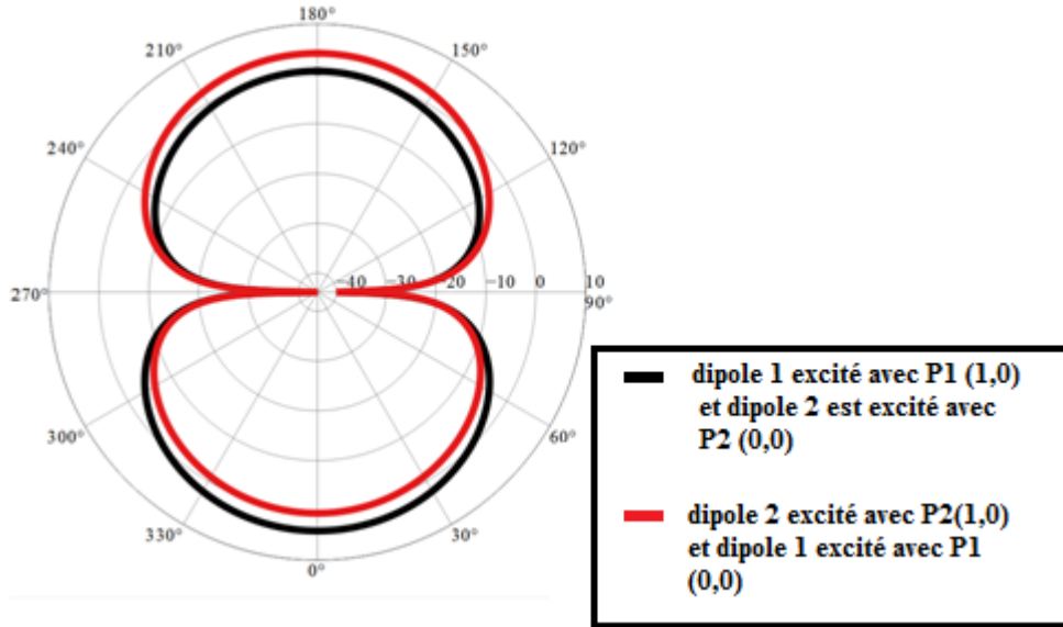
Figure 30 : Directivité 2D totale simulée du réseau d'antennes proposé à 868 MHz dans le plan d'azimut lorsque les deux dipôles sont excités de façon alternative.
