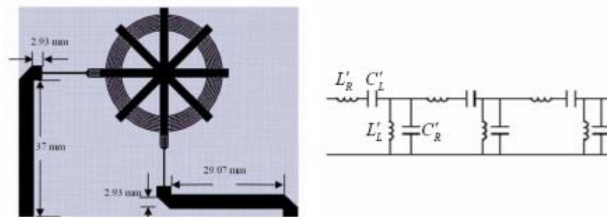
Figure I.10 : antenne basée sur le concept de « Composite Right-/Left-Handed Transmission Line « CRLH »
