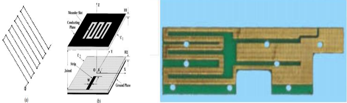
Figure I.5 : Géométrie de l'antenne méandre dans [9]
