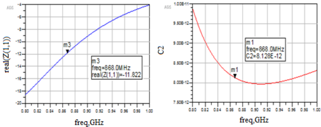
Figure 87: L'impédance ( R=-11 \Omega en parallèle avec C= 8.2\text{pF} ) synthétisée à la sortie du circuit NIC proposé
