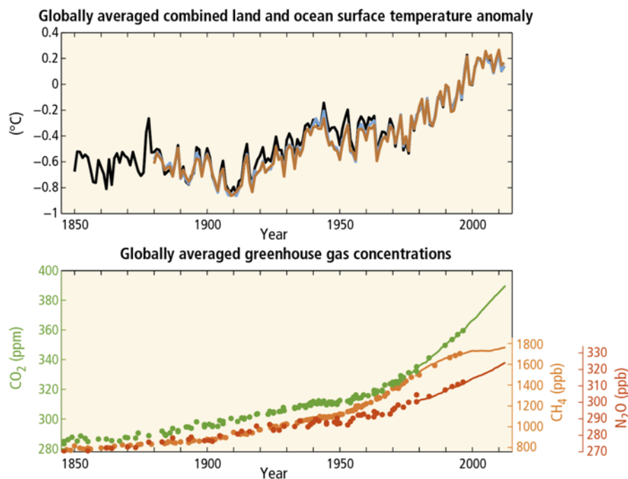
Figure 1 : Haut : anomalies de température globale depuis 1850 (les couleurs représentant des jeux de données différents). Bas : concentration globale de certains gaz à effet de serre (i.e. CO 2 , CH 4 et N 2 O). Extrait du 5 ème rapport d'évaluation du GIEC (IPCC 2014).
