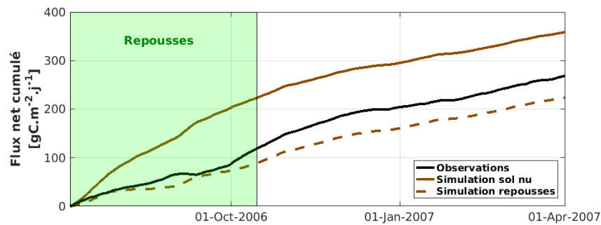
Figure IV-4 : Evolution temporelle du flux net de CO 2 cumulé pendant l'interculture 2006-2007 à Auradé. Les observations correspondent à la courbe noire. Les courbes correspondantes aux simulations sans et avec prise en compte des repousses sont respectivement en marron et marron pointillée.
