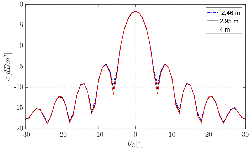
FIGURE 3.22 – SER d’une plaque métallique de dimension 148 \text{ mm} \times 151 \text{ mm} , issue d’une simulation sur HFSS, dans une configuration mono-statique, pour trois distances d’observation différentes
