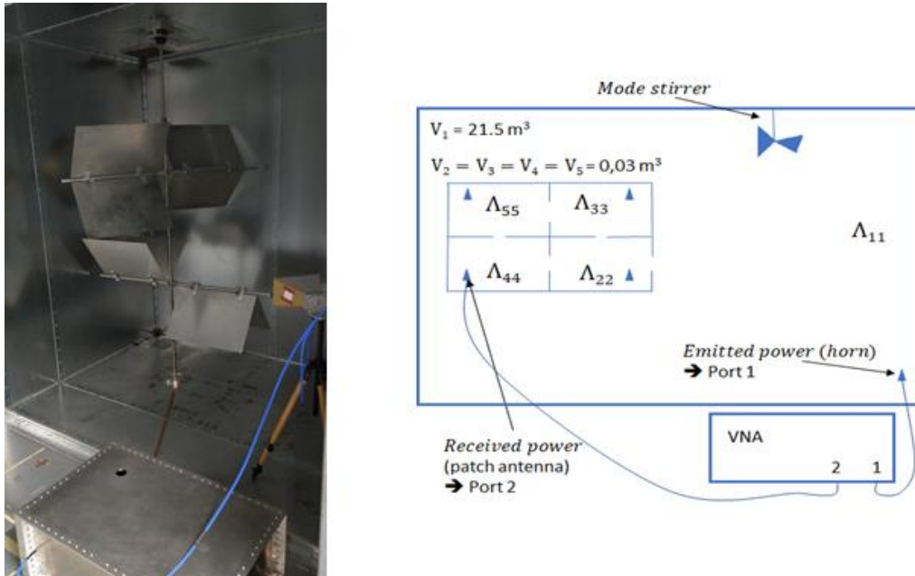
Figure 42 : Photographie et schéma du système à 5 cavités
