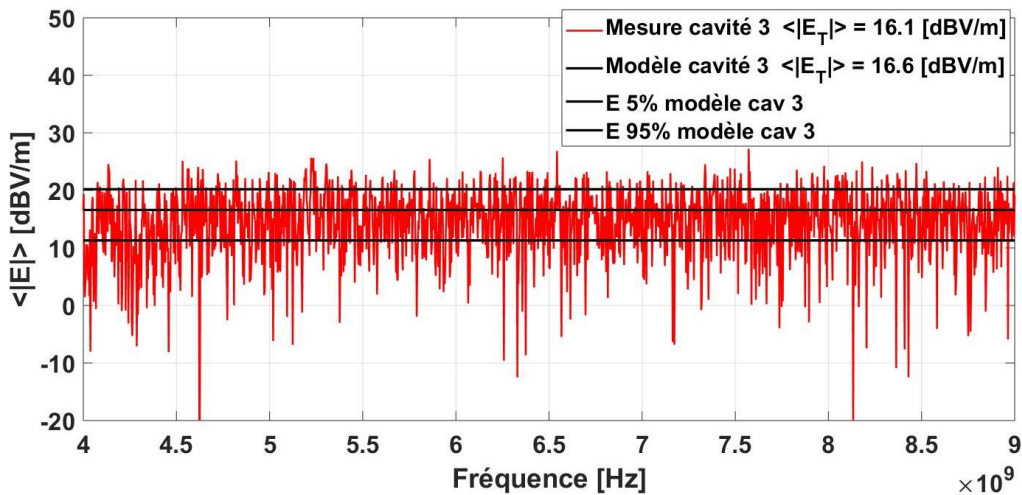
Figure 36 : Comparaison du champ électrique total déduit de la mesure et calculé par le modèle Power Balance au sein de la cavité n°3 pour le cas n°1
