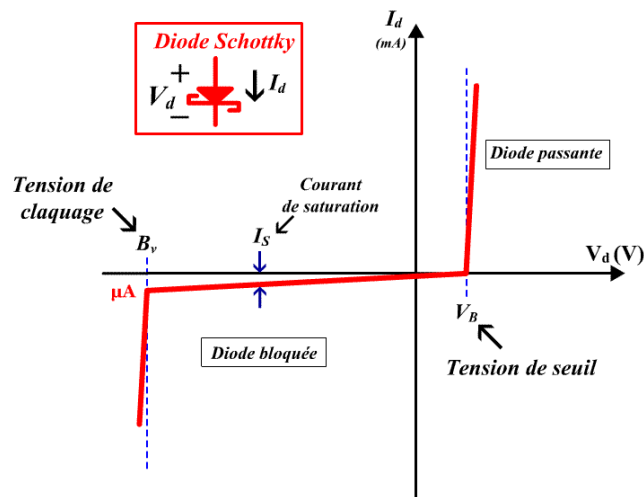
Figure 1-17 Caractéristique globale courant / tension d'une diode Schottky.
