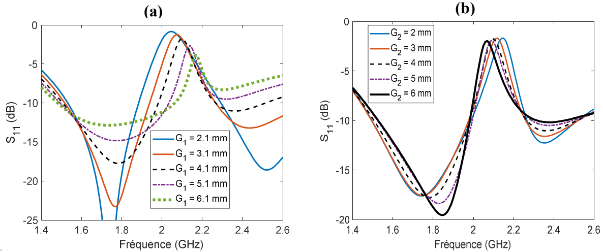
Figure 4-5 Evolution du coefficient de réflexion en fonction de : (a) gap G_1 et (b) gap G_2 .
