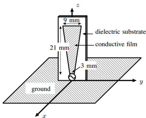
Figure 2-22 Configuration de l'antenne et le prototype réalisé [20].
