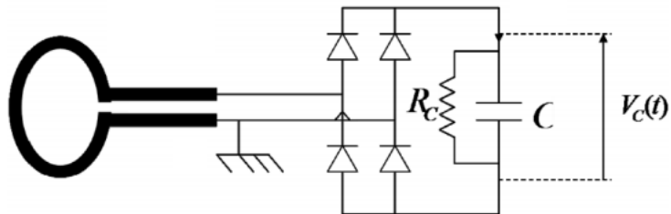
Figure 1-22 Exemple de rectenna en technologie CPS.
