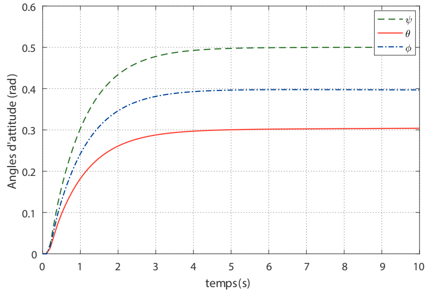
FIGURE 2.15 – Réponses du système en fonctionnement nominal : angles d'attitude.
