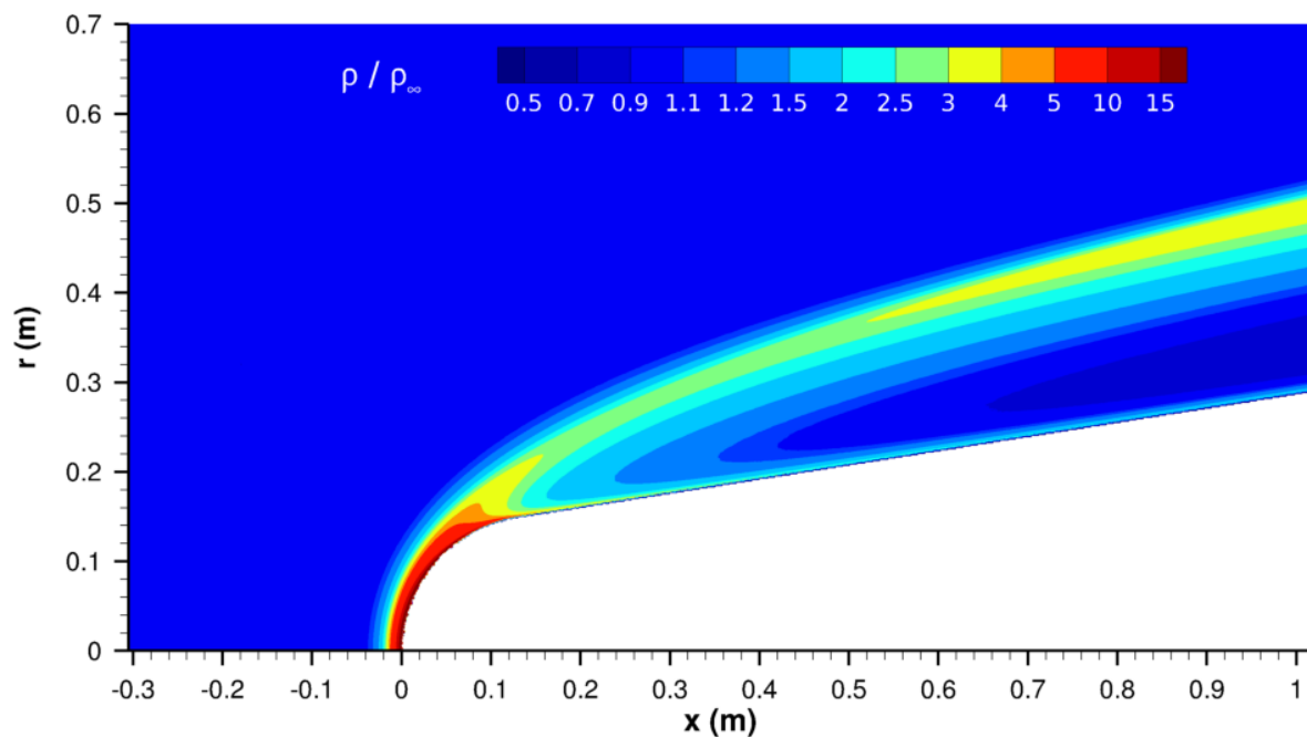
FIGURE 3.47 – Champ de masse volumique autour de la sonde RAM-C (81 km).
