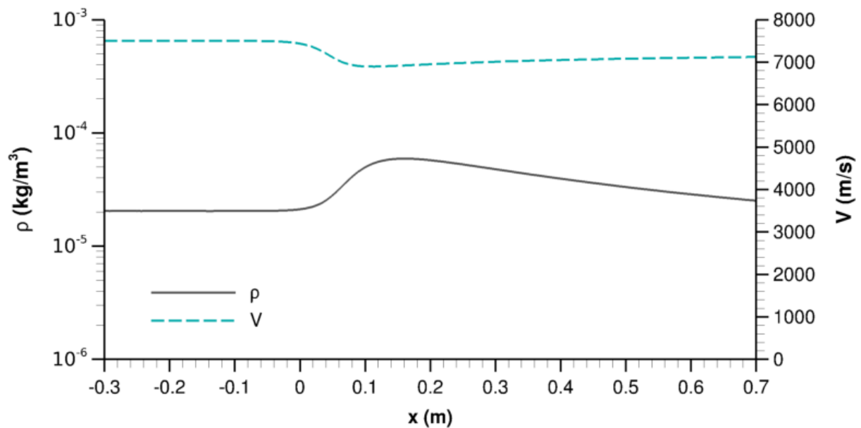
FIGURE 4.21 – Evolution de la vitesse et de la masse volumique sur la ligne de courant n°6.
