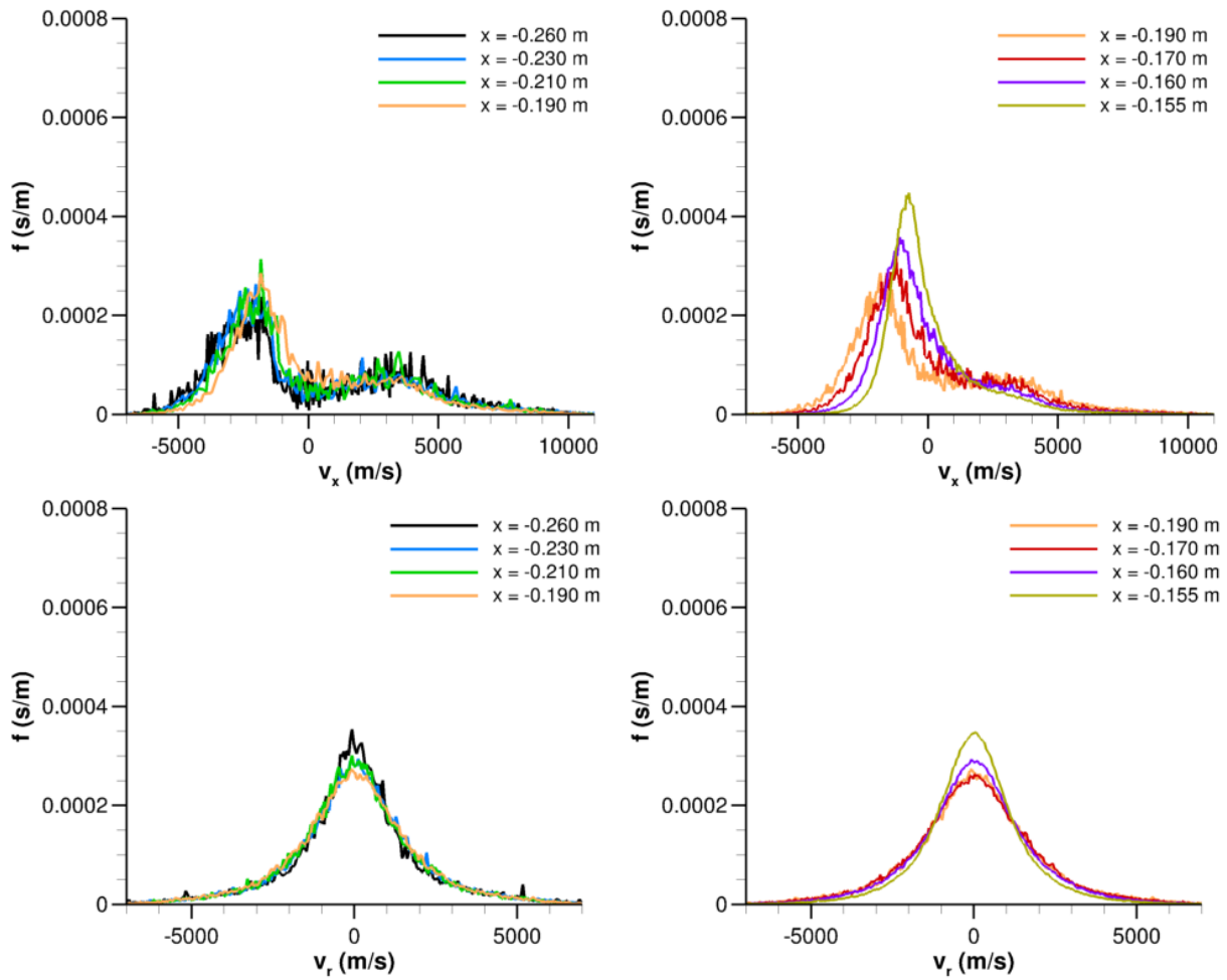
FIGURE 3.30 – Distribution de vitesse longitudinale v_x ( haut ) et radiale v_r ( bas ) de O à différents endroits le long de la ligne de courant du point d'arrêt ( Kn = 0, 1 ).
