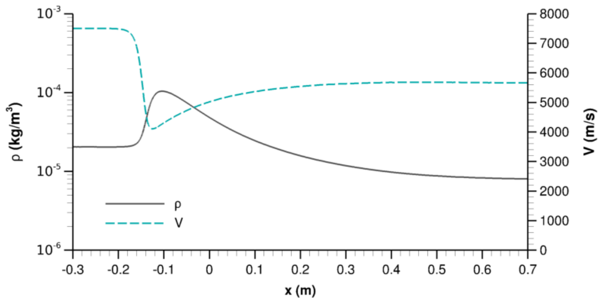
FIGURE 4.12 – Evolution de la vitesse et de la masse volumique sur la ligne de courant n°3.
