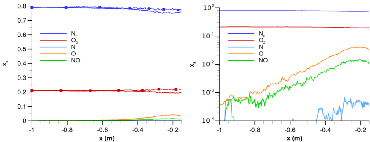
FIGURE 3.37 – Fraction molaire des différentes espèces chimiques le long de la ligne de courant du point d'arrêt ( Kn = 1 ).
