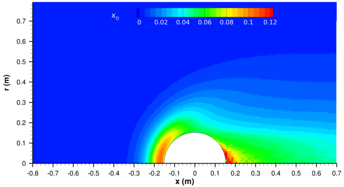
FIGURE 3.23 – Fraction molaire d'oxygène atomique ( Kn = 0, 1 ).
