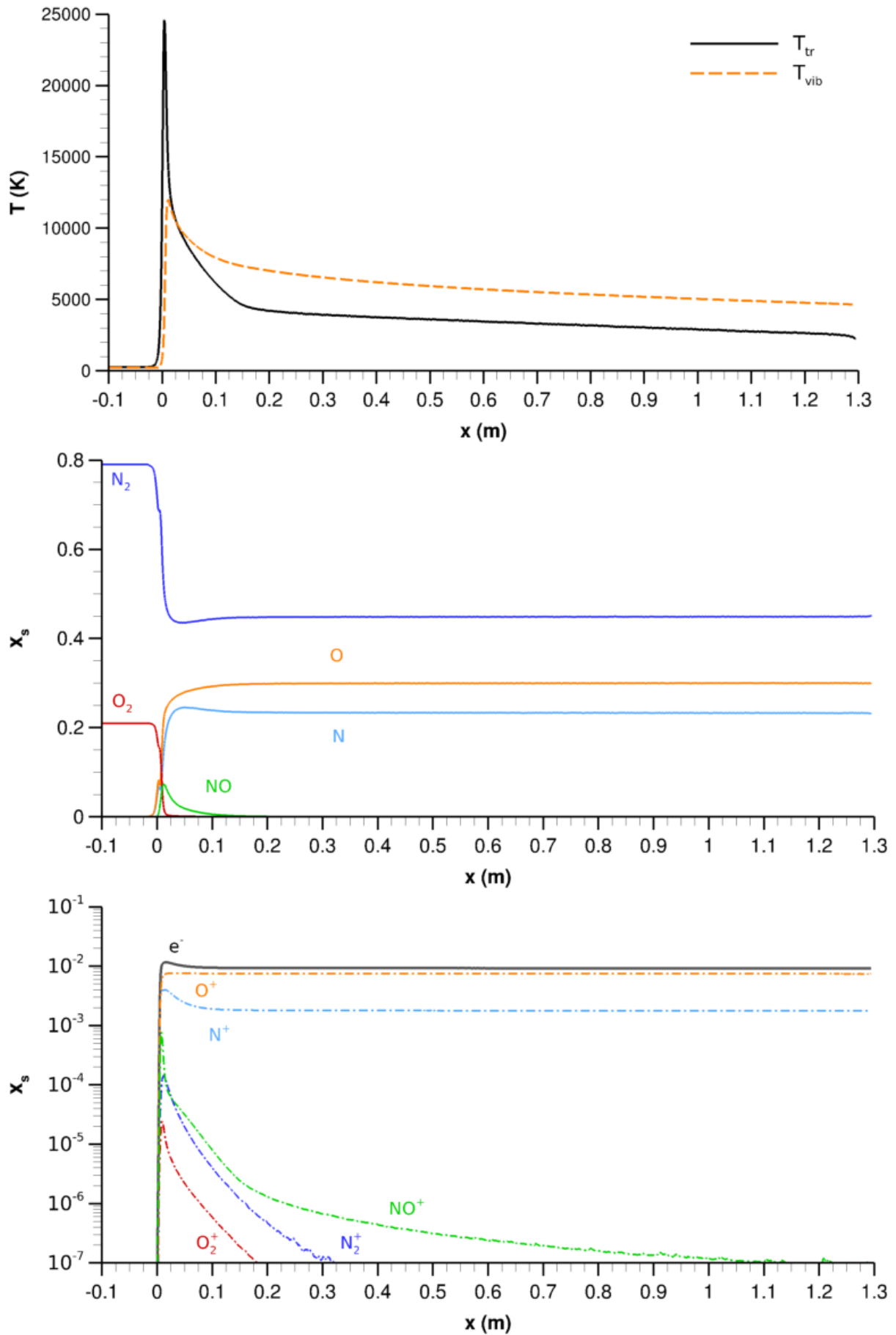
FIGURE 4.47 – Evolution de la composition chimique et des températures le long de la ligne de courant colorée en violet sur la figure 4.45 (RAM-C II 71 km).
