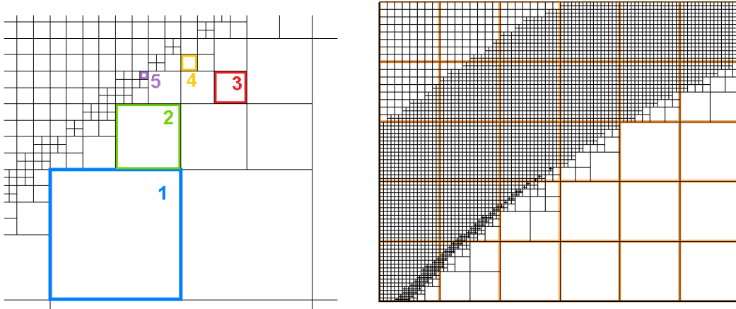
FIGURE 3.1 – A gauche : Schéma d'un maillage de type octree (ici en 2D). Les numéros désignent le niveau d'octree correspondant à la cellule. A droite : Schéma d'un domaine de calcul et son maillage dans SPARTA (ici en 2D). Les lignes colorées correspondent au maillage de fond, premier niveau de l'octree.
