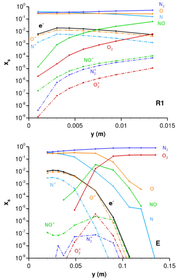
FIGURE 4.48 – Variation de la composition du gaz en fonction de la distance à la paroi au niveau des capteurs R_1 et E (RAM-C II 71 km).
