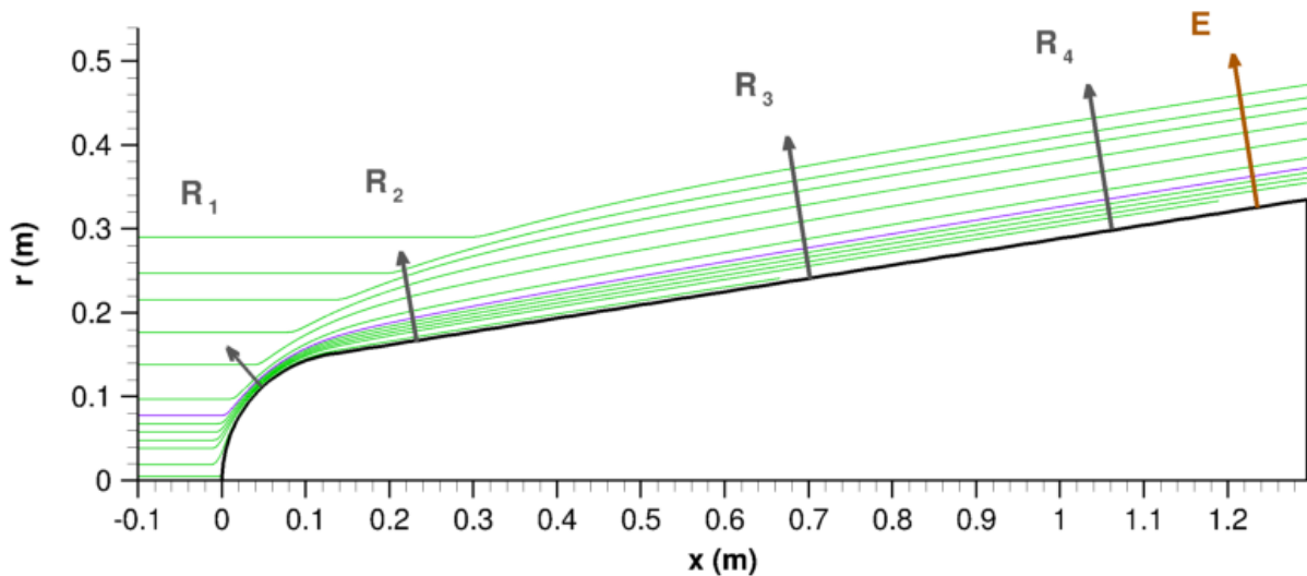
FIGURE 4.45 – Lignes de courant étudiées avec l’approche lagrangienne pour la configuration RAM-C II à 71 km.
