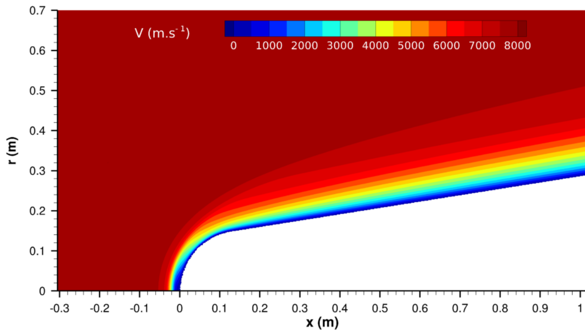
FIGURE 3.48 – Champ de vitesse autour de la sonde RAM-C (81 km).
