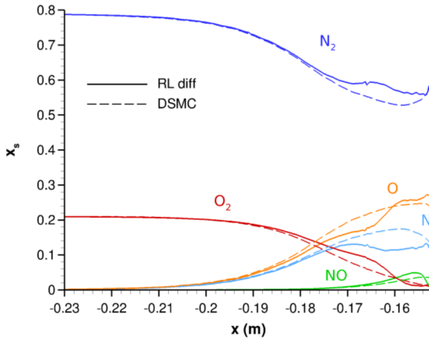
FIGURE 4.4 – Fractions molaires des espèces majoritaires recalculées avec le réacteur lagrangien, avec une prise en compte simplifiée de la diffusion massique.
