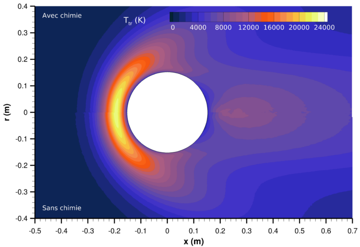
FIGURE 3.24 – Comparaison de température translationnelle ( Kn = 0, 1 ).
