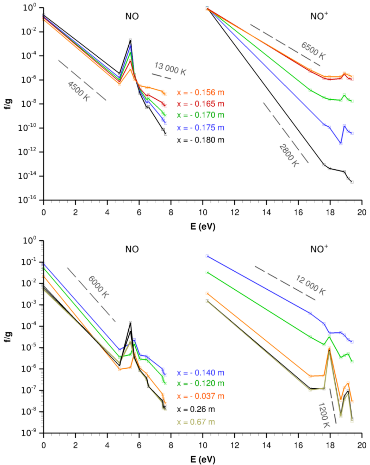
FIGURE 4.29 – Distribution des états électroniques de NO et NO + en différents points de la ligne de courant n°2.
