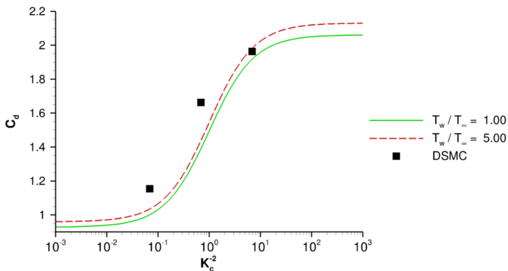
FIGURE 3.43 – Coefficient de traînée au point d'arrêt d'une sphère. Corrélations de Singh et Schwartzentruber et résultats des simulations DSMC.
