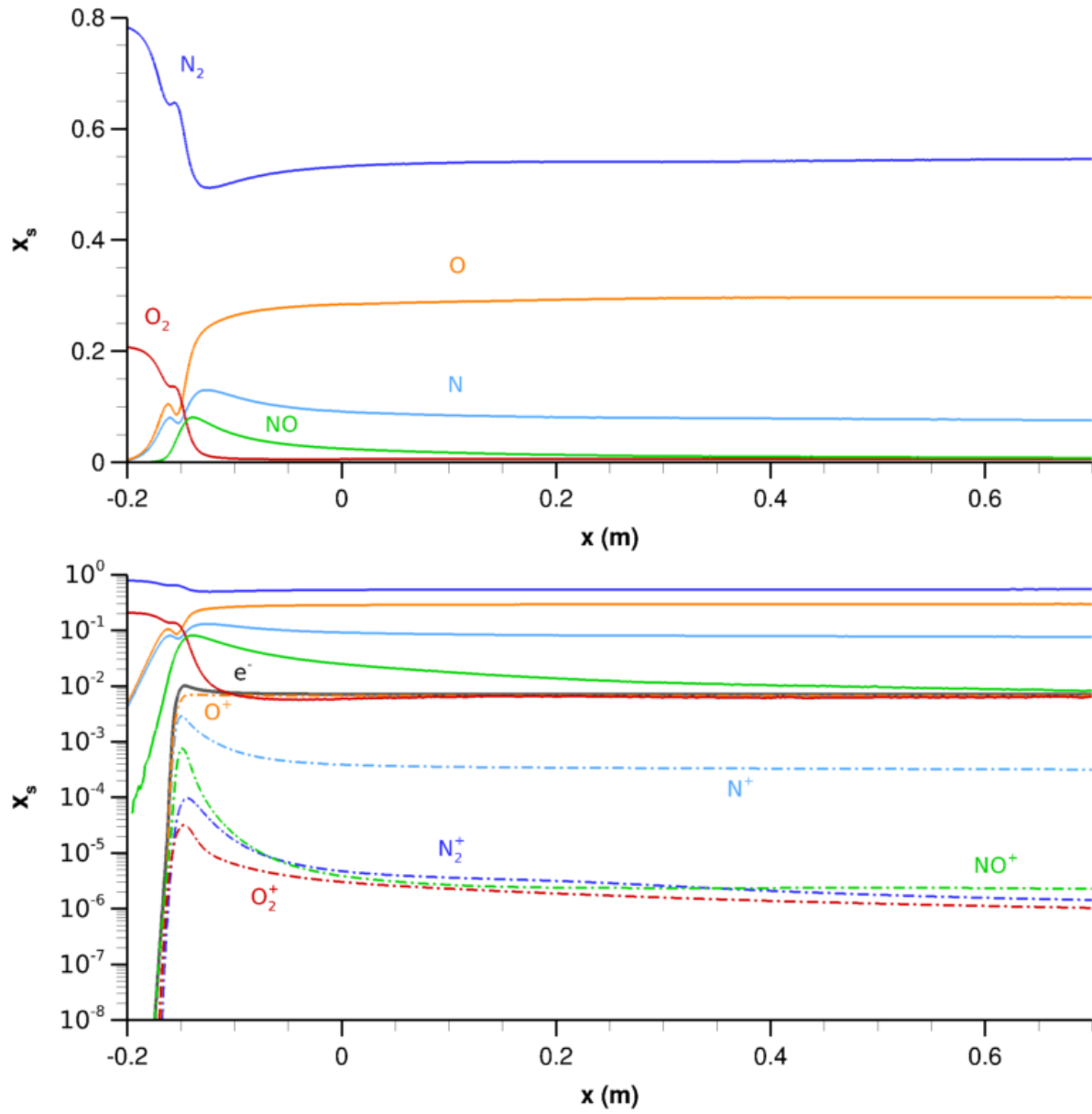
FIGURE 4.10 – Evolution de la composition chimique sur la ligne de courant n°2.
