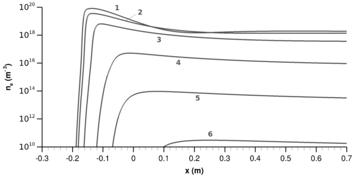
FIGURE 4.22 – Evolution de la densité électronique sur les lignes de courant autour de la sphère (cf. figure 4.8).
