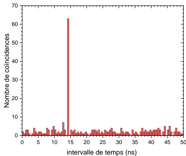
Figure V.11 : Histogramme de coïncidences entre les deux canaux de polarisations croisées en fonction du temps. L'intensité de pompe est fixée à 100mW. L'intégration est réalisée sur 2000s.
