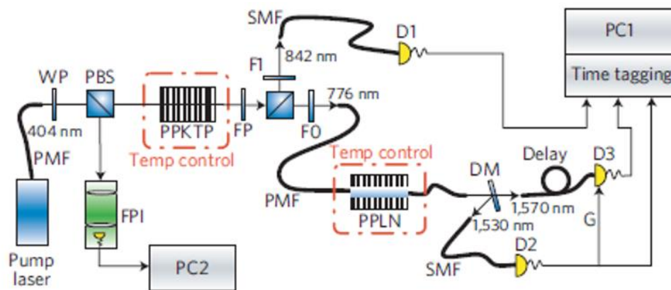
Figure II.7 : Montage expérimental de caractérisation de TPG indirecte par cascade quadratique. Le montage permet une mesure des coïncidences temporelles et de l'incertitude de l'énergie de pompe respectivement via des compteurs de photons uniques et un interféromètre. Tiré de [84].
