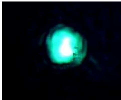
Figure III.16 : Cliché réalisé à la webcam du mode en sortie du guide 2. La section transverse du mode obtenu est proche de ce qui est attendu pour un mode de propagation fondamental.
