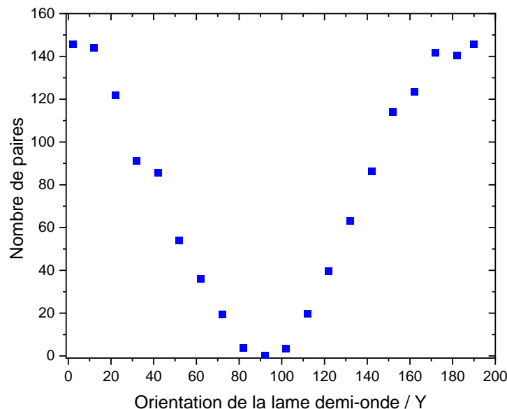
Figure V.15 : Evolution du nombre de paires en fonction de l'orientation de la lame demi-onde. A 0° et 180°, la pompe est polarisée selon la direction Y du cristal et l'interaction est donc la plus efficace.
