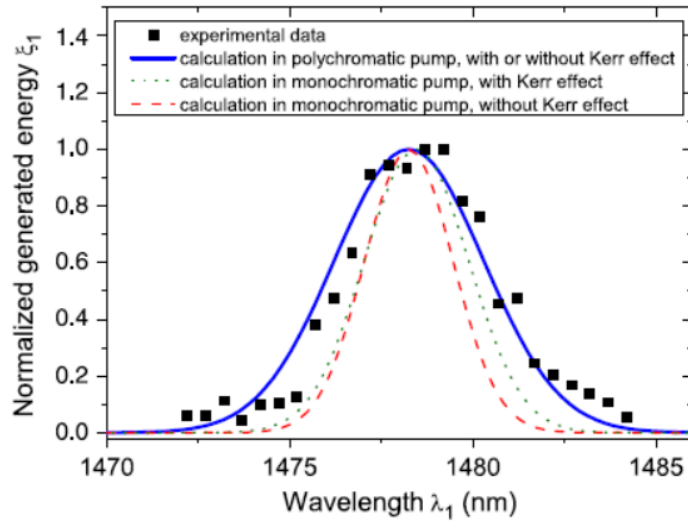
Figure II.4 : Comparaison entre le spectre généré à \omega_1 lors de la TPG bi-injectée et les calculs réalisés à partir de la modélisation quantique [35]. L'énergie de pompe incidente est \varepsilon_0 = 52\mu J et l'énergie de stimulation est (\varepsilon_2 + \varepsilon_2) = 68\mu J . En noir les points expérimentaux. En bleu la modélisation prenant en compte la polychromaticité de la pompe. En rouge la modélisation en pompe monochromatique et sans prendre en compte l'effet Kerr optique. En vert la modélisation monochromatique avec prise en compte de l'effet Kerr optique.
