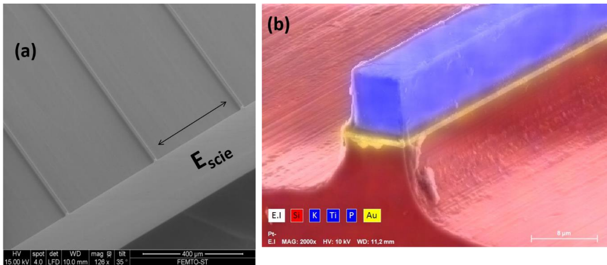
Figure III.3 : (a) Cliché MEB réalisé à l'institut Femto-ST qui présente des guides tracés par le passage de la scie. La distance entre les guides arêtes obtenus est égale à l'épaisseur de la scie (environ 200\mu\text{m} ). (b) Cliché MEB enrichi de l'analyse spectroscopique des éléments chimiques réalisé à l'Institut Néel de la face d'entrée d'un guide.
