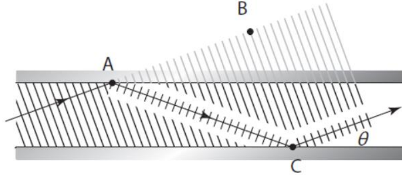
Figure III.8 : Guidage par réflexion totale entre deux miroirs séparés d'une distance d .
