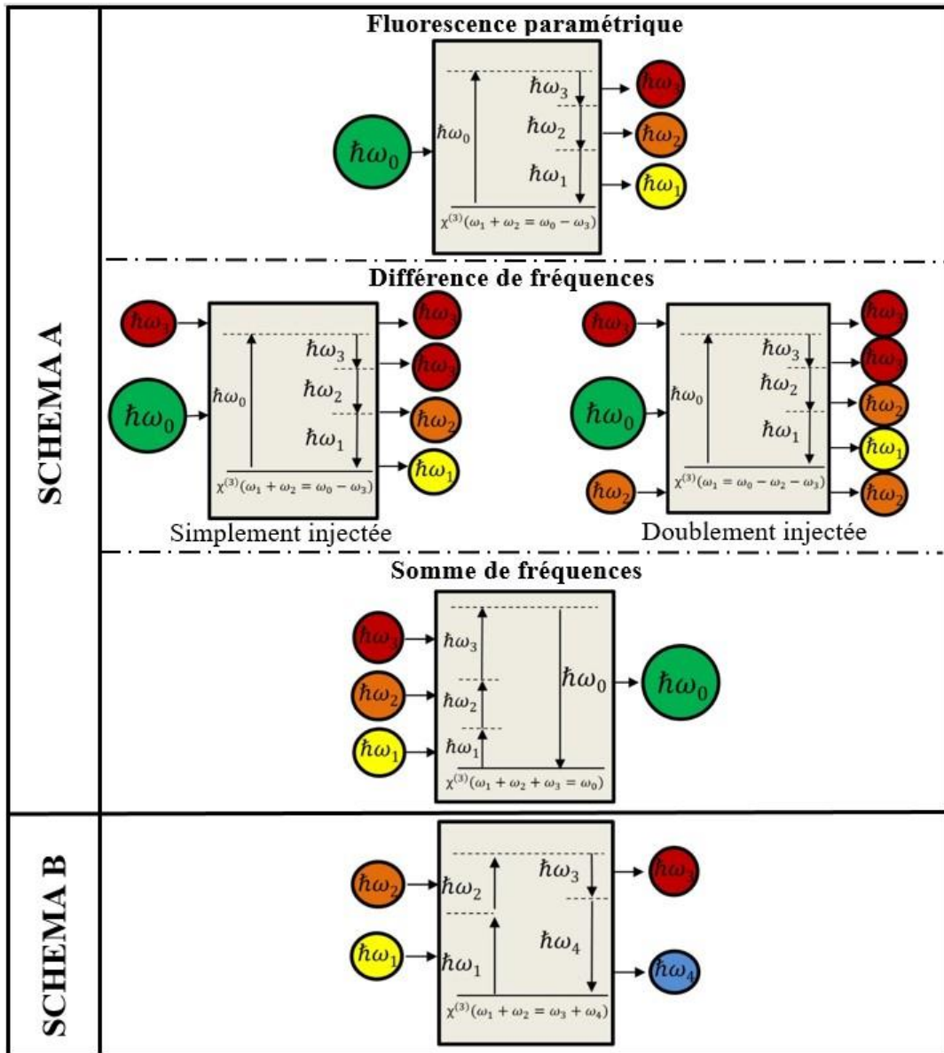
Figure I.11 : Diagrammes photoniques des différentes interactions optique non linéaires cubiques possibles. Le trait plein représente le niveau d'énergie fondamentale de la matière, les traits pointillés représentent les niveaux d'énergie du champ électro-magnétique [6].
