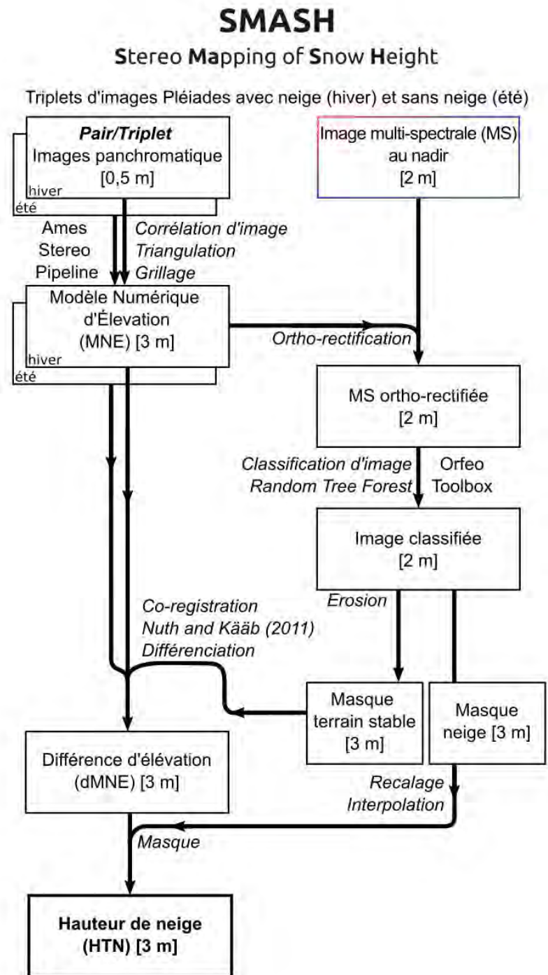
Figure 2.2 – La chaîne de production de cartes de hauteur de neige à partir d'images stéréo Pléiades (SMASH).
