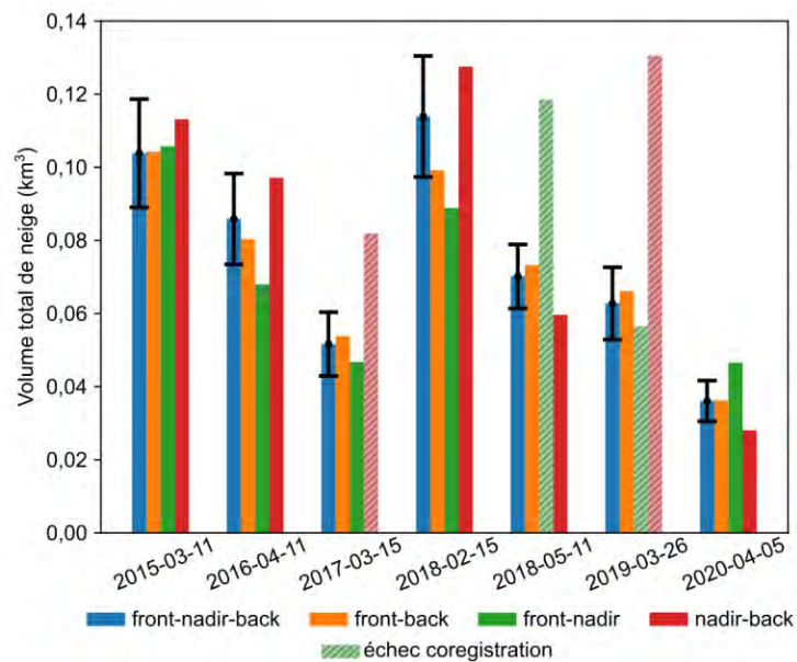
Figure 3.12 – Volume total de neige de la zone pour toutes les cartes de HTN (front-nadir-back en bleu, front-back en jaune, front-nadir en vert et nadir-back rouge). L’erreur est indiquée pour les données front-nadir-back (bleu) considérées comme référence. Elles sont également visibles dans la Figure 3.6. Les barres hachurées sont celles pour lesquelles l’étape de coregistration a échoué (voir en Annexe, Figure A.20).
