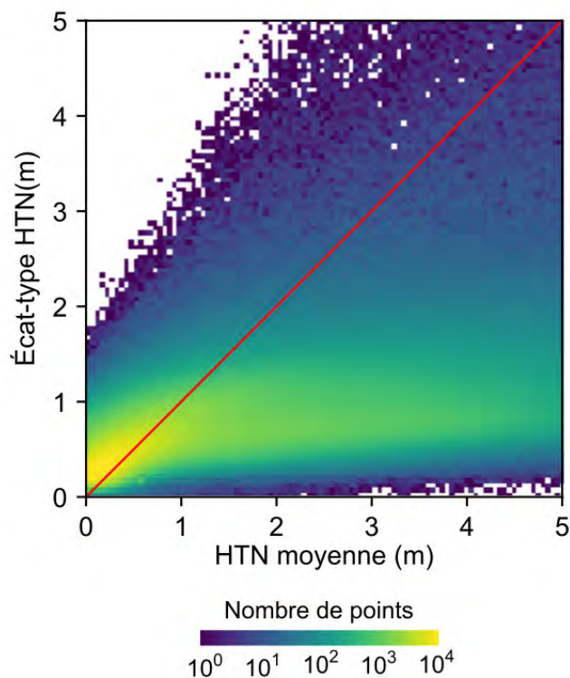
Figure 3.9 – Carte de chaleur de l'écart-type des HTN en fonction de la moyenne des HTN. L'échelle de couleur est logarithmique avec le plus de points dans les zones jaunes.
