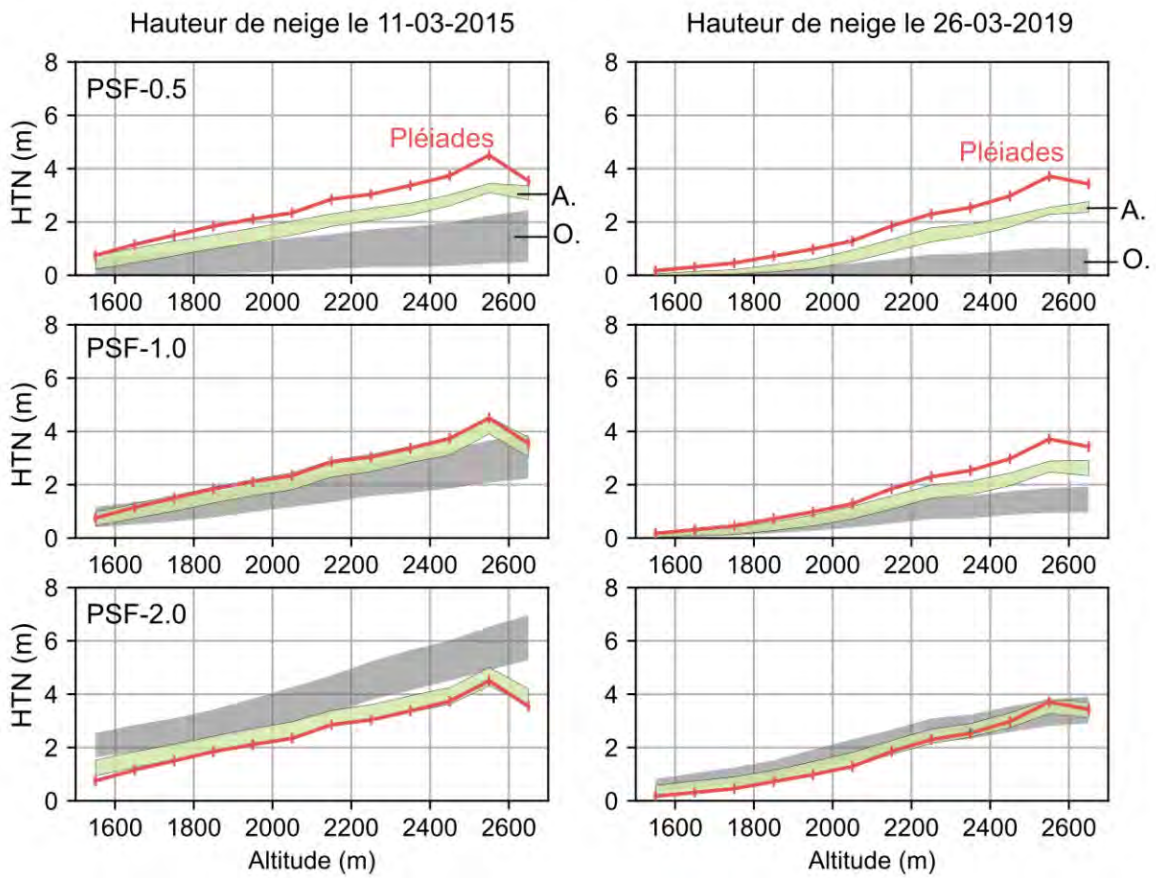
Figure 4.12 – HTN en fonction de l'altitude. L'enveloppe de l'open-loop (gris) et l'analyse (vert) montrent l'espace entre le 1 er et 3 ème quartiles. La HTN Pléiades (rouge) est la moyenne de la tranche d'altitude. Les barres représentent l'erreur assignée (voir 4.1.6.1).
