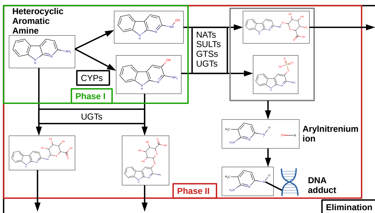
FIGURE 1.1 – Description du métabolisme des AHAs. L'activation métabolique des AHA se déroule en deux phases : une première phase d'oxydation nommée "phase I" (délimitée en vert), cette phase est principalement catalysée par les enzymes du métabolisme de phase I : les cytochromes P450 (CYPs). Le métabolite oxydé ainsi formé subit ensuite une réaction de conjugaison dite "phase II" (délimitée en rouge). Elle est catalysée par les enzymes de phase II que sont les UDP-glucuronyl transférases (UGTs), les N-acetyl transférases (NATs), les Sulfotransférases (SULTs) ou les Glutathion-S-transférase (GSTs) Le métabolite conjugué peut alors soit être excrété, c'est la phase III du métabolisme des xénobiotique (délimitée en noir). Dans certains cas le métabolite conjugué subit un clivage hétérolytique et forme un ion arylnitrenium qui est réactif vis-à-vis de l'ADN et peut conduire à la formation d'un adduit à l'ADN.
