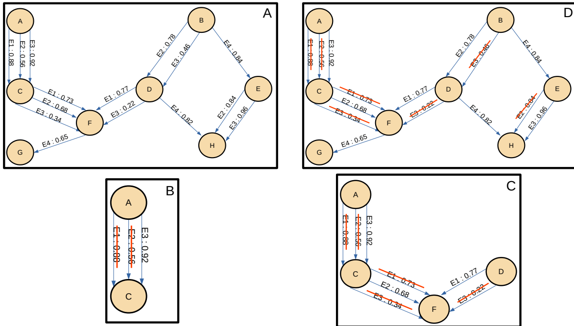
FIGURE 2.8 – Application des règles de réduction des cartes du métabolisme annotées en vue de construire un modèle Bayésien Cette figure montre la réduction d'une carte du métabolisme annotée (A) dont nous avons fait apparaître l'annotation de l'enzyme, ici E1, E2, E3 et E4, et du SOM score. La figure (B) illustre l'application de la première règle de réduction qui dit qu'une seule réaction peut consommer et produire les mêmes métabolites. Il y a une réaction consommant A et produisant C qui a été divisée en trois réactions, une pour chaque enzyme pouvant annoter la réaction. La réaction associée au score SOM le plus haut (0,68) a été sélectionnée. La figure (C) illustre l'application de la seconde règle de réduction qui concerne les réactions produisant le même métabolite mais consommant un métabolite différent. Dans cet exemple c'est le cas des réactions de C vers F et D vers F. Ici le score SOM maximal est 0,77 associé à une réaction de D vers F et annotée par l'enzyme E1. Cette réaction est retenue comme la seule réaction de D vers F, la réaction annotée par E3 de D vers F est éliminée. Ensuite les autres réactions annotées par E1 sont éliminées, ici c'est la réaction de C vers F annotée par E1 qui est éliminée. Il ne reste que deux réactions de C vers F, la première règle est appliquée et c'est la réaction annotée par E2 avec un score SOM de 0,68 qui est retenue. La figure (D) résume la réduction complète de la carte de la figure (A).
