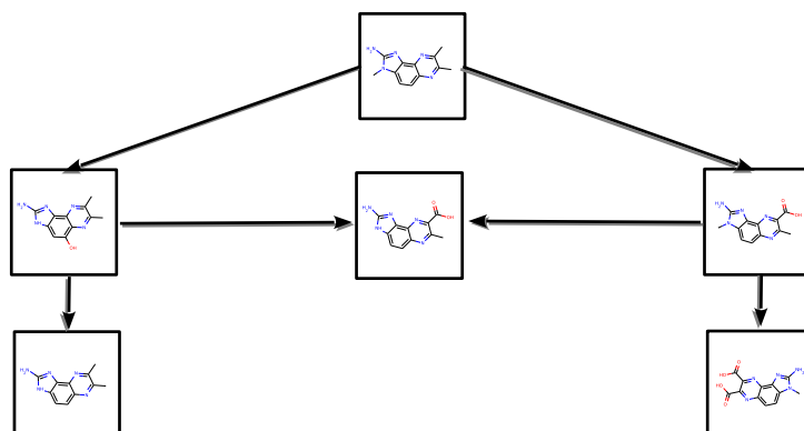
FIGURE 2.1 – Représentation d'une carte du métabolisme Celle-ci relie les différentes molécules, ou métabolites, par des réactions. Les métabolites sont représentés par leur structure 2D et sont encadrés. Les réactions sont représentées par des flèches.
