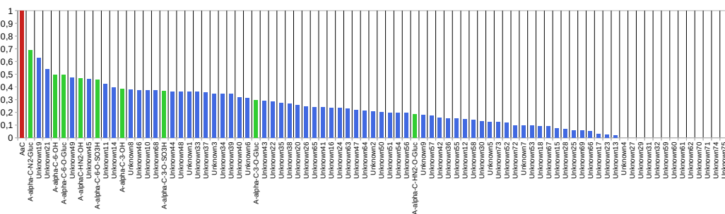
(a) Distribution du score de probabilités de production de chaque métabolite de la carte prédite du métabolisme d'AαC
