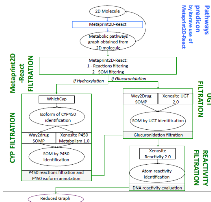
FIGURE 1.2 – Pipeline pour la prédiction des voies métaboliques des xénobiotiques et l’identification des métabolites réactifs à l’ADN Ce pipeline provient de la thèse à l’origine de l’étude Delannée et al. 2019 [20]. Il décrit un pipeline en deux parties permettant de générer des cartes du métabolisme des AHAs. La première partie est une étape de prédiction des métabolites en utilisant Metaprint2D-React (en bleu) comme outil de prédiction du métabolisme. Ensuite vient une partie de filtration des résultats de la première partie à partir de différents outils de prédictions de sites du métabolisme (en vert). Les prédictions sont également filtrées à travers les résultats de Xenosite Reactivity afin d’orienter la construction des cartes du métabolisme vers la formation d’adduits à l’ADN.
