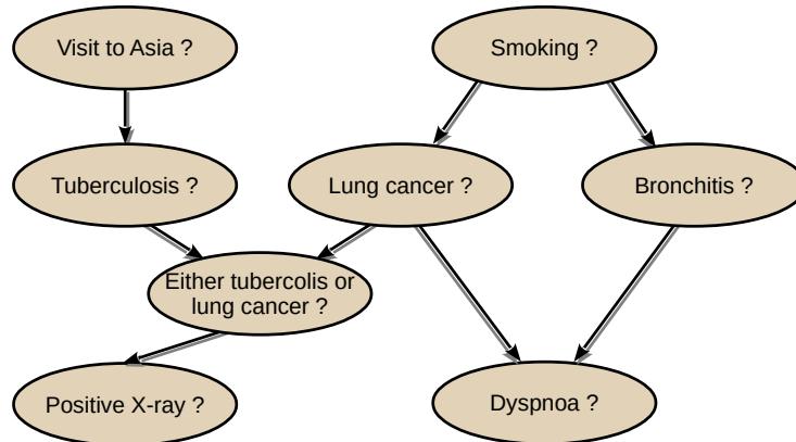
FIGURE 2.6 – Représentation du réseau bayésien Asia Ce réseau décrit des variables, représentées par des ovales, et les relations entre ces variables représentées par des flèches. Le réseau original a été proposé par Lauritzen et Spiegelhalter en 1988 [42] et décrit les influence de certaines variables sur d'autre dans un contexte de maladie pulmonaire.
