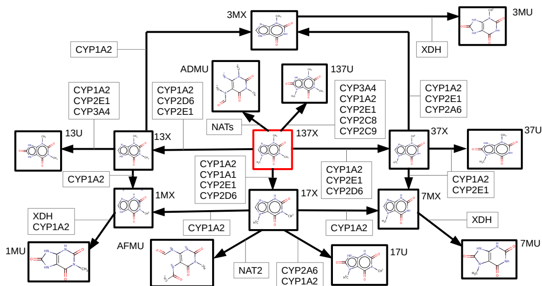
FIGURE 3.1 – Représentation schématique des connaissances sur le métabolisme de la caféine. Les enzymes catalysant les réactions sont représentées dans des cadres gris. XDH = xanthine déhydrogénase; NATs = N-acetyl transférases nous n'avons pas pu identifier dans la littérature la ou les isoformes associées à cette annotation. Nous faisons l'hypothèse qu'il s'agit de NAT2 car il s'agit d'une réaction similaire à celle générant AFMU
