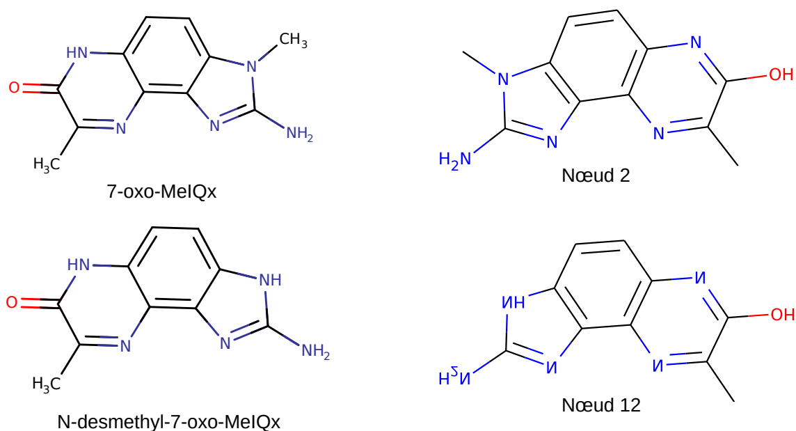
FIGURE 4.1 – Comparaison des structures chimiques des métabolites de MeIQx. Les métabolites expérimentalement identifiés de MeIQx sont décrits à gauche de la figure. Les métabolites de droite sont des métabolites provenant de la carte du métabolisme prédite, par SyGMa, de MeIQx.
