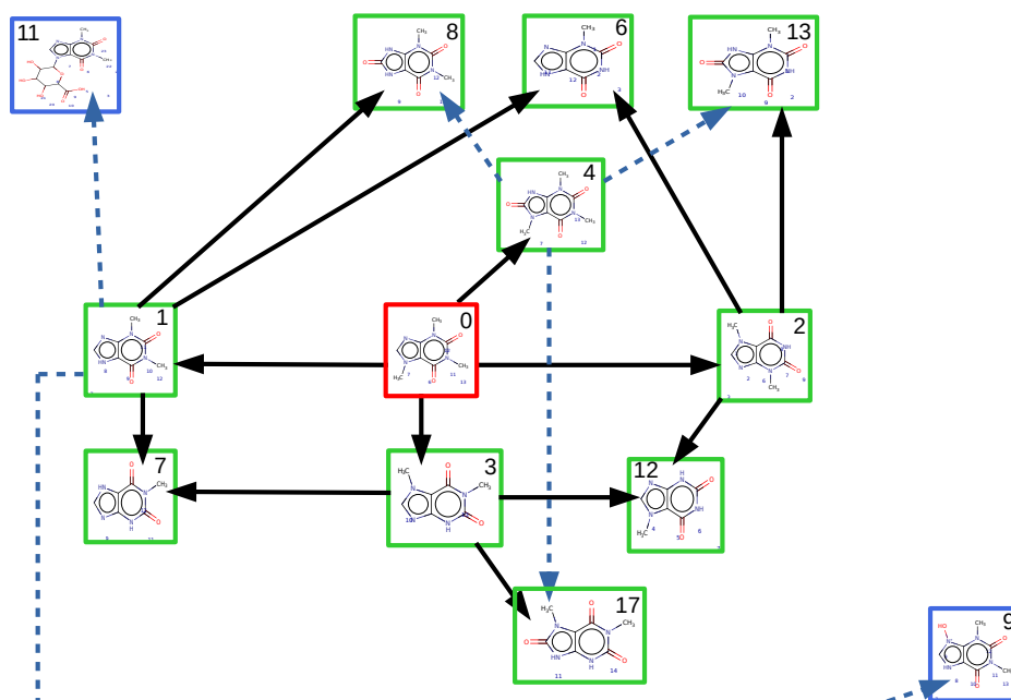
FIGURE 3.4 – Carte du métabolisme de la caféine prédite par SyGMA et filtrée à partir du score de probabilité de production. Cette carte est la carte obtenue après une filtration des métabolites de la carte précédente et cela afin de conserver uniquement les métabolites avec un fort score de probabilité de production. Le seuil de filtration utilisé est de 0,70 ce qui signifie que les métabolites associés à un score strictement inférieur sont éliminés. La carte contient 13 métabolites et 17 réactions. Deux métabolites, inconnus dans le métabolisme de la caféine, (noeuds 9 et 11), sont prédit comme ayant une probabilité de production proche des métabolites expérimentalement identifiés.
