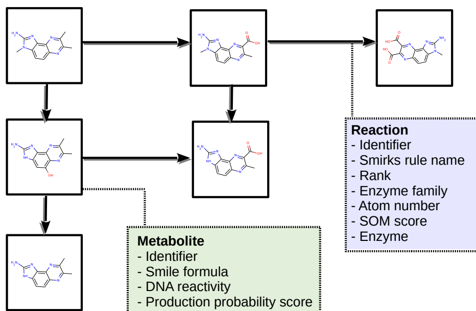
FIGURE 2.4 – Annotations des cartes du métabolisme. Les métabolites sont représentés par leur structure 2D dans des carrés noirs, ce sont les noeuds du graphe. Les flèches représentent les arêtes dirigées et donc les réactions. Les rectangles de couleur listent les annotations des métabolites (vert) et les annotations des réactions (violet).
