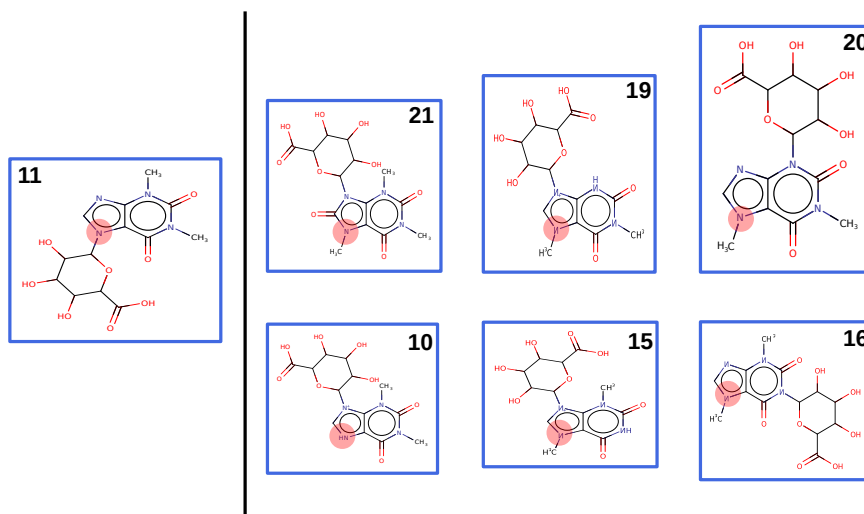
FIGURE 3.5 – Comparaison de la structure chimique des métabolites inconnus de la caféine issus de glucuronidation. À gauche le métabolite du noeud 11 qui est conservé après la filtration et à droite les métabolites éliminés par la filtration. Chaque métabolite est identifié par le numéro du noeud auquel il est associé. La zone rouge marque l'azote auquel le groupe glucuronyl est associé dans le métabolite 11.
