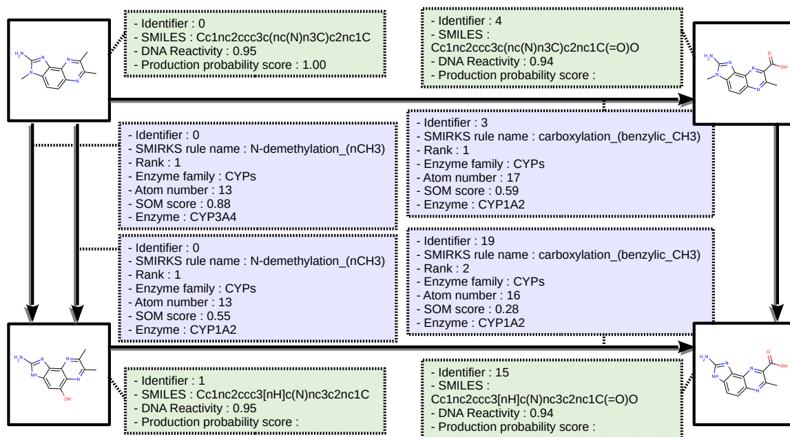
FIGURE 2.5 – Exemple d’une carte du métabolisme annotée. Cet exemple de carte du métabolisme annotée est un extrait de la carte de la figure 2.4, elle reprend les mêmes codes et donne des exemples concrets des valeurs que peuvent prendre les annotations.
