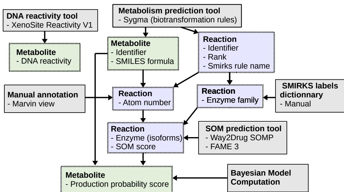
FIGURE 2.3 – Pipeline de production des annotations des métabolites et des réactions. Les annotations sont décrites dans les cadres verts (métabolites) et violets (réactions). Ces annotations sont obtenues par différents outils et procédés qui sont représentés par les cadres gris. Le "SMIRKS labels dictionary" est détaillé dans l'Annexe 2.
