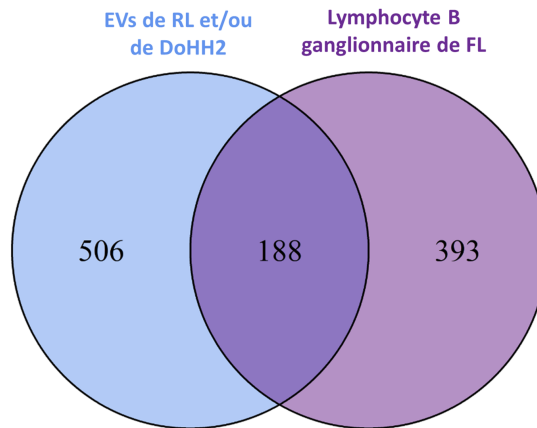
FIGURE 5.5 – Expression des miRNAs dans les EVs de lignées B RL et/ou DOHH2 et les B ganglionnaires de FL.
