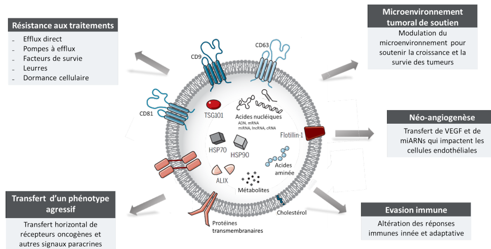
FIGURE 1.12 – Les EVs dérivées de tumeurs influencent de nombreux aspects de la cancérogénèse. Par leur capacité à transférer certaines molécules bioactives et à propager le transfert horizontal de protéines et d'acides nucléiques de multiples natures, les vésicules extracellulaires dérivées de tumeurs peuvent affecter une variété d'événements cellulaires et avoir un impact sur la progression tumorale. Illustration librement adaptée de KALLURI et LEBLEU [141].
