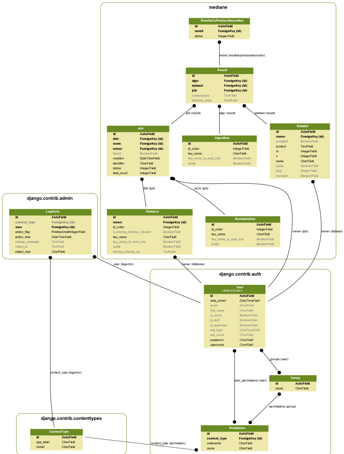
FIGURE 4.1 – Base de données de l'outil CoRankCo
