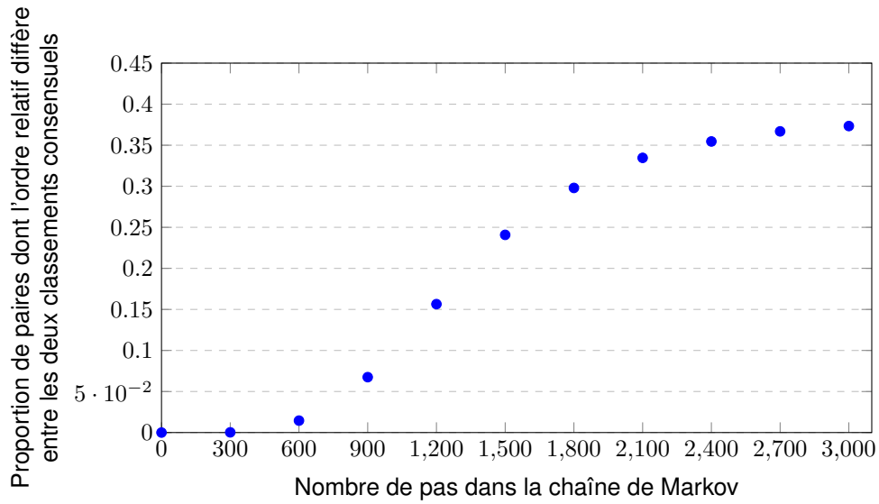
FIGURE 4.5 — Proportion moyenne (sur les jeux de données du Dataset 4) de paires dont l'ordre relatif est différent entre les deux classements consensuels obtenus à partir de deux KCFs différentes en fonction du nombre de pas dans la chaîne de Markov.
