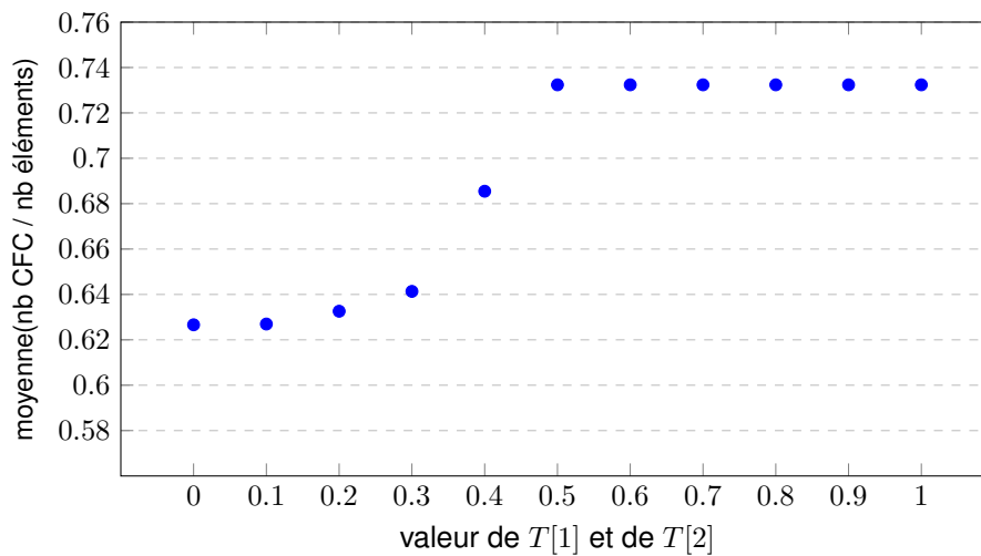
FIGURE 4.7 – Influence de T[1] et T[2] sur la capacité à partitionner le problème initial en sous-problèmes : moyenne sur l'ensemble des jeux de données du Dataset 1 du nombre de sous-problèmes obtenus par l'algorithme ParCons divisé par le nombre d'éléments en fonction de T[1] = T[2] .
