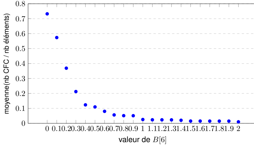
FIGURE 4.6 – Influence de B[6] sur la capacité à partitionner le problème initial en sous-problèmes : moyenne sur l’ensemble des jeux de données du Dataset 1 du nombre de sous-problèmes obtenus par l’algorithme ParCons divisé par le nombre d’éléments en fonction de B[6] .
