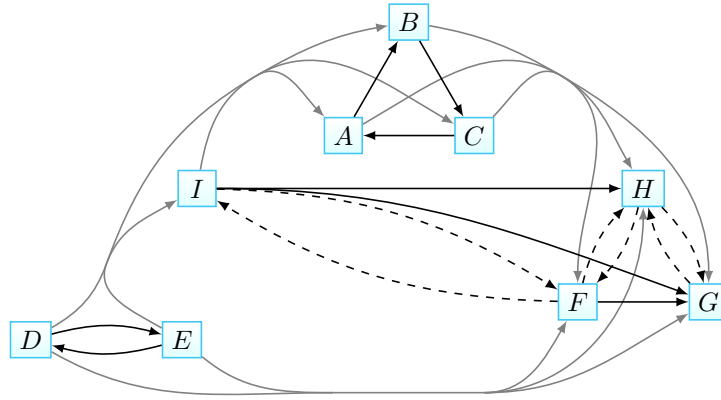
FIGURE 3.3 – Graphe robuste des éléments G_r pour l'exemple de la Table 3.1. Les arcs gris avec sources/cibles multiples indiquent la présence d'un arc de chaque sommet de chaque source vers chaque sommet de chaque cible (par exemple, il y a un arc depuis chaque sommet de (D, E) vers chaque autre sommet). Les arcs en pointillés représentent les arcs de G_r qui ne sont pas présents dans G_e .
