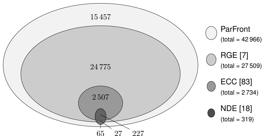
FIGURE 3.11 – Diagramme de Venn indiquant le nombre de frontières obtenues par chacune des quatre méthodes suivantes : NDE (éléments propres, Betzler et al. [18]), critère de Condorcet étendu Truchon [83], RGE ( graphe robuste des éléments , [7]) et ParFront.
