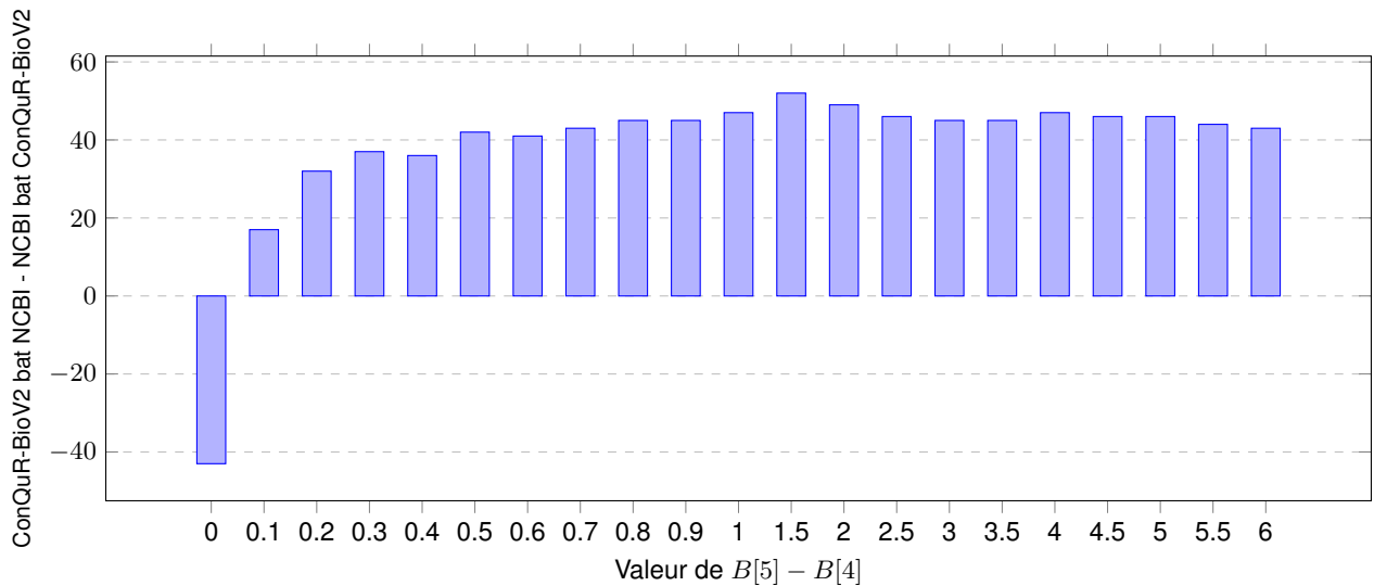
FIGURE 4.3 – Nombre de jeux de données du Dataset 2 tels que ConQuR-BioV2 bat le NCBI moins le nombre de jeux de données tels que le NCBI bat ConQuR-BioV2 en fonction de la valeur de B[5] - B[4] .
