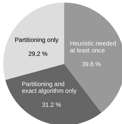
FIGURE 3.9 – Proportion de jeux de données telle que le partitionnement a été utilisé seul (classement consensuel optimal), le partitionnement et un algorithme exact ont été utilisés, sans heuristique (classement consensuel optimal), une heuristique était nécessaire pour au moins un sous-problème (classement consensuel éventuellement non optimal).
