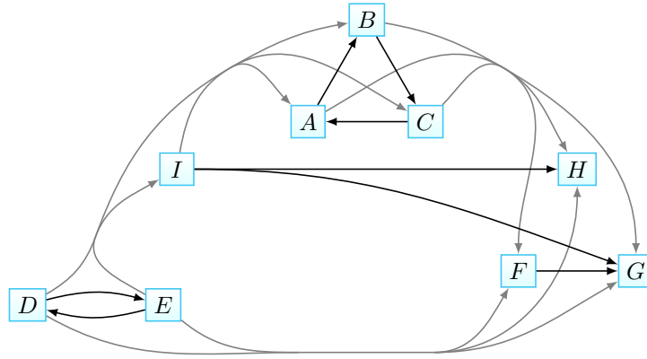
FIGURE 3.1 – Graphe des éléments G_e pour l'exemple de la Table 3.1. Les arcs gris avec sources/cibles multiples indiquent la présence d'un arc de chaque sommet de chaque source vers chaque sommet de chaque cible (par exemple, il y a un arc depuis chaque sommet de (D, E) vers chaque autre sommet, mais il n'y a pas d'arc de I à F ).
