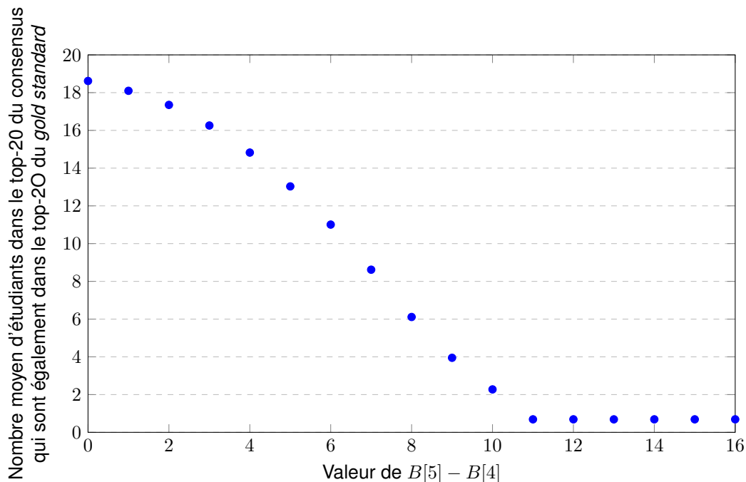
FIGURE 4.4 – Nombre moyen (sur les jeux de données du Dataset 3) d'étudiants dans le top-20 du classement consensuel qui sont également dans le top-20 du classement obtenu en considérant la moyenne générale en fonction de la valeur B[5] - B[4] .
