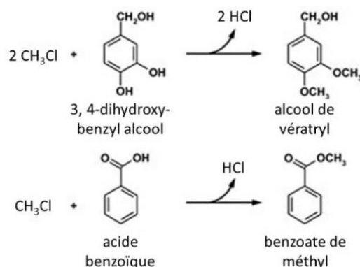
Figure 1.8. Réactions de dégradation du chlorométhane par les champignons
