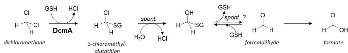
Figure 1.12. Dégradation du dichlorométhane par la voie hydrolytique de la glutathione S-transférase
