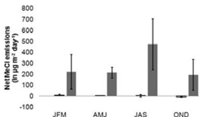
Figure 1.9. Flux du chlorométhane dans un sol forestier en fonction des saisons
