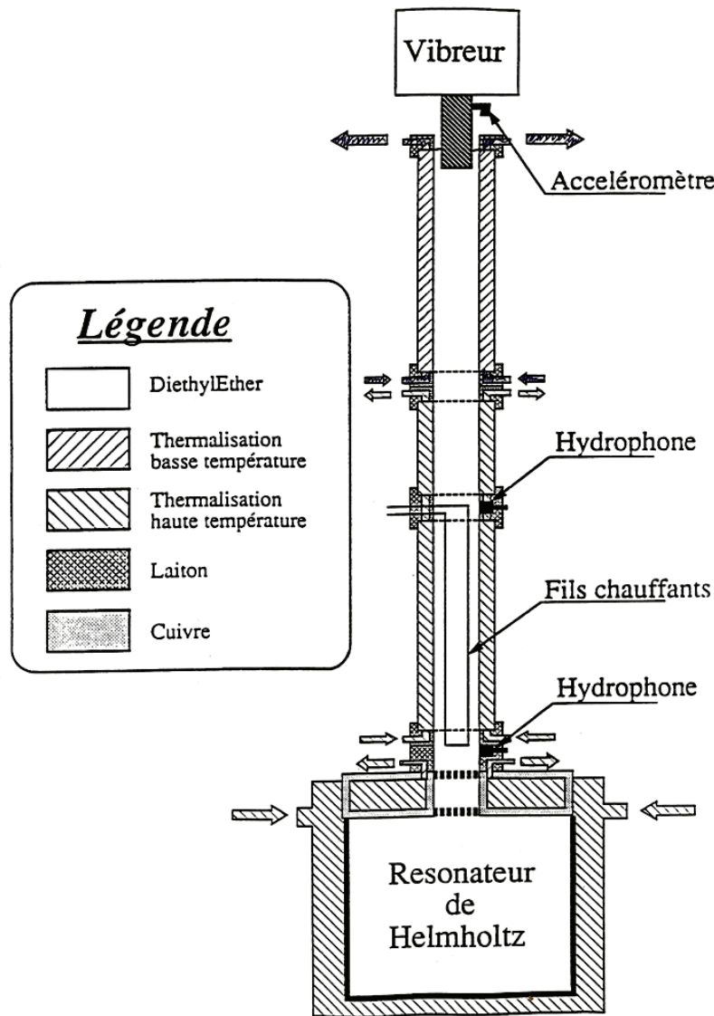
Figure 50 : Le dispositif expérimental basé sur un résonateur de Helmholtz de Coste [Cos91]
