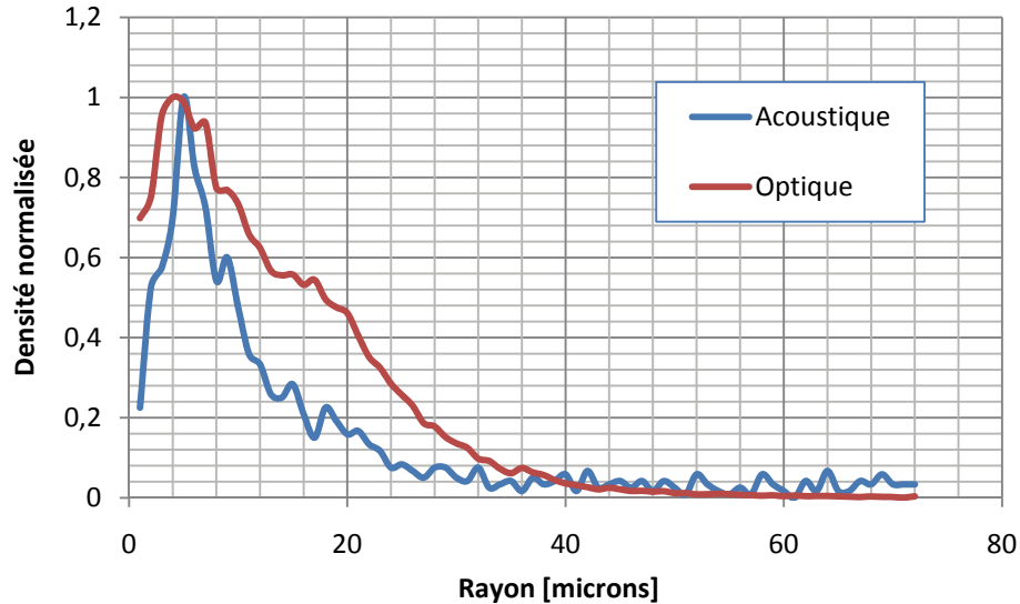
Figure 73 : Autre reconstruction d'histogrammes optique et acoustique par mixage HF-BF
