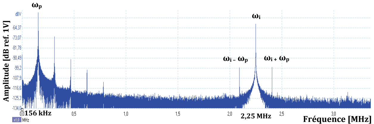
Figure 70 : Exemple de spectre acoustique permettant la reconstruction de l'histogramme des rayons des bulles
