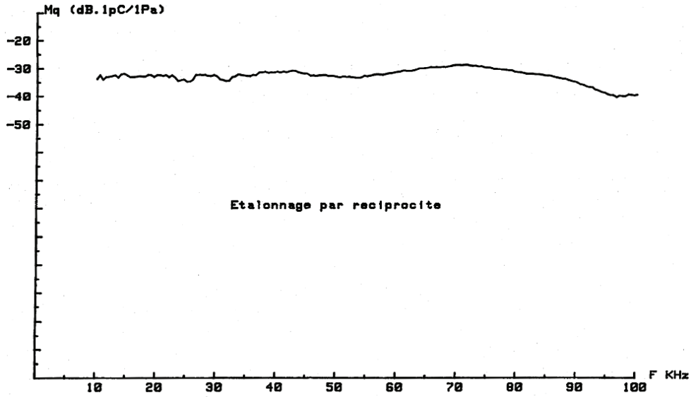
Figure 81 : Sensibilité BF d'un TUSHT en charge en sodium à 545°C [Lhu84-2]
