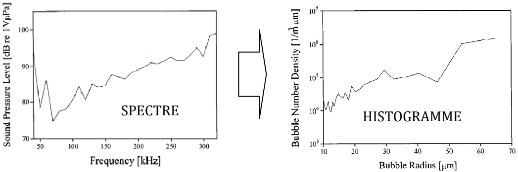
Figure 44 : Histogrammes des rayons reconstruits à partir des fréquences différence mesurées et de leur intensité par [Sut98]
