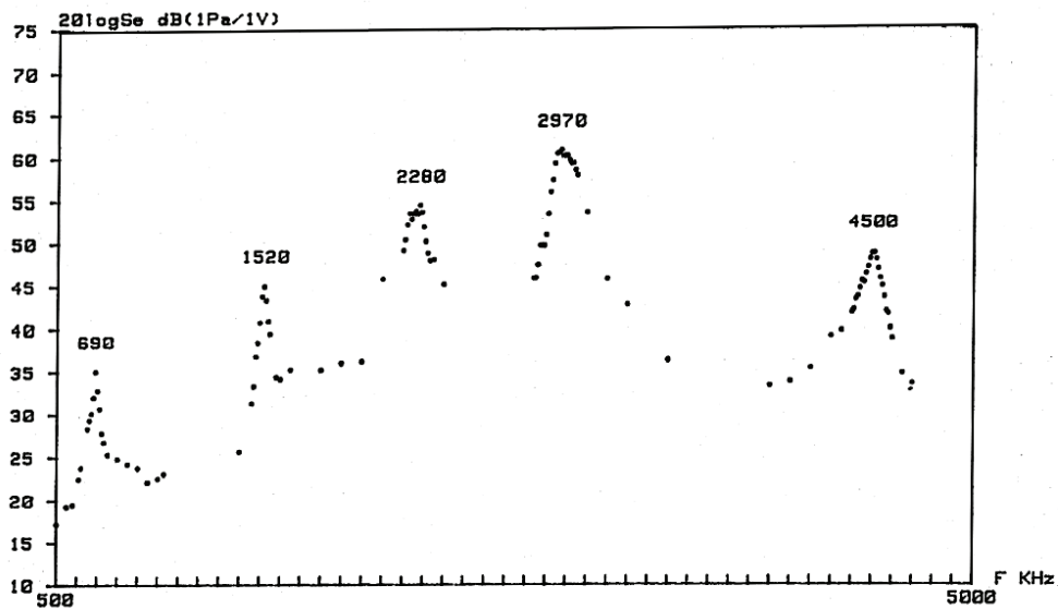
Figure 82 : Efficacité HF en tension d'un TUSHT à 1 m en eau à 20°C [Lhu84-2]
