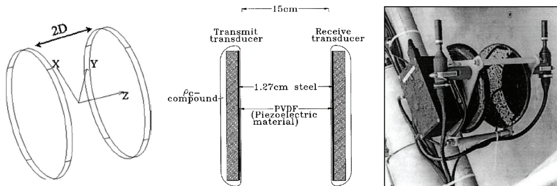
Figure 86 : Le résonateur amélioré de [Far98 - Far05]
