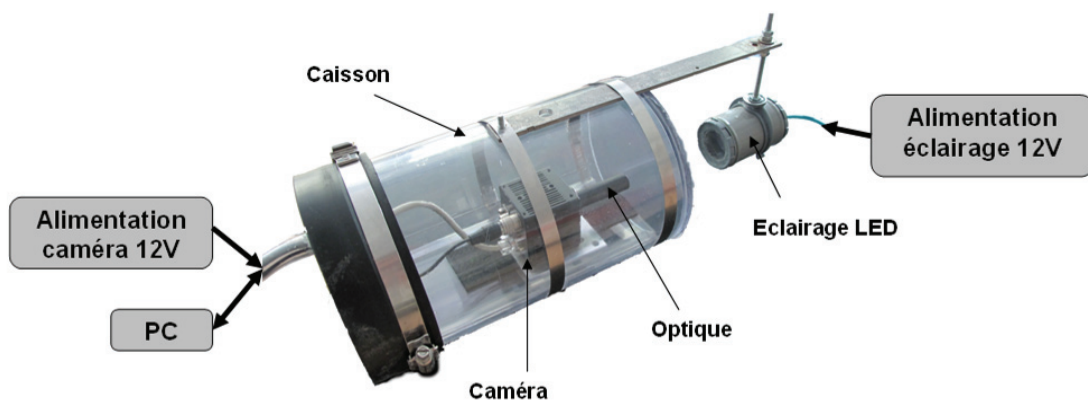
Figure 55 : Vue générale du dispositif optique
