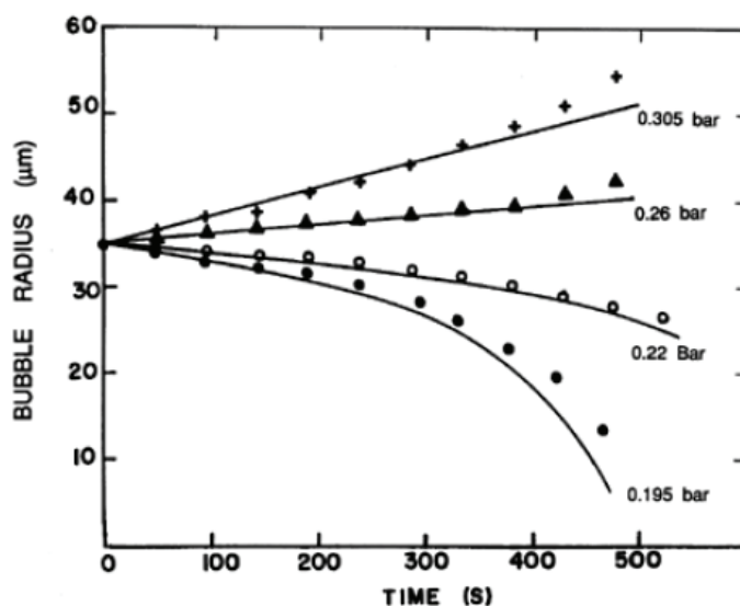
Figure 18 : Dissolution de bulles et croissance par diffusion rectifiée [Cru80]
