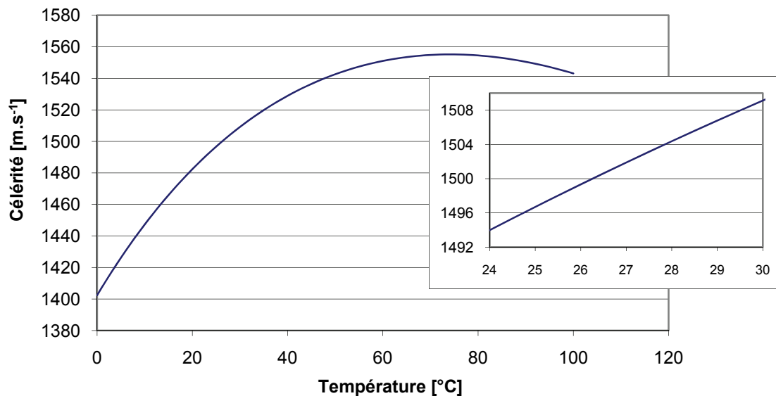
Figure 93 : L'équation de Marczak : la célérité dans l'eau en fonction de la température de 0°C à 100°C (et zoom entre 24°C et 30°C)
