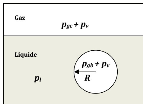
Figure 8 : Equilibre d'une bulle dans un liquide saturé : pressions en jeu
