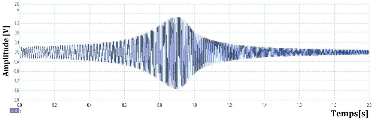
Figure 105 : Signal temporel de la résonance sans bulles
