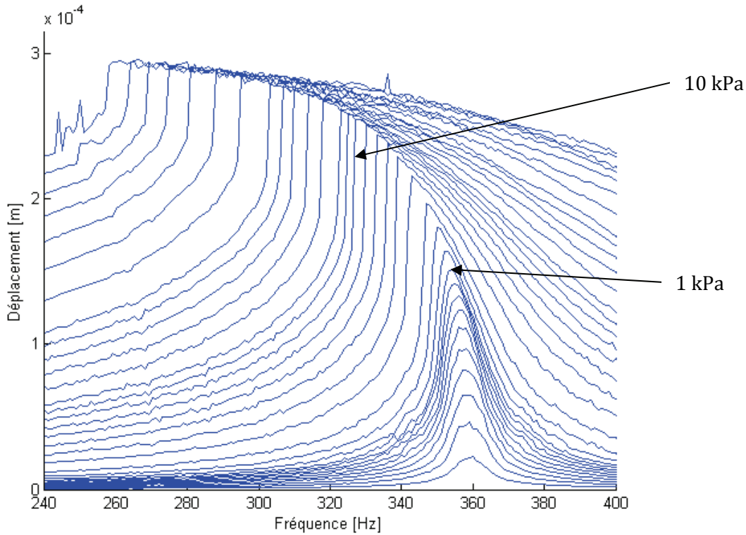
Figure 119 : Zoom sur la résonance principale présentée Figure 118
