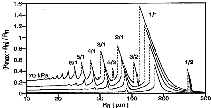
Figure 48 : Courbes de résonances d'une bulle insonifiée à 20 kHz, pour des amplitudes de pression acoustique de 10, 30, 50 et 70 kPa [Lau99]
