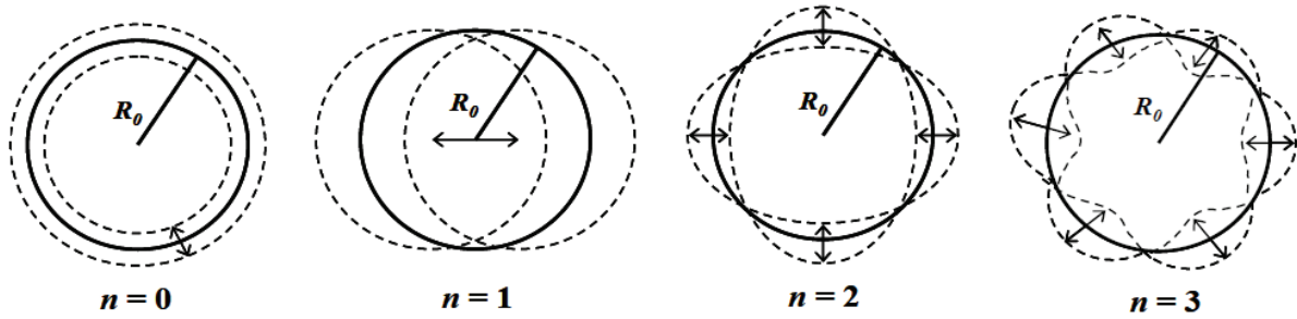
Figure 24 : Les modes de vibration 0, 1, 2, 3 des bulles sphériques [Dur09]
