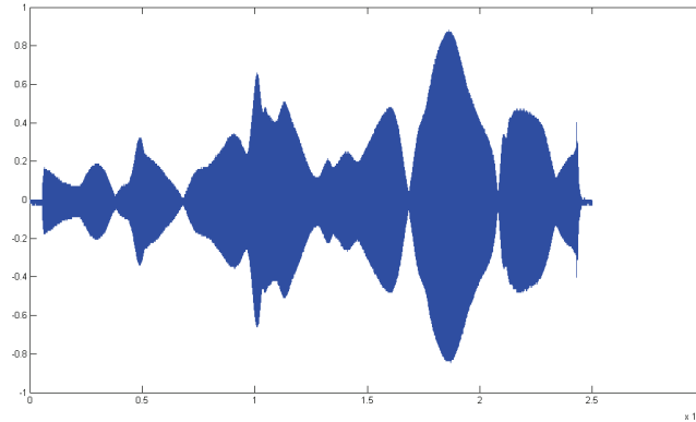
Figure 90 : Signal temporel en l'absence de bulles
