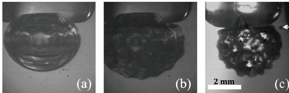
Figure 127 : Photographies de l'excitation d'une bulle de 2,1 mm de rayon moyen à 1,506 kHz et des pressions acoustiques de 24 Pa (a), 44 Pa (b) et 139 Pa (c) [Mak08-2]
