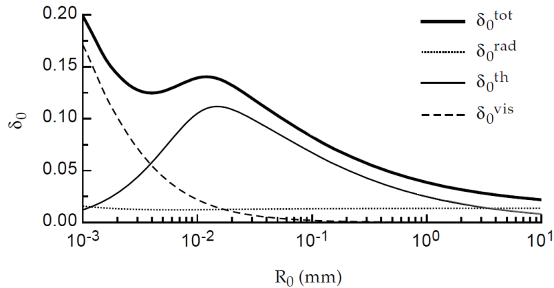
Figure 15 : Les différentes composantes de la constante d'amortissement à la résonance en fonction du rayon de la bulle (air-eau) [Ler04]
