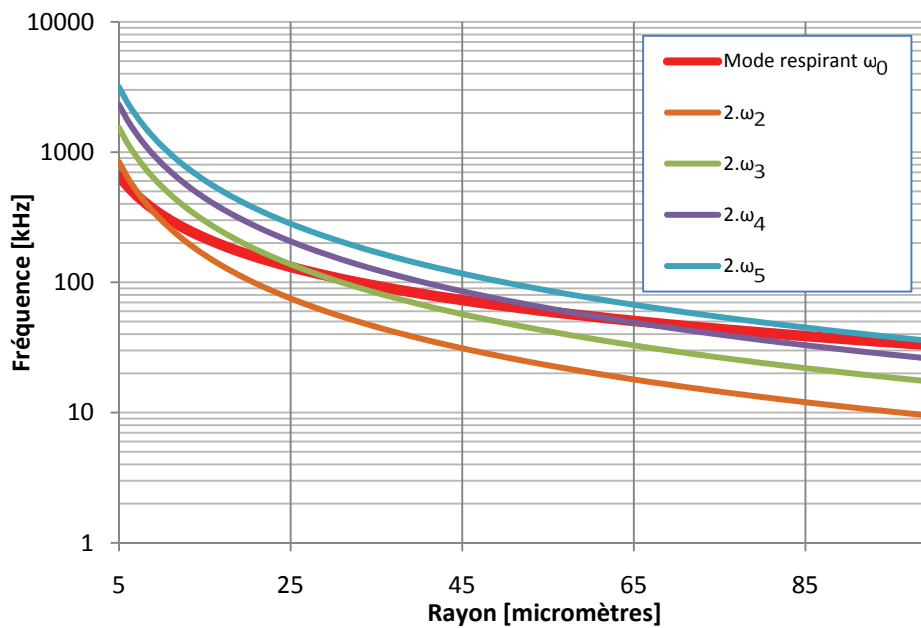
Figure 125 : Tracé de la fréquence de résonance fondamentale et du double des quatre premiers modes de distorsion de la bulle en fonction de son rayon
