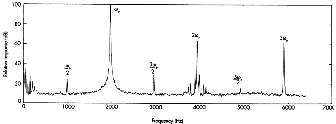
Figure 31 : Spectre des harmoniques, ultraharmoniques et subharmonique d'une bulle résonnante à 2 kHz [Lei94]
