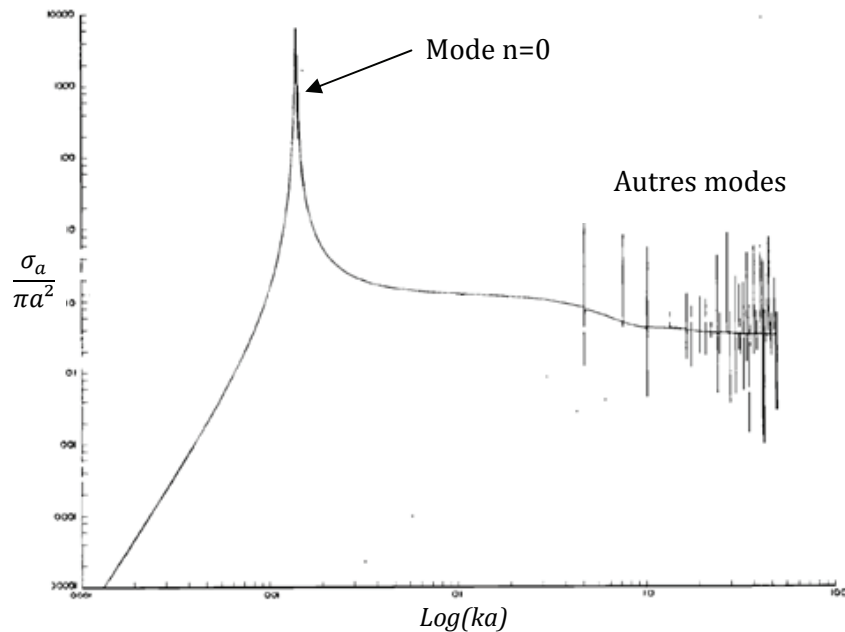
Figure 25 : Section de diffusion \sigma_a d'une bulle d'air dans l'eau, en fonction de la fréquence réduite [Sag79]
