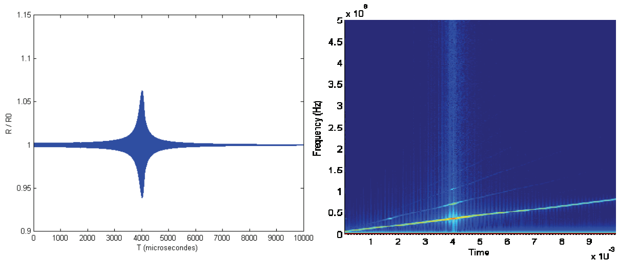
Figure 112 : Simulation du modèle de Keller-Miksis. Bulle de 10 \mu\text{m} de rayon, amplitude de 1 kPa. Evolution temporelle du rayon (à gauche) et spectrogramme (à droite).
