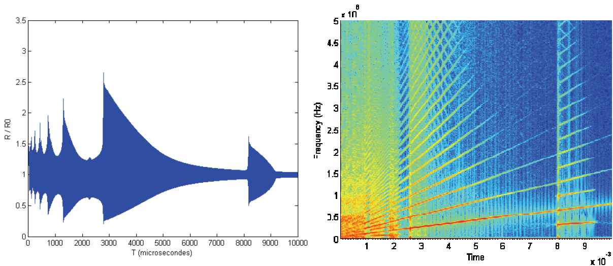
Figure 115 : Simulation du modèle de Keller-Miksis. Bulle de 10 \mu\text{m} de rayon, amplitude de 80 kPa. Evolution temporelle du rayon (à gauche) et spectrogramme (à droite).
