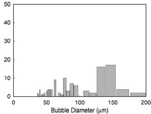
Figure 40 : Histogramme des rayons des bulles reconstruit grâce au mixage non linéaire de deux fréquences [Buc05]
