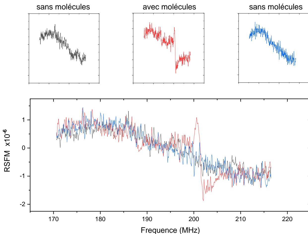
FIGURE 37 Représentation d'une succession de 3 scans. Le second est fait avec 150 mTorr dans la cellule de réflexion sélective et les deux autres sont faits sans molécule dans la cellule. L'échelle de fréquence ici n'a pas été corrigée en utilisant le lambdamètre.
