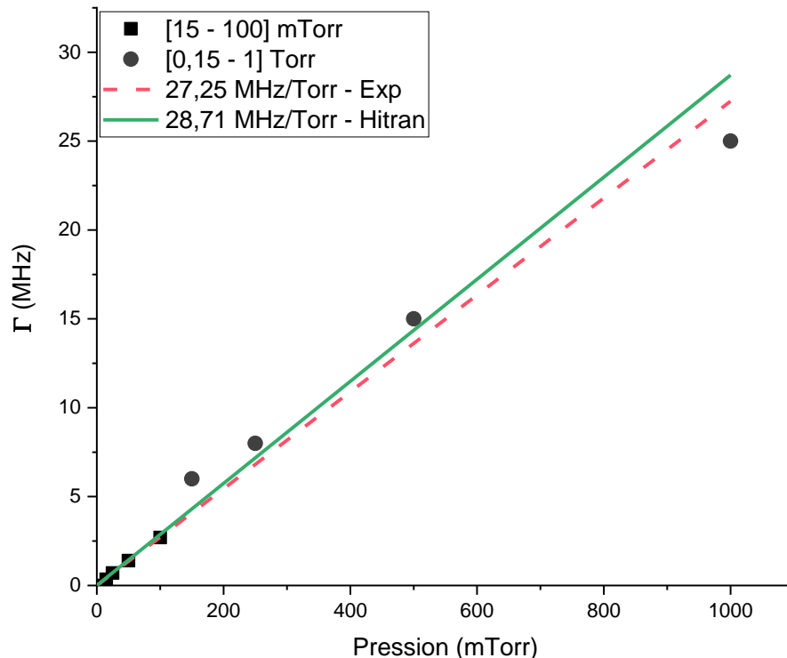
FIGURE 30 Estimation de l'élargissement par pression de la transition sP(1,0) du NH_3 pour les deux gammes de pression étudiées. Dans la première gamme [0.15 – 1]Torr , on a une résolution limitée par la largeur collisionnelle et dans la deuxième gamme [15 – 100]mTorr la largeur collisionnelle est similaire à la largeur du laser et à l'excursion de la modulation FM. On a représenté une fonction linéaire qui traduit l'évolution de l'élargissement par pression que l'on estime à 27.25 MHz/Torr qui est similaire à celle que l'on trouve dans Hitran et dans [21].
