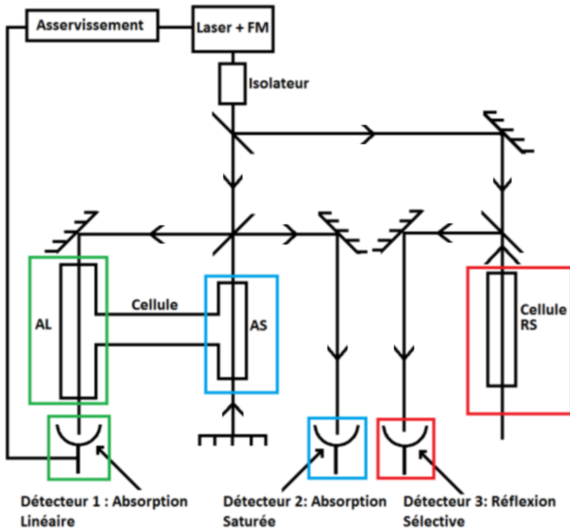
FIGURE 7 Montage expérimental de réflexion sélective sur des transitions rovibrationnelles moléculaires. Le faisceau du laser (QCL) à 10,6\mu\text{m} traverse un isolateur optique pour éviter un retour sur le laser et ensuite, à l'aide de lames séparatrices, il est divisé en trois montages différents : Le montage principal de réflexion sélective, afin de sonder les molécules près de la surface, un montage auxiliaire d'absorption saturée qui nous permet d'identifier les fréquences des transitions moléculaires en volume et un montage auxiliaire d'absorption linéaire qui nous permet principalement d'asservir le laser afin de réduire sa dérive en fréquence pendant le balayage.
