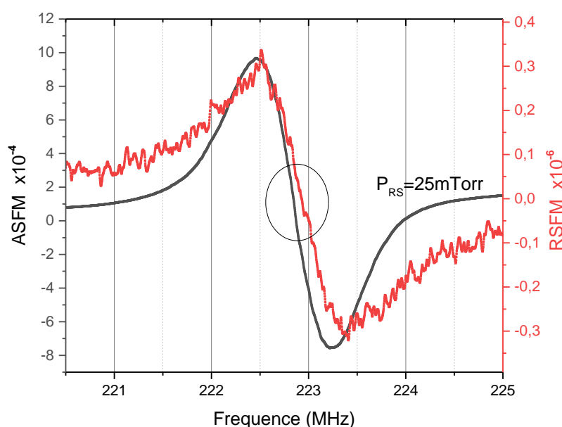
FIGURE 41 Spectres de réflexion sélective et d'absorption saturée dans les mêmes conditions de pression. Accumulation et moyenne sur 80 scans de réflexion sélective. On remarque que le zéro sur le spectre de réflexion sélective ne se superpose pas avec celui de l'absorption saturée.
