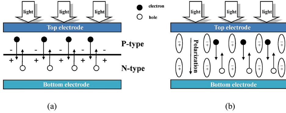
FIGURE 8.2 : Illustration d'un principe de fonctionnement d'un semi-conducteur classique à bande interdite unique. Cellule de type p-n (a) et celle basée sur FE (b). Image de la réf. [4].
