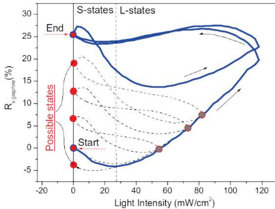
FIGURE 8.10 : Balayages d'intensité lumineuse qui démontrent l'existence de plusieurs états écrits par la lumière (en fonction de l'intensité lumineuse maximale).
