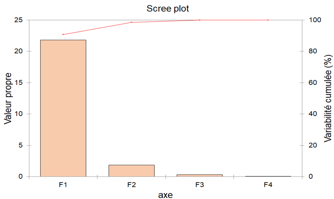
Figure 35. Scree plot des valeurs propres à partir de l'ACP
