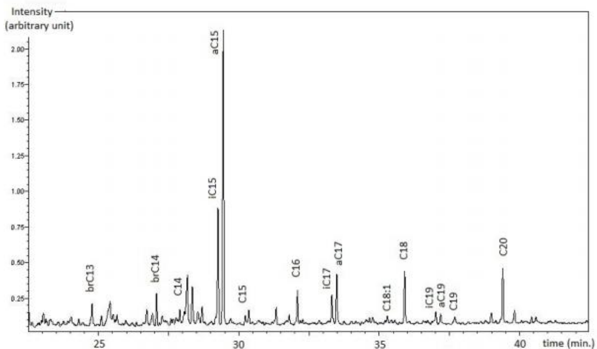
Figure 30. Pyrogramme (TMAH, 600 °C) de la souche Staphylococcus aureus résistante à la Méricilline (SARM)
