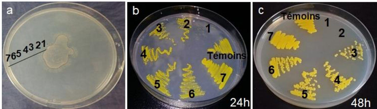
Figure 21. Implication des substances diffusibles au cours de la prédation
