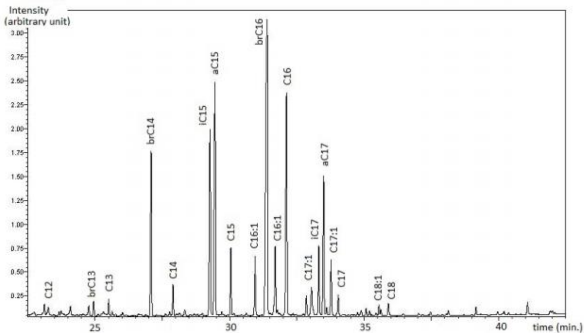
Figure 31. Pyrogramme (TMAH, 600 °C) de l'actinobactérie prédatrice Streptomyces griseoflavus EMM111
