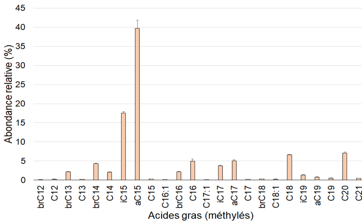
Figure 32. Abondance relative (%) des acides gras (méthylés) dans la souche Staphylococcus aureus résistante à la Mécicilline (SARM)
