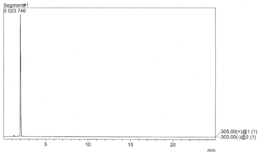
Figure 52. Chromatogramme (SIM 303 et 305) obtenu par couplage LCMS de la fraction FC9b3
