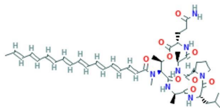
DKxanthene-534 C 29 H 34 N 4 O 6
