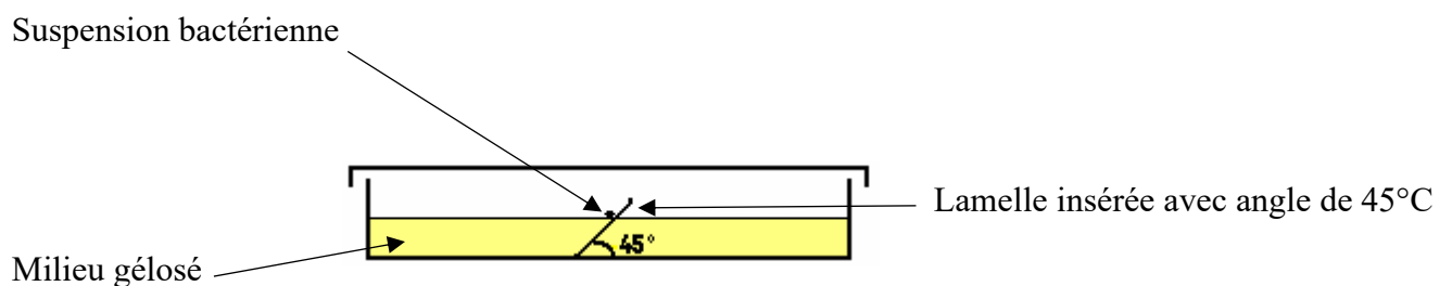
Figure 23. Schéma présentant la culture sur lamelle (Ouchari, 2019)
