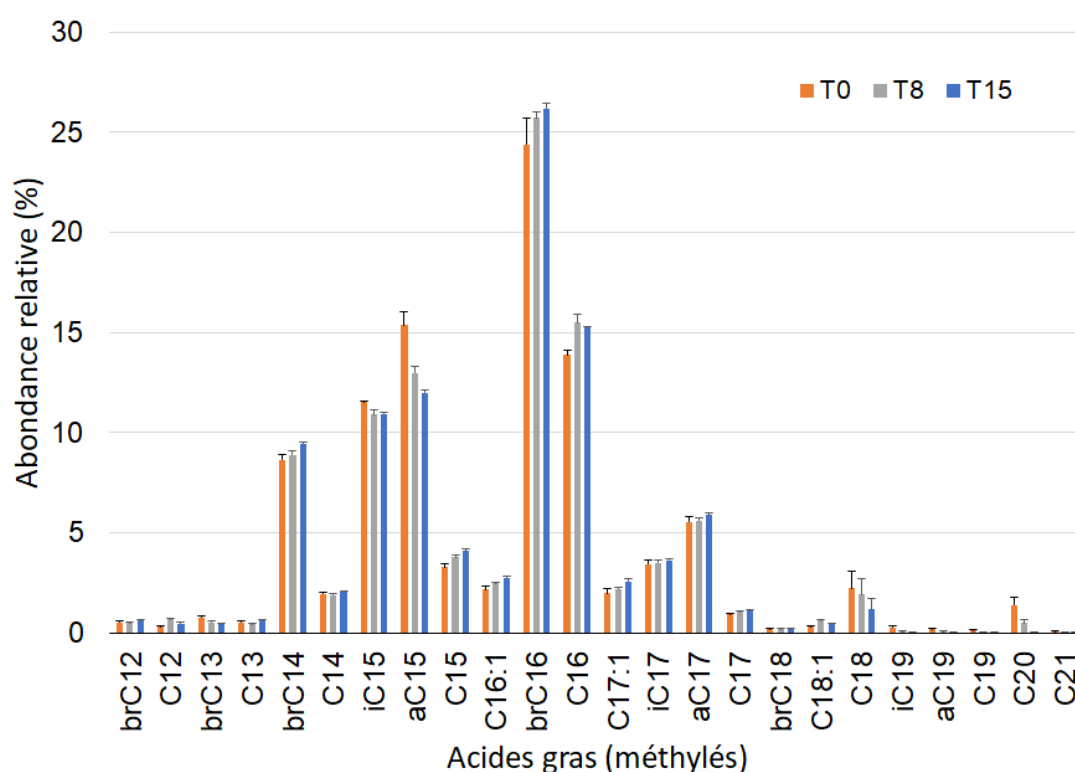
Figure 34. Abondance relative (%) des acides gras (méthylés) au cours de la co-culture (T0, T8 et T15)
