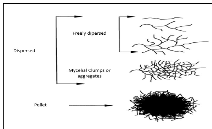
Figure 4. Morphologie des hyphes en croissance dans le milieu liquide (Alonso, 2007)
