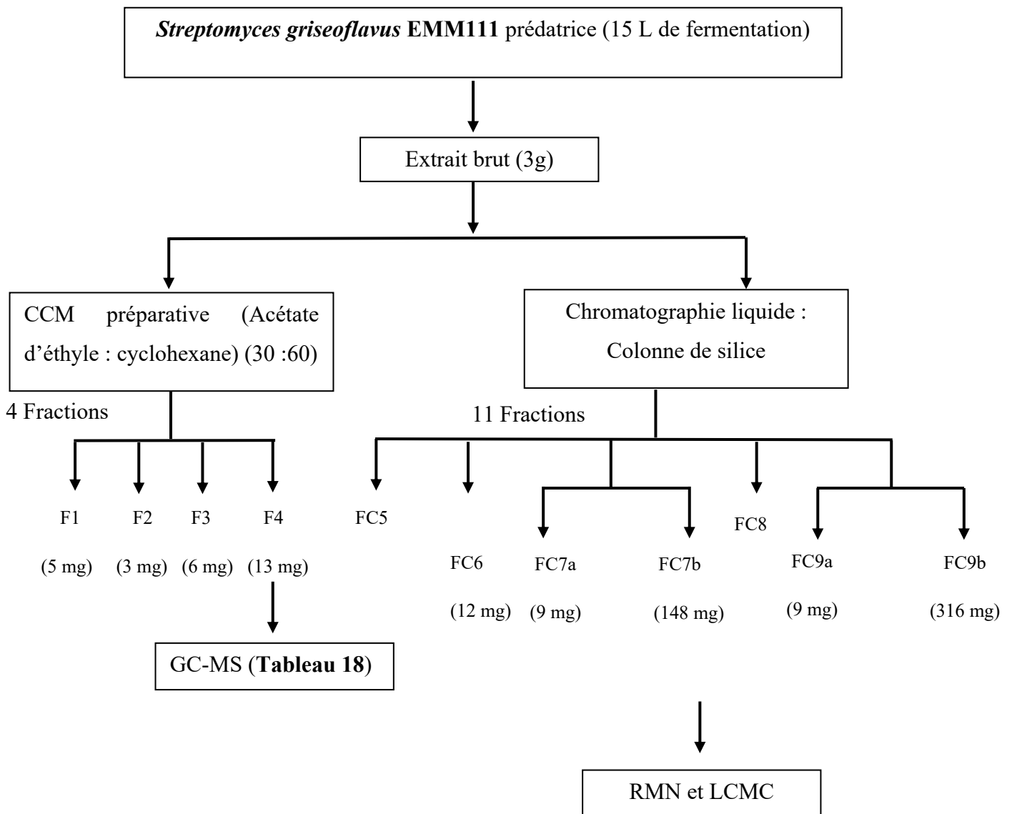
Figure 44. Protocole de séparation des fractions bio actives
