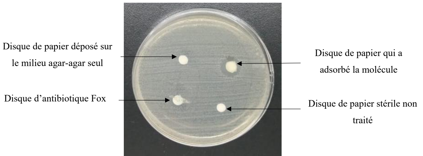
Figure 22. Activité antibactérienne de l'isolat EMM111 contre la souche Staphylococcus aureus résistante à la méticilline
