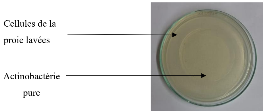
Figure 12. Etude du spectre de l'activité de prédation
