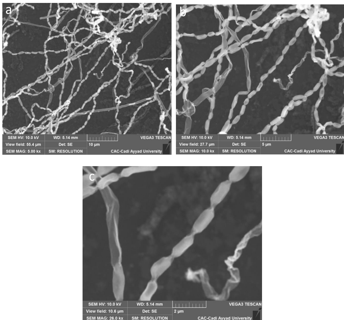
Figure 29. Observation des spores, du mycélium aérien et du substrat de l'isolat EMM194 (a \times 5000, b \times 10000, c \times 26,000)
