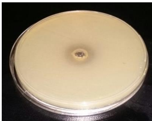
Figure 43. Activité antibactérienne de l'extrait de la souche S. griseoflavus EMM111 par l'acétate d'éthyle vis-à-vis SARM par la technique des puits
