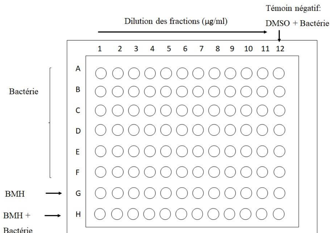
Figure 39. Schéma de la technique de micro-dilution.
