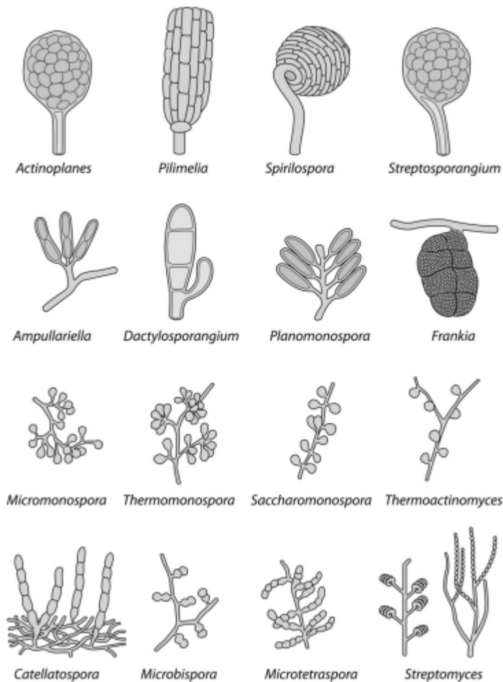
Figure 9. Différentes chaînes de spores chez les actinobactéries (Ait Barka et al., 2016)
