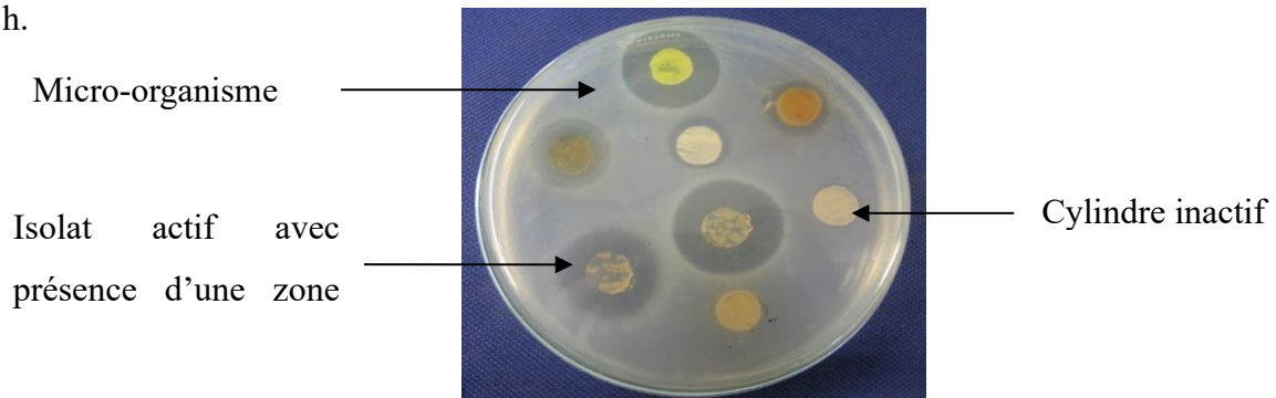
Figure 13. Mise en évidence de l'activité antibactérienne en milieu solide par le test des cylindres d'agar
