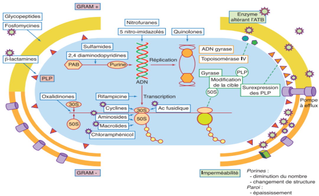
Figure 2. Mode d'action des antibiotiques (Chaussade et al. , 2013)
