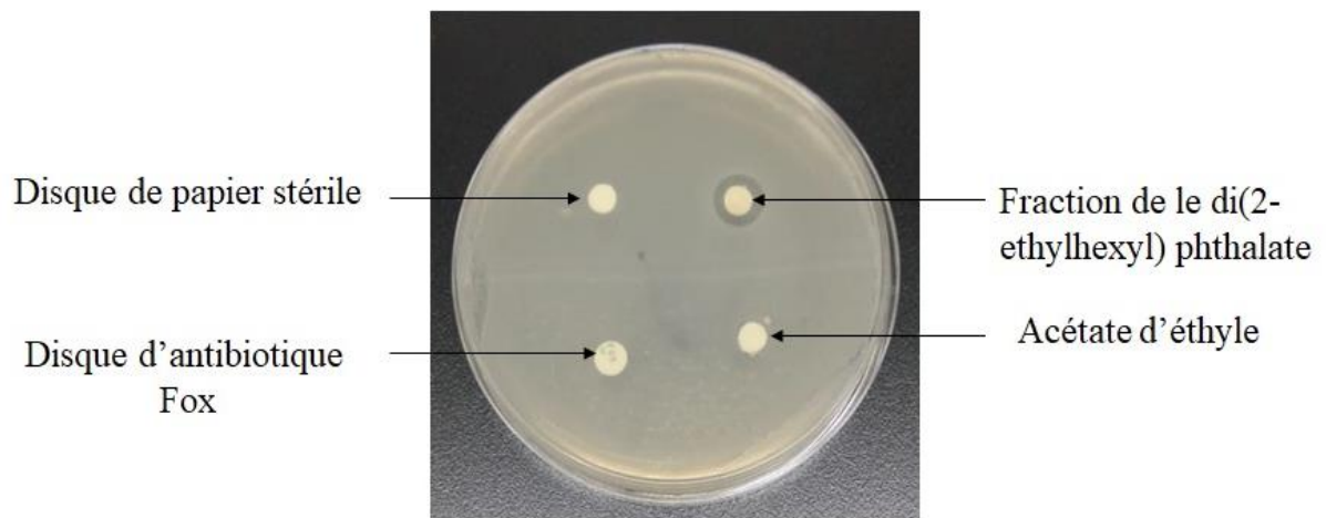
Figure 49. Activité antibactérienne de la fraction contenant le di(2-ethylhexyl) phthalate vis-à-vis SARM
