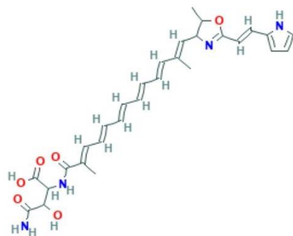
DKxanthene-534 C 29 H 34 N 4 O 6
