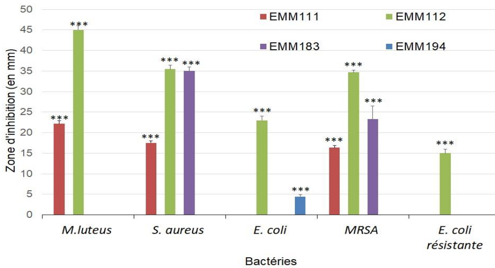
Figure 18. Action antibactérienne des 4 isolats d’actinobactéries vis-à-vis des 4 bactéries sur milieu Bennett. Chaque valeur représente la moyenne \pm écart-type de trois répétitions
