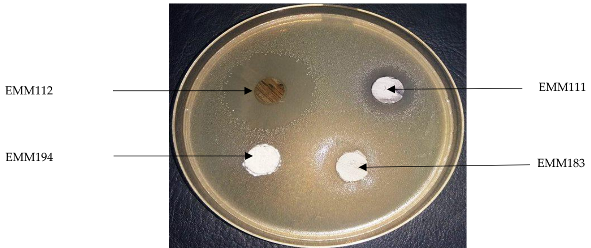
Figure 19. Mise en évidence de l’activité antibactérienne contre la souche S. aureus résistante à la Mécicilline (SARM)
