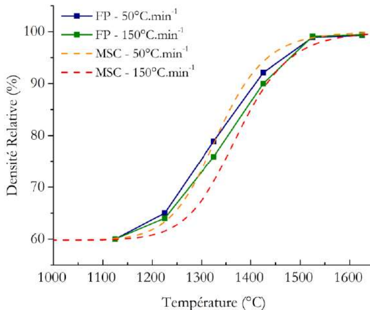
Figure 70 : Evolution de la densité relative des échantillons BSZ3Y traités en frittage pixélisé en fonction de la température maximale avec deux vitesses de montée ( 50 et 150^\circ\text{C.min}^{-1} ) et les courbes MSC correspondantes
