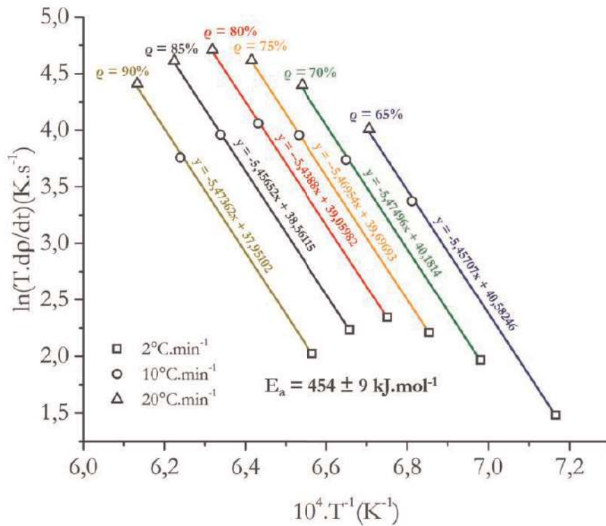
Figure 68 : Diagramme d'Arrhenius des vitesses de densification à différentes densités à partir des courbes dilatométriques obtenus avec trois rampes de montée en température pour la zircone yttrée à 3 %mol (BSZ3Y)
