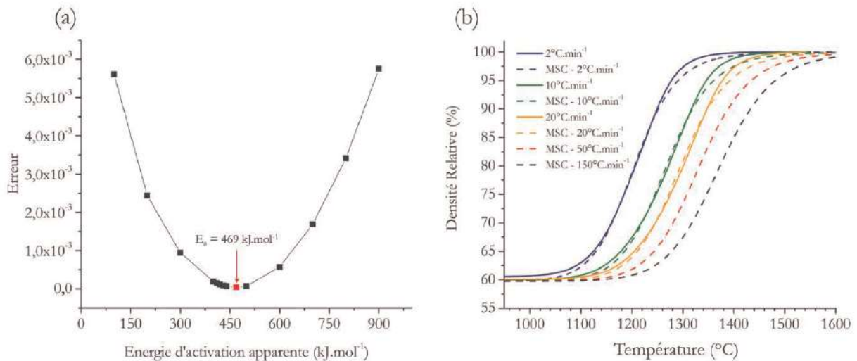
Figure 69 : (a) Erreur déterminée par la méthode des moindres carrés en fonction de l'énergie d'activation apparente et (b) Courbes de densification expérimentales et calculées avec la MSC obtenues pour la zircone BSZ3Y
