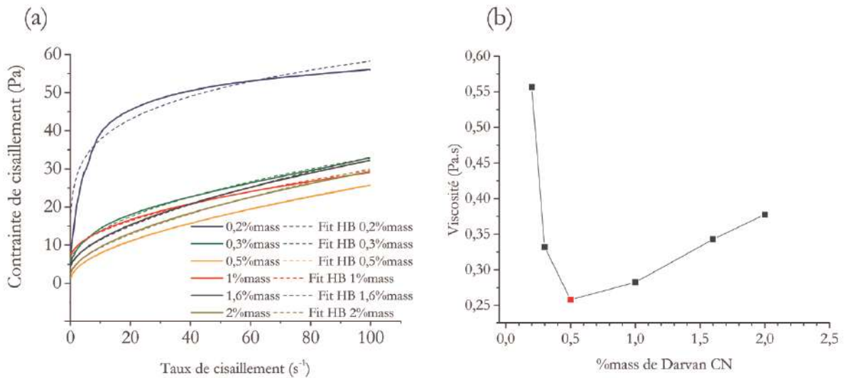
Figure 37 : (a) Contrainte en fonction du taux de cisaillement de suspensions d'alumine préparées avec différents taux de dispersant (b) Viscosité en fonction du taux de dispersant à 100\text{s}^{-1}
