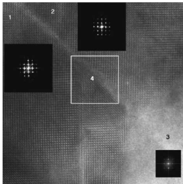
Figure 20 : Observation MET d'un joint de maclé dans une zircon 3Y-TZP pure. La phase monoclinique est en zone 1 et 2. La phase quadratique est en zone 3. La zone 4 est maclée [138].
