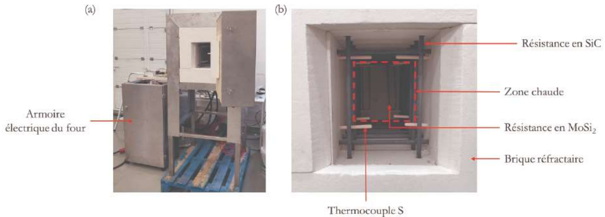
Figure 88 : Photos du four vue de (a) l'extérieur et (b) de l'intérieur
