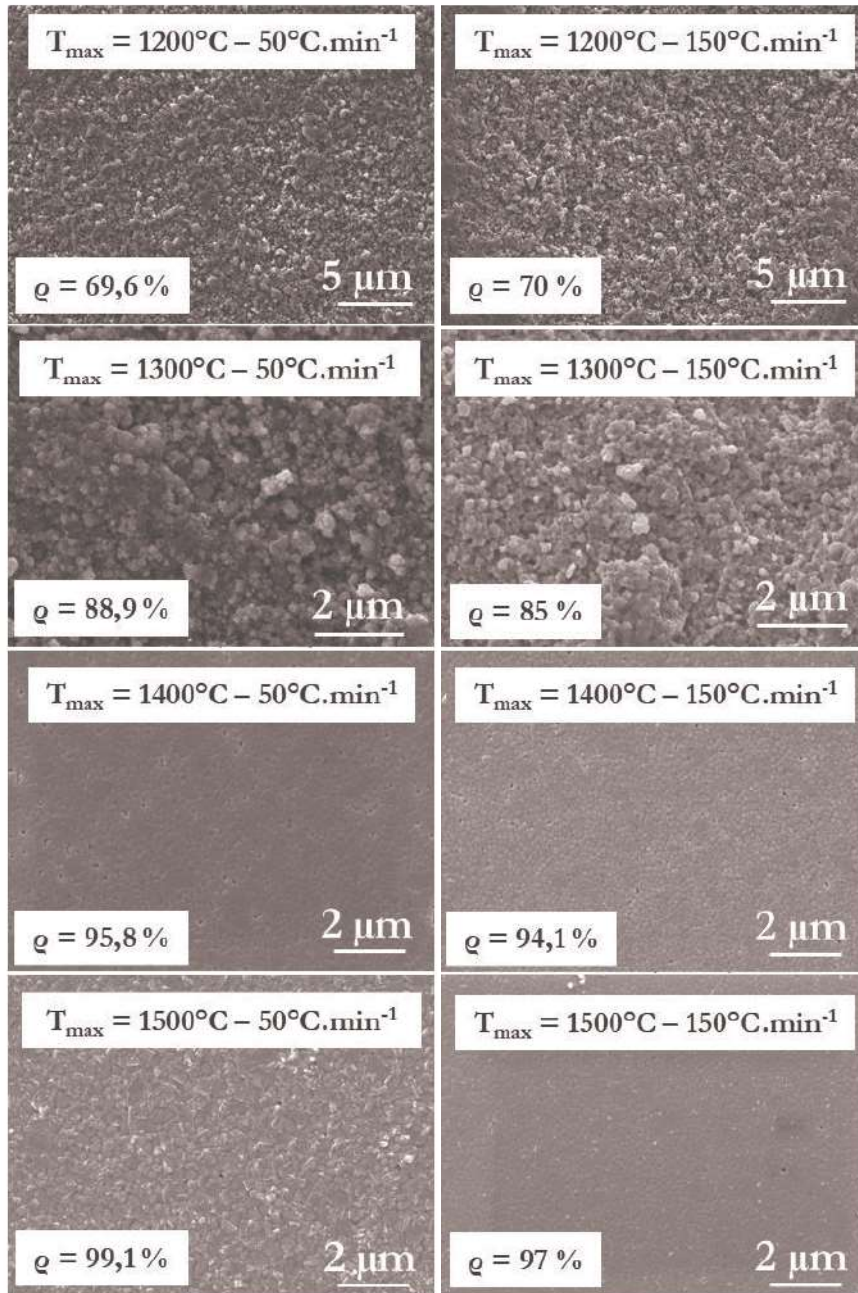
Figure 80 : Micrographies MEB des microstructures des échantillons de zircono BSZ3Y obtenus par frittage SPS-SP
