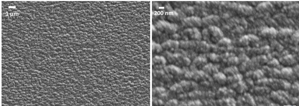
Figure III. 13 : Micrographies MEB d'un film de DNC déposé sur la structure AlN/ZnO/LiNbO 3 (S3)
