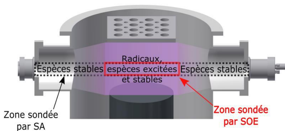
Figure V. 1 : Représentation simplifiée des zones de détection des radicaux et des espèces stables et excitées
