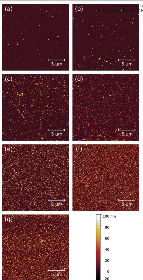
Fig. 2 AFM images with scale bar 20 \times 20 \mu m of the PBA NPs deposit on the amino-gold surface with different initial concentrations: (a) 0.04 mg \cdot mL^{-1} ; (b) 0.08 mg \cdot mL^{-1} ; (c) 0.16 mg \cdot mL^{-1} ; (d) 0.31 mg \cdot mL^{-1} ; (e) 0.62 mg \cdot mL^{-1} ; (f) 1.50 mg \cdot mL^{-1} ; (g) 2.50 mg \cdot mL^{-1} .
