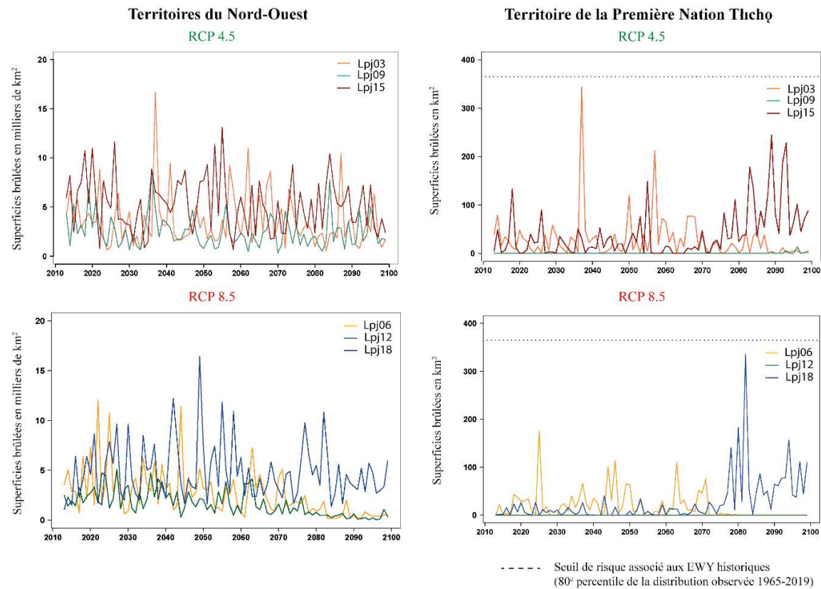
Figure 4.6. Superficies annuelles brûlées simulées entre 2013 et 2099 aux TNO et sur le territoire de la Première Nation Thchq, en fonction de divers modèles climatiques ( Annexe XXI ) et deux scénarios de forçage radiatif (RCP4.5 et RCP8.5). Le seuil associé aux EWY historiques (80 e percentile) sur le territoire Thchq est représenté en pointillés. Les projections de chaque modèle climatique sont représentées par une couleur différente.
