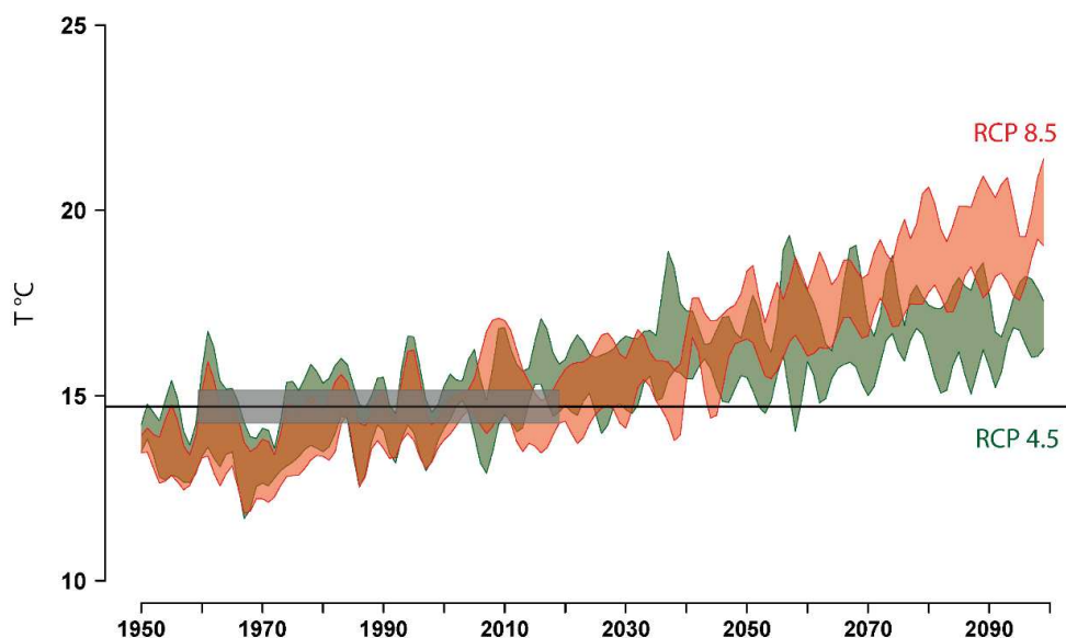
Figure 4.2. Moyenne des températures mensuelles maximales simulées pendant la saison de feu (mai à septembre), pour chaque année entre 1950 et 2099, sur le territoire de la Première Nation Tłıchǰ. Les enveloppes en vert (RCP4.5) et en rouge (RCP8.5) indiquent l'intervalle de confiance bootstrap à 90 % des valeurs des multi-modèles (CanESM2, EC-EARTH, CanRCM4 et RCA4; Annexe XXI ) pour deux scénarios RCP. La période ombragée en gris (1965-2019) correspond aux observations climatologiques historiques à partir desquelles le seuil de température associé à des EWY (14,7 °C), défini au chapitre II , a été calculé (ligne horizontale noire).
