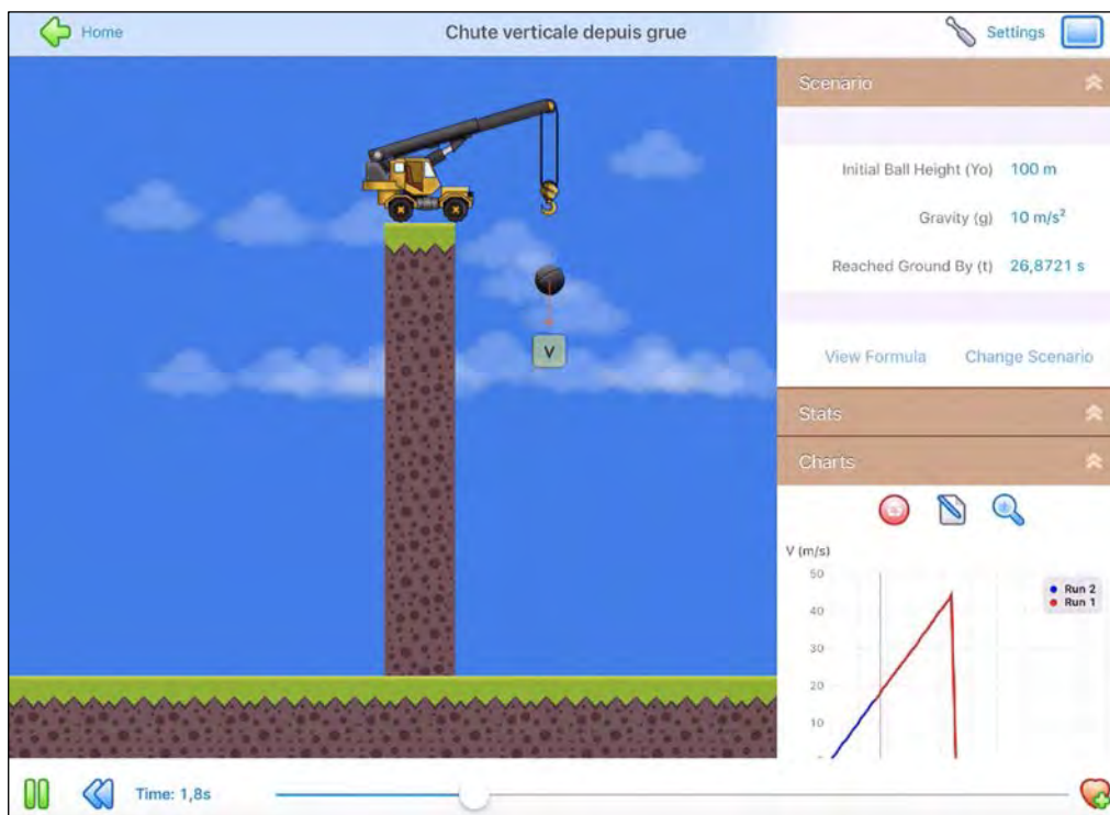
Figure 27 : simulateur de chute verticale.
