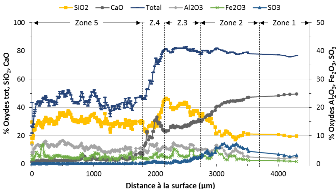
Figure V - 12 : Profils de composition chimique en fonction de la distance à la surface (analyses EPMA) de la pâte de CEM I immergée dans la solution AA+BS+NA (0,30 mol.L -1 d'acide acétique, 0,2429 mol.L -1 de bicarbonate de sodium et 0,0444 mol.L -1 de nitrate d'ammonium) pendant 18 semaines
