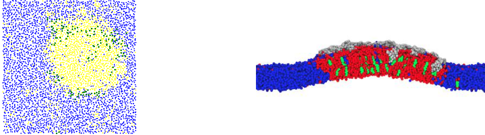
FIGURE 18 – Simulation d'une bicouche de 43 nm de côté constituée d'un mélange DPPC-DIPC-chol (30 :58 :12) et 5% de GM1 dans le feuillet supérieur. Gauche : Répartition spatiale des espèces, vue de dessus de la dernière étape. DPPC (Lo) en jaune, DIPC (Ld) en bleu et GM1 en vert. Droite : Image de la dernière étape de simulation. DPPC (Lo) en rouge, DIPC (Ld) en bleu, cholestérol en vert et GM1 en argenté. On peut remarquer la localisation préférentielle de GM1 dans la phase Lo et l'importante courbure locale de la membrane. La visualisation est produite en utilisant VMD.
