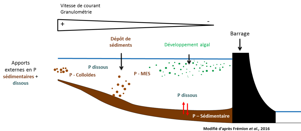
Figure 1: Apports externes et internes du P en retenue de barrage.
