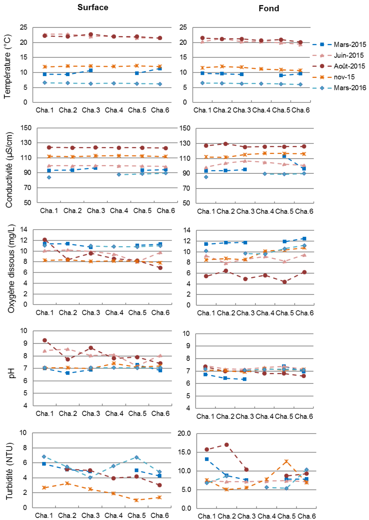
Figure 60 : Evolution des paramètres physico-chimiques dans les eaux de surface et de fond de la retenue de Champsanglard de mars 2015 à mars 2016.
