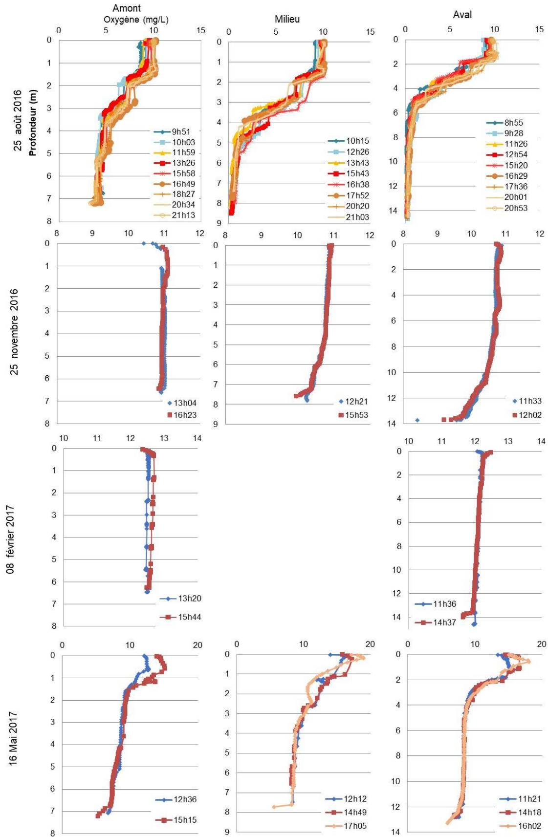
Figure 56 : Variations des teneurs en oxygène dissous (mg/L) le long de la colonne d'eau, pour les différentes stations de mesure dans la retenue de Champsanglard et à différentes saisons.
