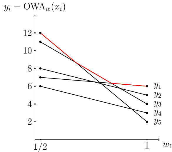
FIGURE 2.1 – Images \text{OWA}_w(x^i) de x^i \in \mathcal{X} et \bigcup_{w \in W} \max_{x^i \in \mathcal{X}} \text{OWA}_w(x^i) (en rouge).
