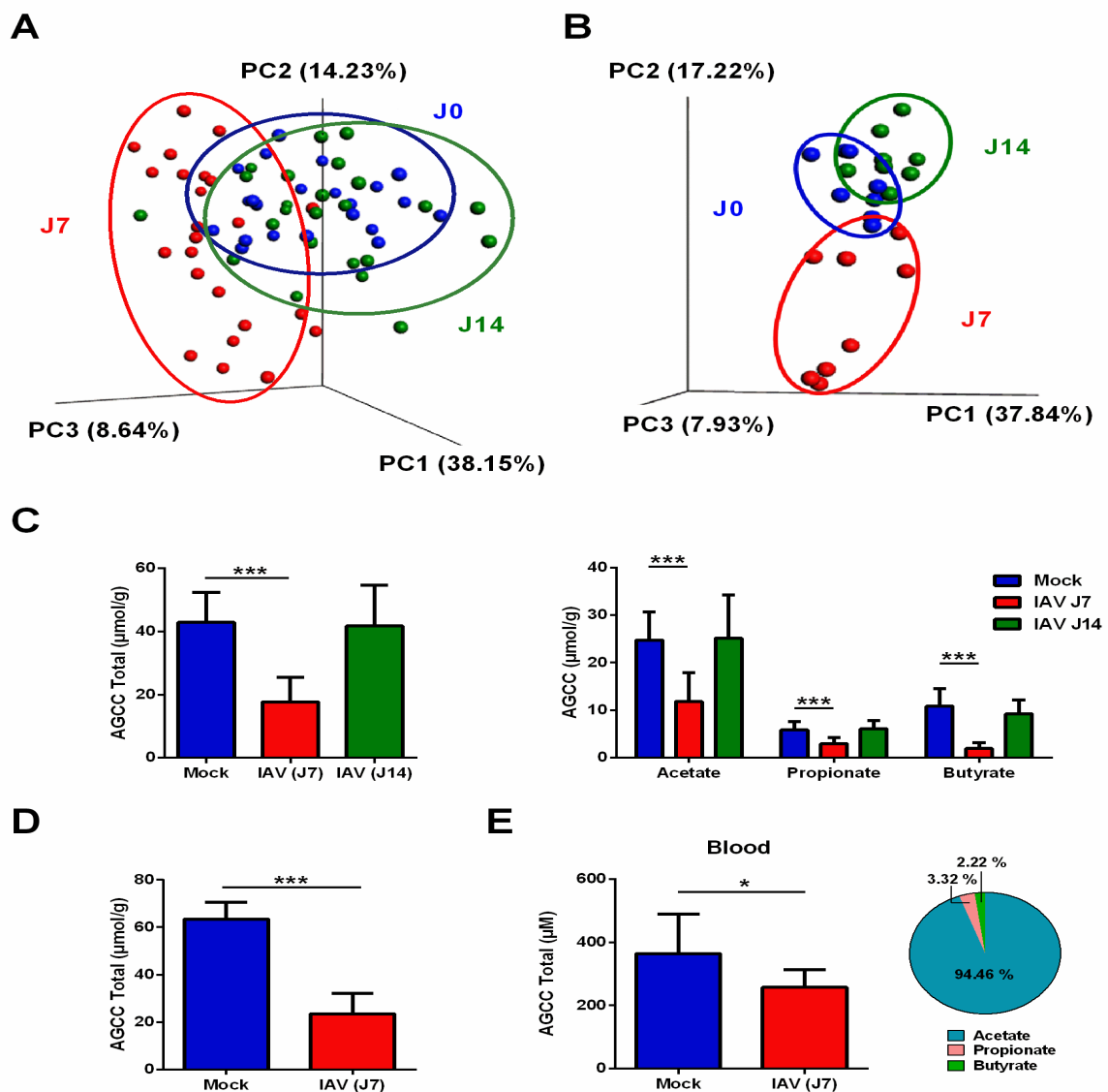
Figure 11. Altération de la composition et de l'activité fermentative (production d'AGCC) du microbiote intestinal au cours de l'infection par l'IAV. (A) Sept et quatorze jours après l'infection par
