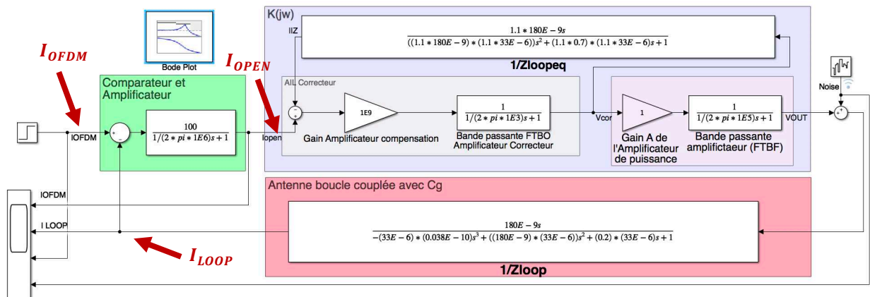
Figure 4-15. Schéma de simulation du circuit émetteur asservi en courant par compensation de pôles.
