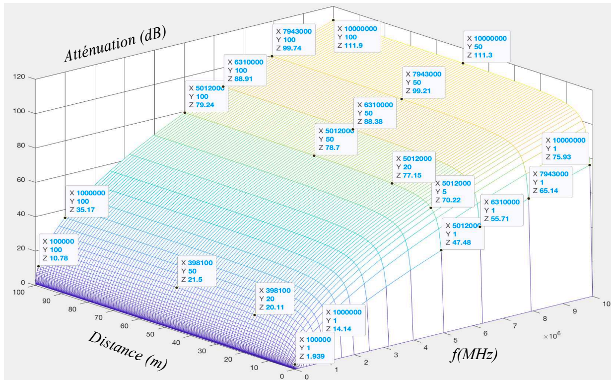
Figure 3-15. Atténuation linéique de puissance d'après le modèle de comportement de C.Urbe et W.Grote [169]
