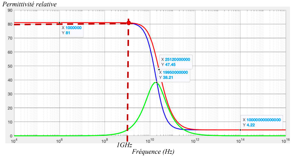
Figure 3-4. Module \left| \frac{\varepsilon}{\varepsilon_0} \right| (rouge), partie réelle \frac{\varepsilon'}{\varepsilon_0} (en bleu), partie imaginaire \frac{\varepsilon''}{\varepsilon_0} (en vert) de la permittivité relative du modèle retenu en fonction de la fréquence (Hz) avec \varepsilon_\infty = 4,22 et \varepsilon_s = 81
