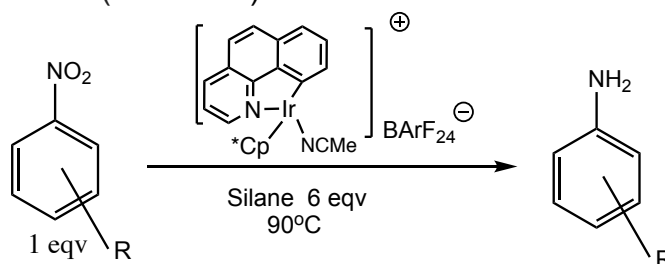
Schéma 5: Iridacycle cationique 1b effectuer la réduction nitro
