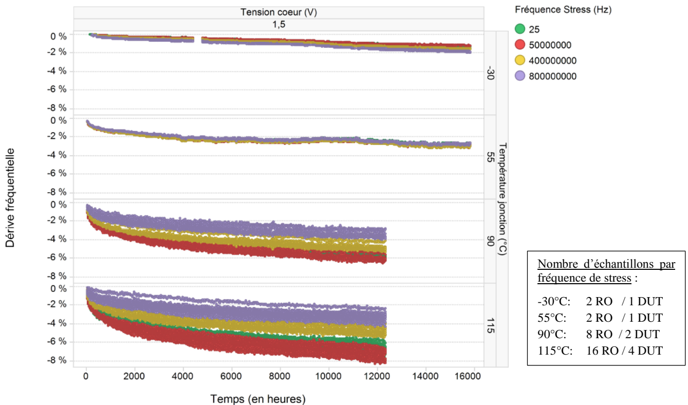
Figure 102 : Dérives fréquentielles en fonction de la température et de la fréquence de stress pour tous les RO à V_{nom}+50\%
