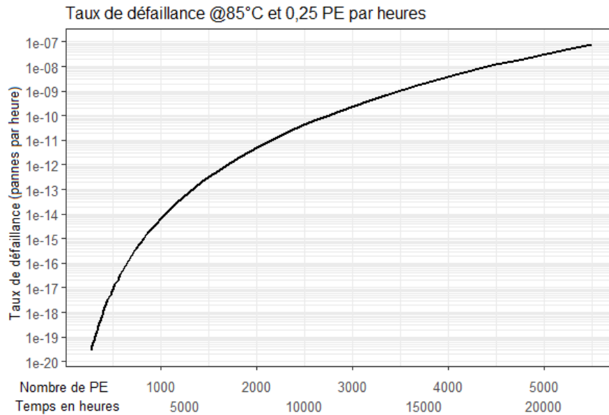
Figure 72 : Taux de défaillance à 85°C, NAND endurance
