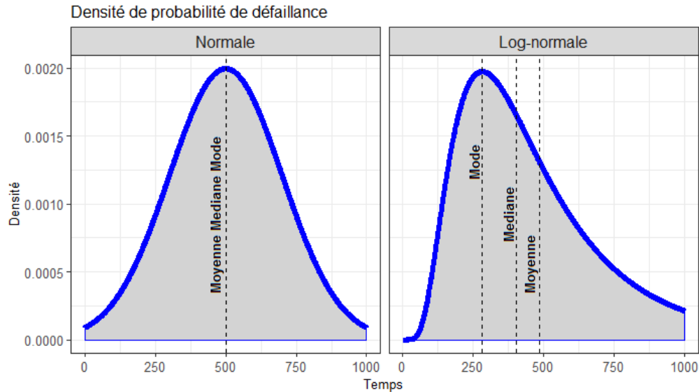
Figure 7 : Comparaison d'une distribution normale et d'une distribution log-normale
