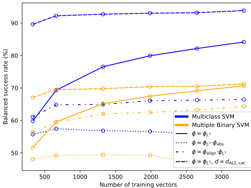
Figure 6.4-10 – Taux de succès de classification \rho des vecteurs de \mathbb{V}'_{\text{close}} en fonction du nombre de vecteurs d'entraînement, pour un classificateur multi-classes et une combinaison de classificateurs binaires, avec divers prétraitements \varphi et métriques d utilisés avec un noyau gaussien.
