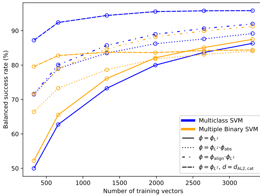
Figure 6.4-9 – Taux de succès de classification \rho des vecteurs de \mathbb{V}'_{\text{known}} en fonction du nombre de vecteurs d'entraînement, pour un classificateur multi-classes et une combinaison de classificateurs binaires, avec divers prétraitements \varphi et métriques d utilisés avec un noyau gaussien.
