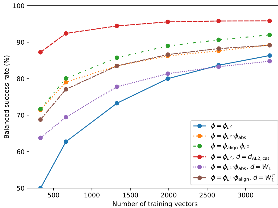
Figure 6.4-5 – Taux de succès de classification \rho des vecteurs de \mathbb{V}'_{\text{known}} en fonction du nombre de vecteurs d'entraînement, pour un classificateur multi-classes avec divers prétraitements \varphi et métriques d utilisés avec un noyau gaussien. d(a, b) = \|a - b\|_2 sauf mention contraire.
