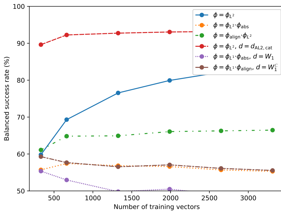
Figure 6.4-6 – Taux de succès de classification \rho des vecteurs de \mathbb{V}'_{\text{close}} en fonction du nombre de vecteurs d'entraînement, pour un classificateur multi-classes avec divers prétraitements \varphi et métriques d utilisés avec un noyau gaussien. d(a, b) = \|a - b\|_2 sauf mention contraire.
