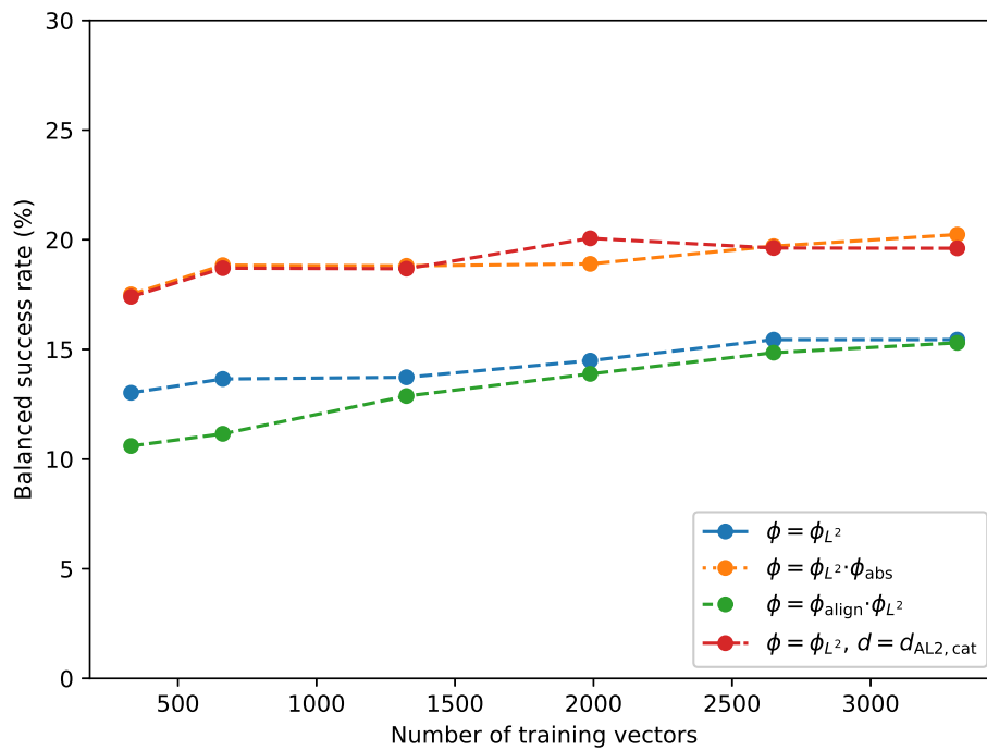
Figure 6.4-4 – Taux de succès de classification \rho des vecteurs de \mathbb{V}_{\text{unknown}} en fonction du nombre de vecteurs d'entraînement, pour un classificateur multi-classes avec divers prétraitements \varphi et métriques d utilisés avec un noyau gaussien. d(a, b) = \|a - b\|_2 sauf mention contraire.
