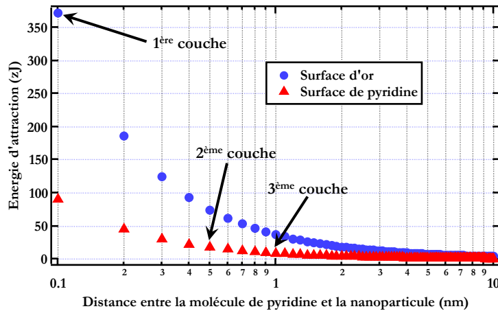
FIGURE 3.11 – Energies d'attraction W(d) calculées à partir de l'équation 3.8. L'attraction sur la surface d'or est calculée avec une constante de Hamaker A = 455 zJ. L'attraction sur une surface de pyridine est calculé avec A = 110 zJ.
