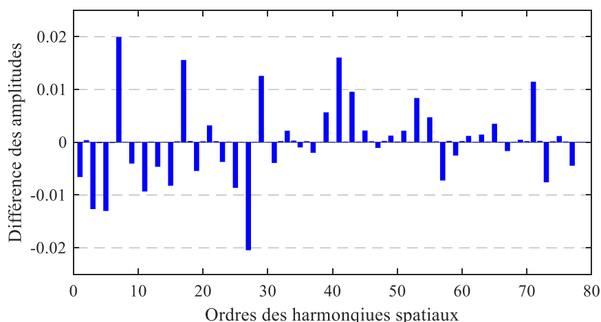
Figure III-29 : Différence entre les deux approches sur l'amplitude des harmoniques spatiaux de l'induction totale dans l'entrefer
