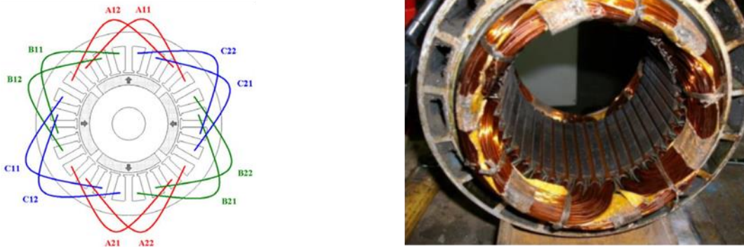
Figure I-2 : Bobinage distribué triphasé [7]
