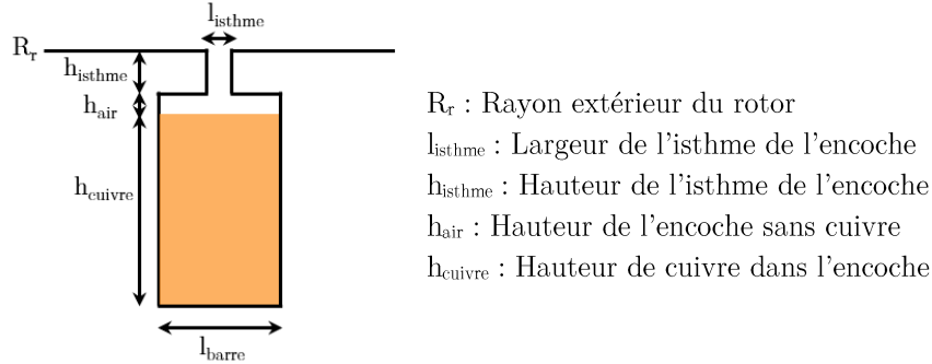
Figure III-24 : Paramétrisation d'une encoche rotorique
