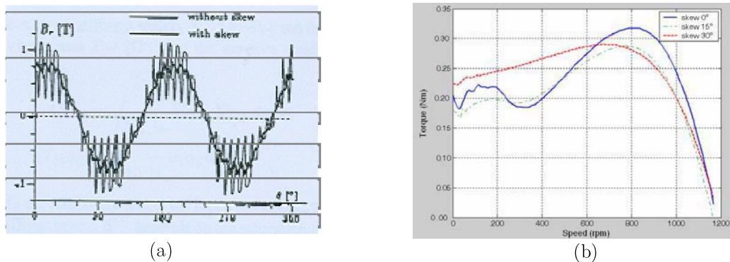
Figure I-28 : Effet du vrillage du rotor, (a) sur l'induction dans l'entrefer, (b) sur la caractéristique couple en fonction de la vitesse [50].
