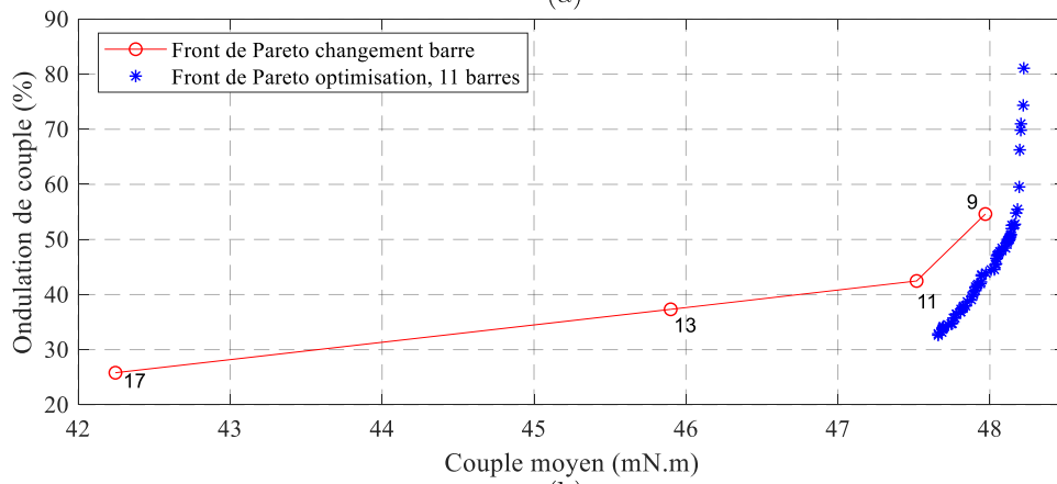
Figure V-6 : Résultats de l'optimisation de la MAS 6s4p11barres bobinage classique, (a) comparaison du front de Pareto avec la solution à 11 barres équidistantes, (b) comparaison avec le front de Pareto obtenu avec le changement du nombre de barres au rotor
