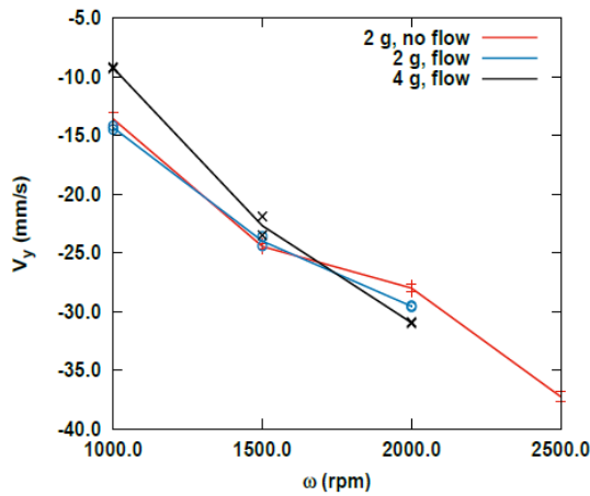
(b) Q_1(V_y)
