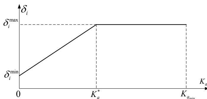
Figure III.18 – Règle de l'amplitude du signal d'excitation
