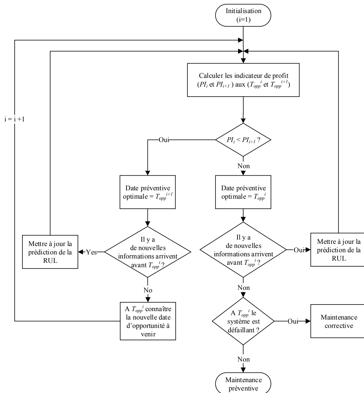
Figure IV.5 – Processus de décision de la stratégie de maintenance prédictive
