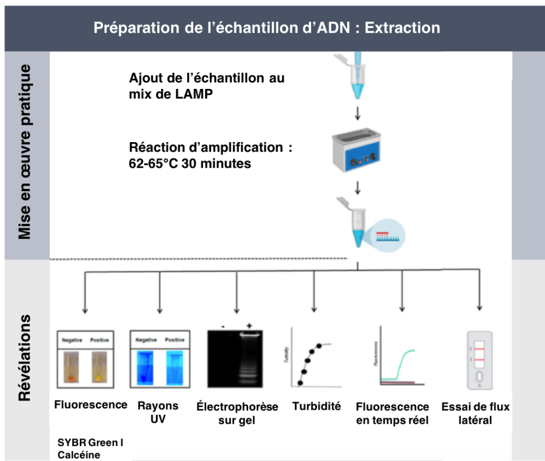
FIGURE 2.4 – Mise en œuvre de la LAMP et systèmes de révélation. Figure adaptée de Silva et al. , (2020) (Silva et al. , 2019).
