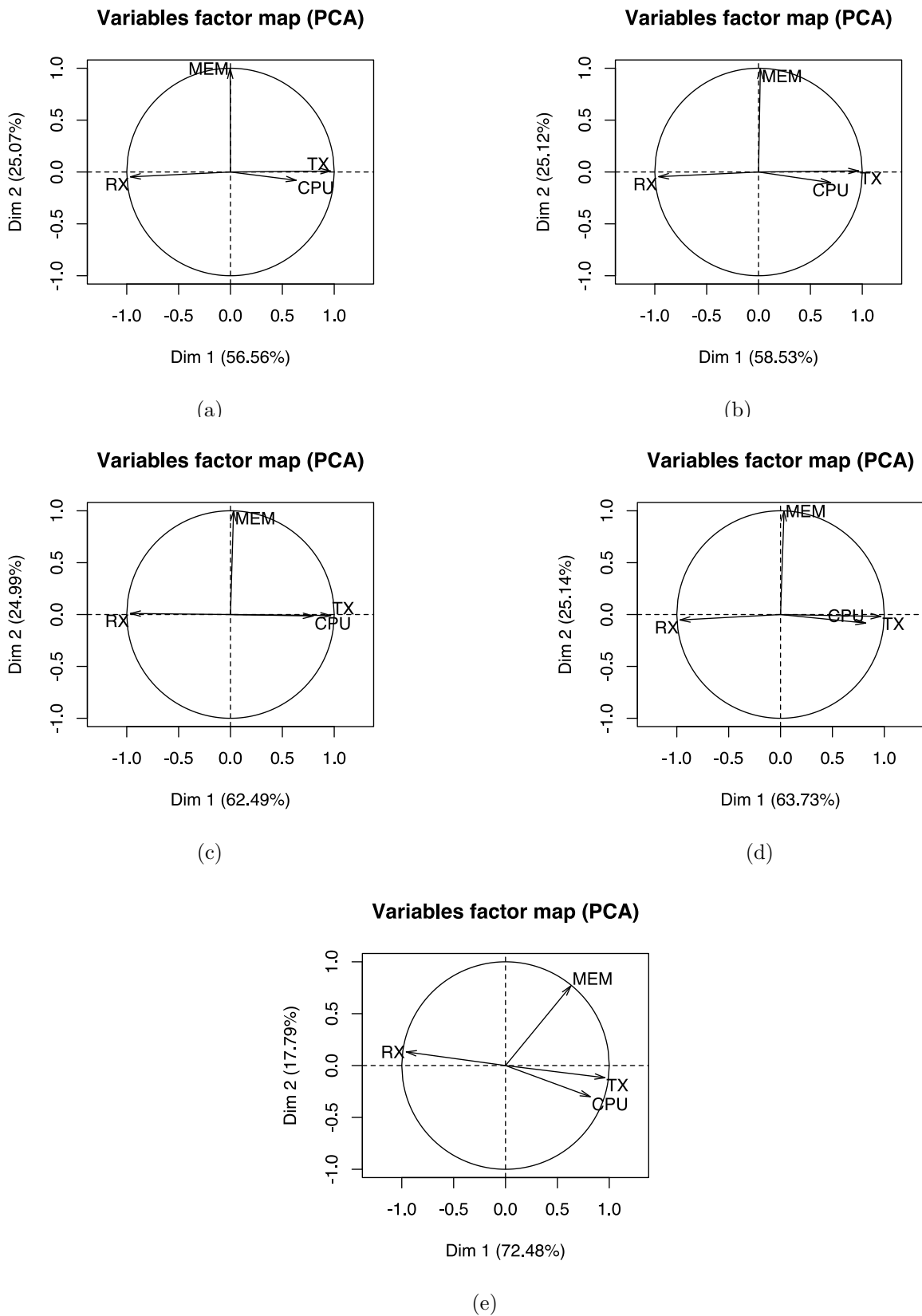
FIGURE A.4 – Cercles de corrélations des ACP réalisées sur le botnetHybrid_V1.0 réalisant des attaques UDP Flood : (a) 8 Mb/s; (b) 16 Mb/s; (c) 40 Mb/s; (d) 56 Mb/s; (e) 80 Mb/s
