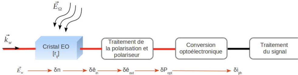
FIGURE 1.2.1 – Principe de la sonde EO : Cascade de conversions des grandeurs physiques mises en jeu. n est l'indice de réfraction du cristal, \hat{e} correspond à l'état de polarisation de l'onde optique, P_{opt} est la puissance optique et I_{ph} représente le photo-courant produit par la photodiode. Extraite de [Jarrige 13].
