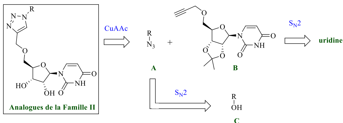
Schéma 11 : Rétrosynthèse envisagée pour les analogues de la Famille II
