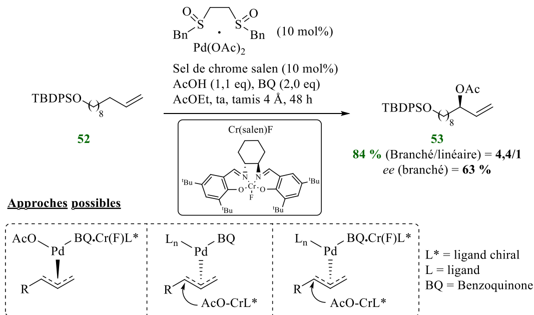
Schéma 21 : Oxydation asymétrique intermoléculaire par activation C-H allylique
