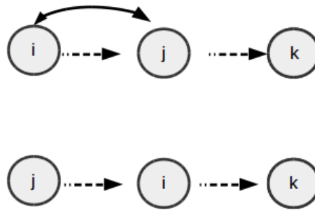
FIGURE 4.2 – Exemple du mouvement S\_Exchange
