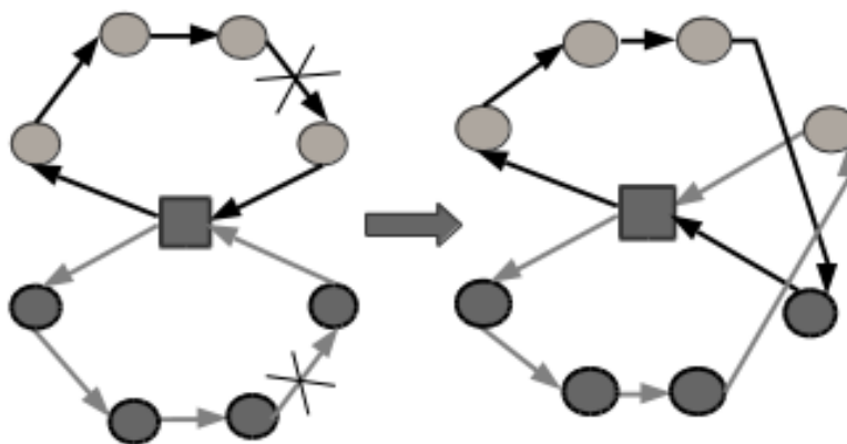
FIGURE 4.5 – Exemple du mouvement 2Opt^*
