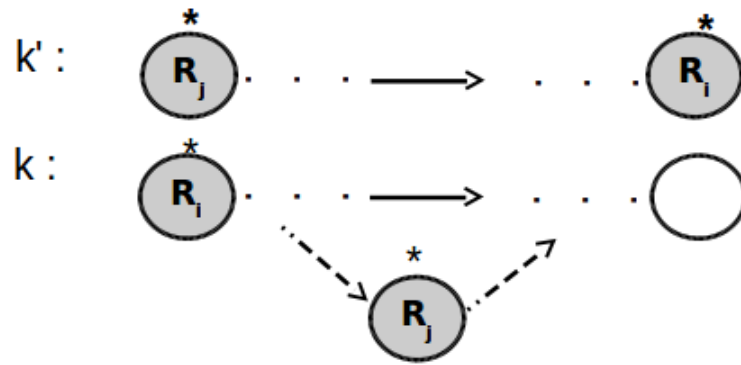
FIGURE 4.8 – Exemple d’une insertion après un client synchronisé
