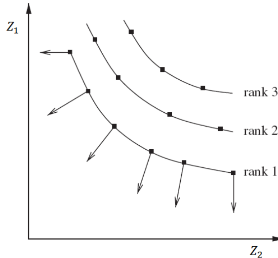
FIGURE 6.4 – Exemple de direction de descente de LS2
