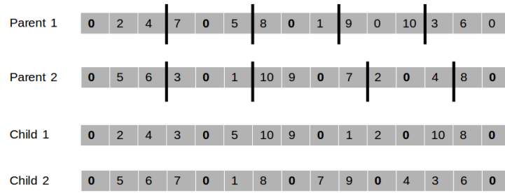
FIGURE 6.3 – Exemple de croisement
