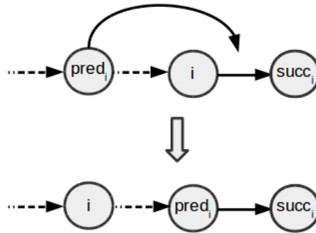
FIGURE 4.1 – Exemple du mouvement S\_Relocate
