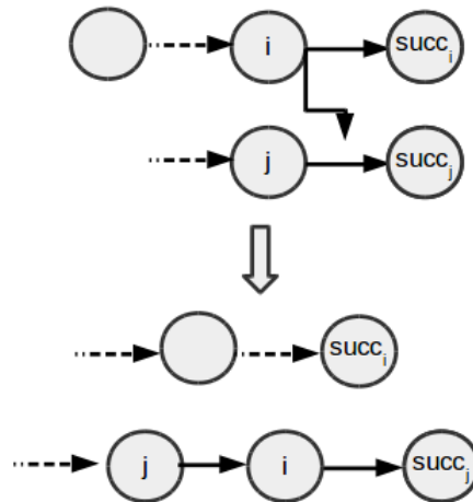
FIGURE 4.3 – Exemple du mouvement M\_Relocate
