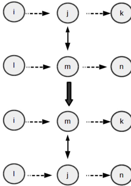
FIGURE 4.4 – Exemple du mouvement M\_Exchange
