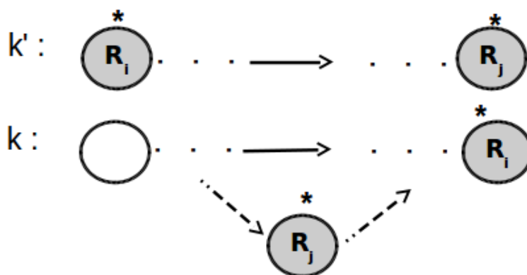
FIGURE 4.7 – Exemple d’une insertion avant le premier client synchronisé
