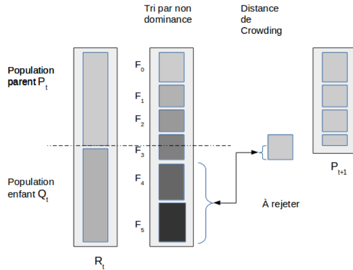
FIGURE 6.1 – Mise à jour de la population
