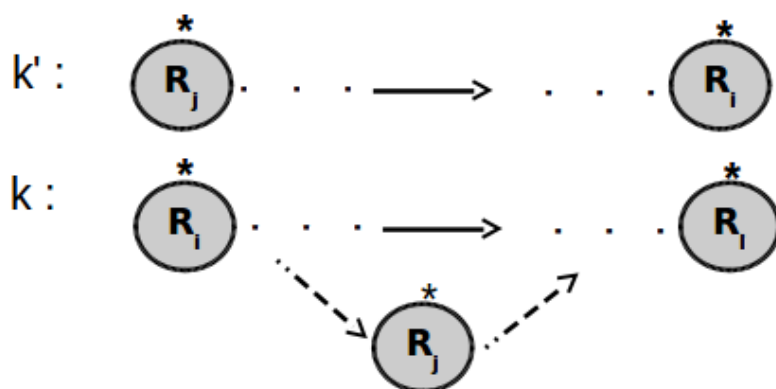
FIGURE 4.6 – Exemple d’une insertion entre deux clients synchronisés
